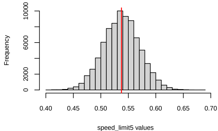
Posterior histogram of speed_limit5
