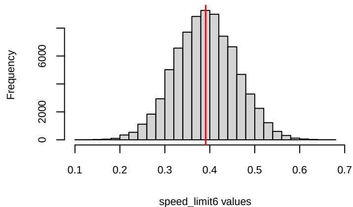
Posterior histogram of speed_limit6
