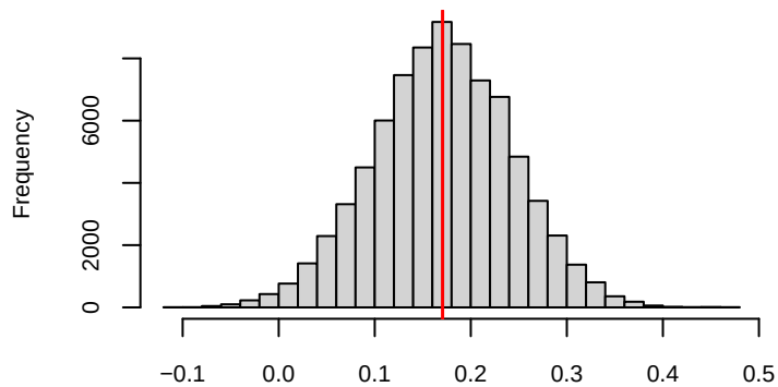
Posterior histogram of speed_limit1
