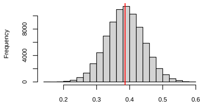
Posterior histogram of speed_limit4
