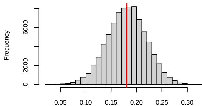
Posterior histogram of speed_limit3
