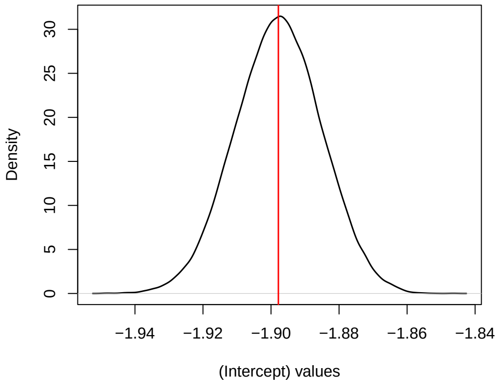
CMC posterior density of (Intercept)
