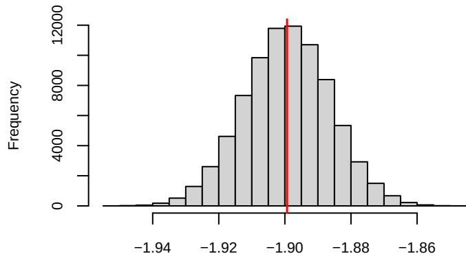
Posterior histogram of (Intercept)
