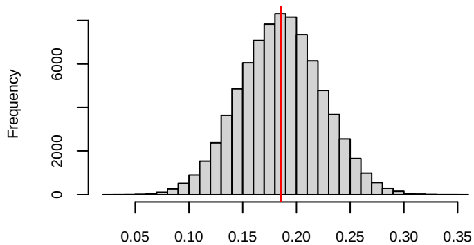
Posterior histogram of speed_limit3
