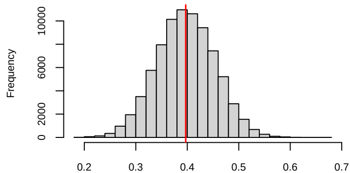
Posterior histogram of speed_limit4
