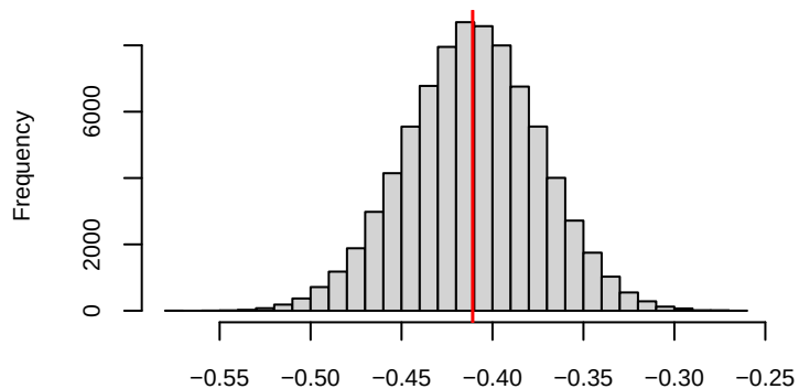
Posterior histogram of road_typeroundabout
