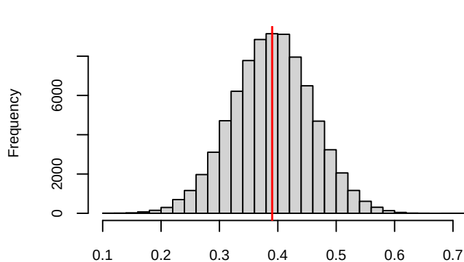
Posterior histogram of speed_limit6
