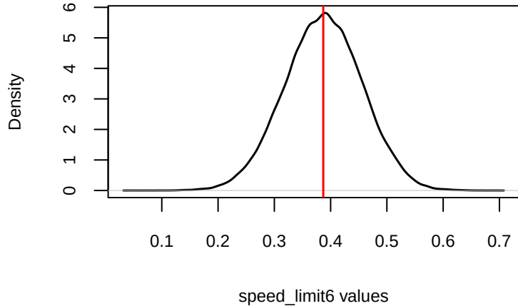
CMC posterior density of speed_limit6
