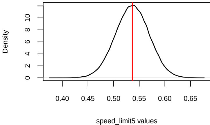
CMC posterior density of speed_limit5
