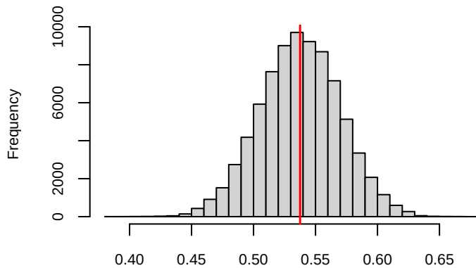
Posterior histogram of speed_limit5
