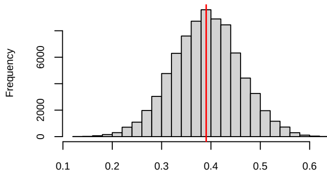
Posterior histogram of speed_limit6
