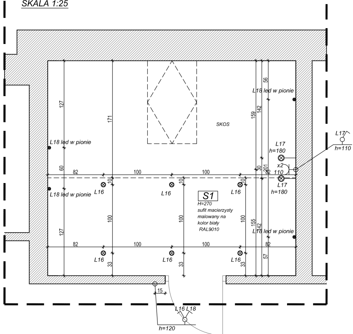
ŁAZIENKA PIĘTRO RZUT SUFITU I ELEKTRYKI SKALA 1:25
