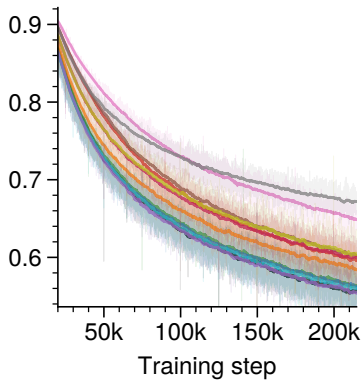
CLS MSE
