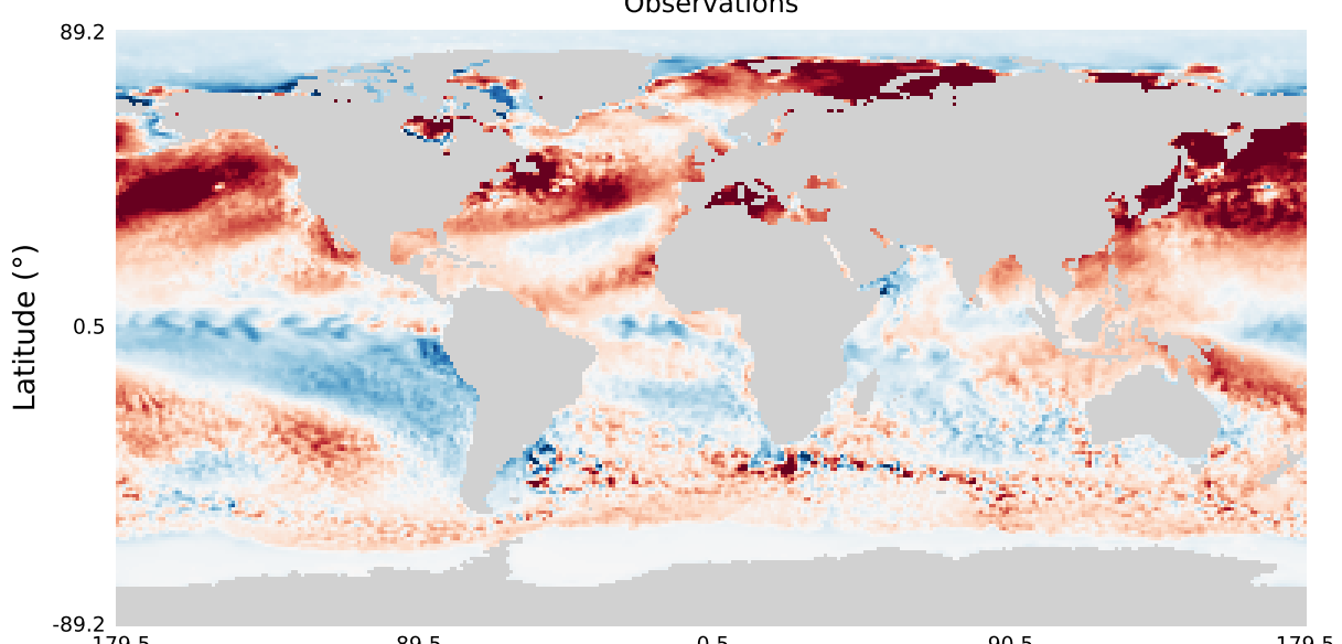
U-global
