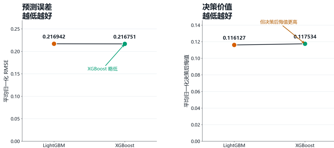
图 1 | 预测指标不能单独决定储能决策价值。图中比较八建筑测试集等权聚合结果。XGBoost 的归一化 RMSE 略低，但归一化决策后悔值略高，表明两类指标在该实验范围内可能给出不同排序。
