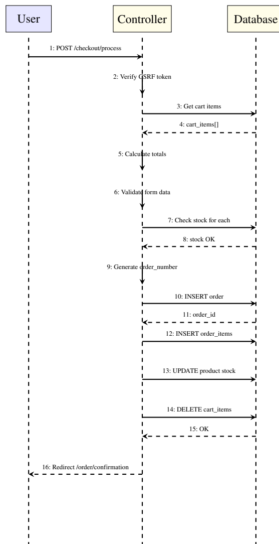
Hình 7.4: Sequence Diagram - Đặt hàng
