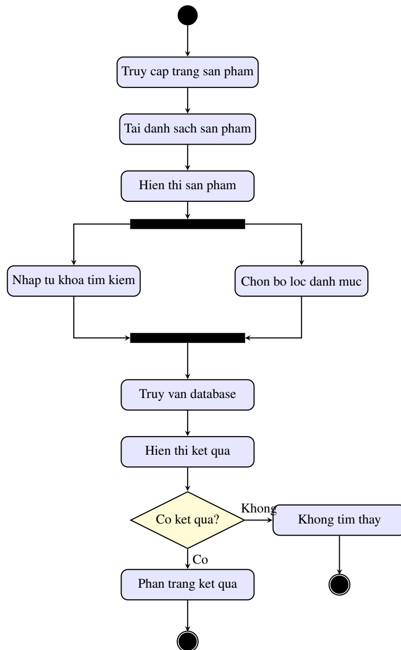
Hình 8.3: Activity Diagram - Tìm kiếm và lọc sản phẩm
