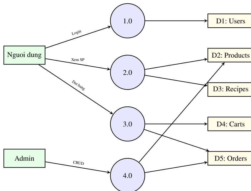
Hình 4.6: Data Flow Diagram Level 1
