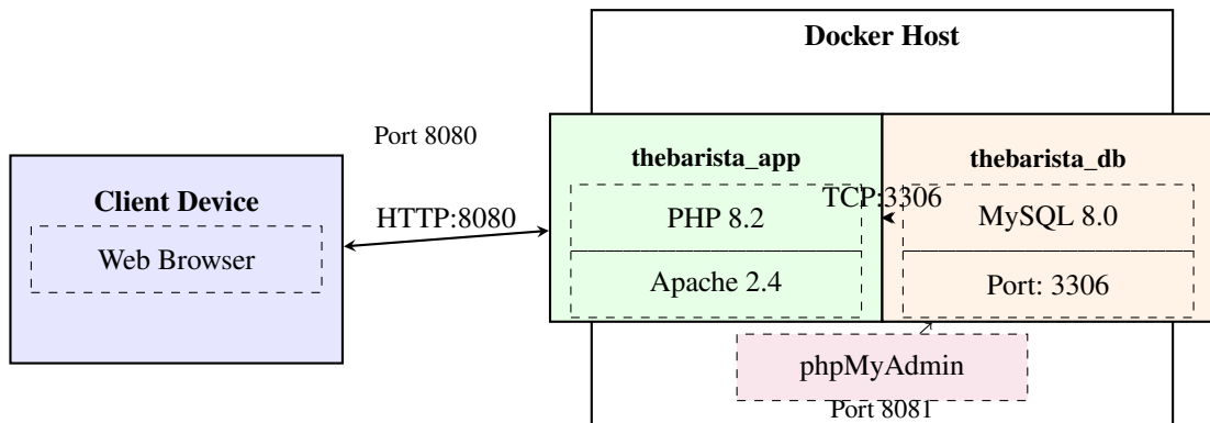
Hình 4.3: Deployment Diagram với Docker
