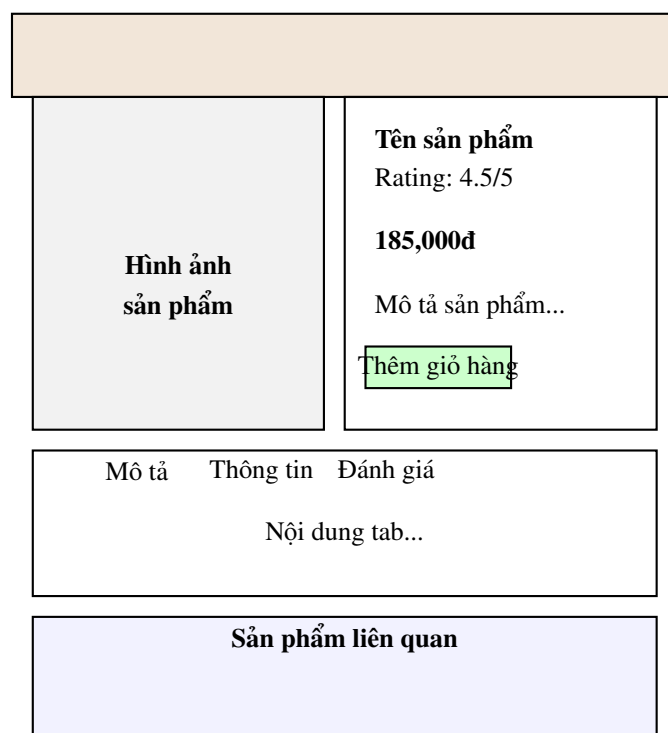
Hình 9.4: Layout chi tiết sản phẩm
