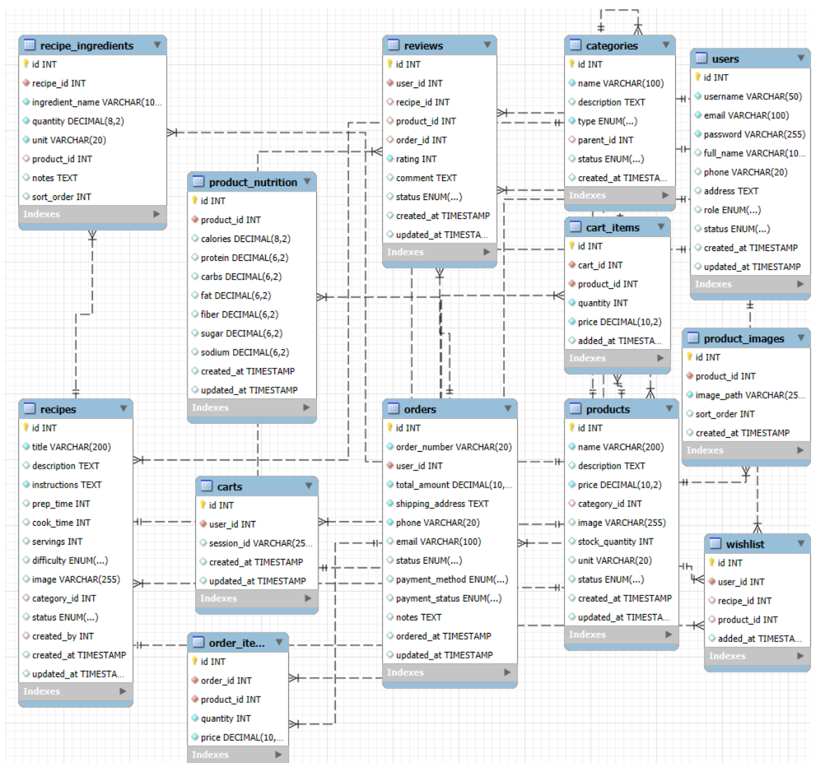
Hình 5.1: Entity Relationship Diagram của hệ thống TheBarista
