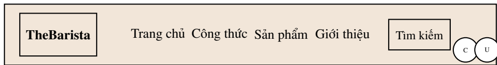
Hình 9.1: Layout Header
