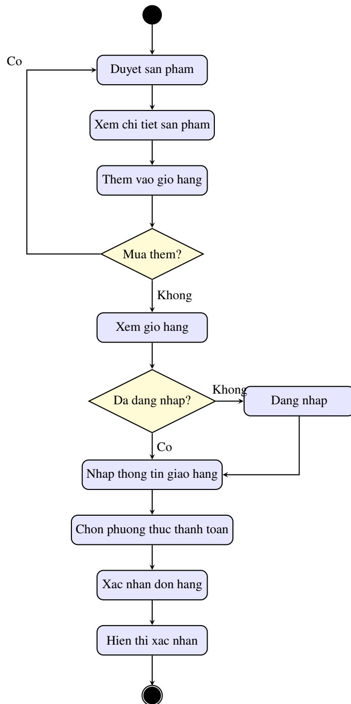
Hình 8.1: Activity Diagram - Quy trình đặt hàng
