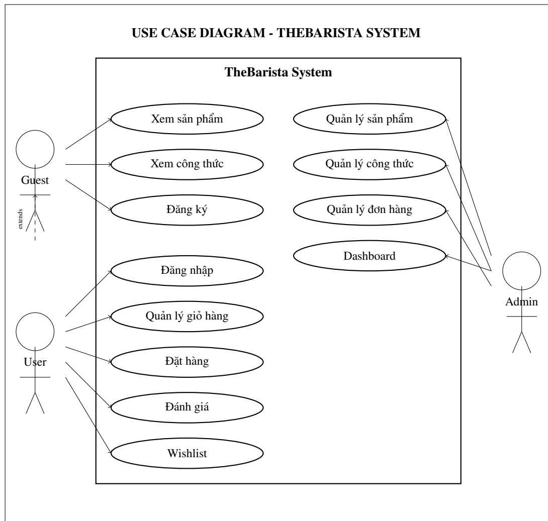
Hình 3.1: Biểu đồ Use Case tổng quan của hệ thống TheBarista
