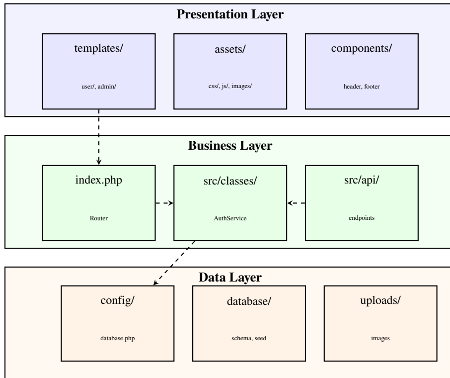
Hình 4.7: Package Diagram - Cấu trúc module hệ thống
