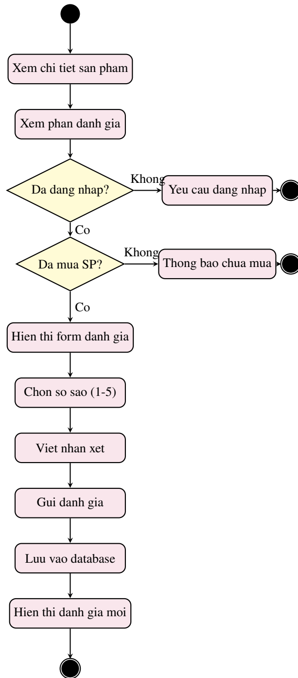
Hình 8.4: Activity Diagram - Đánh giá sản phẩm
