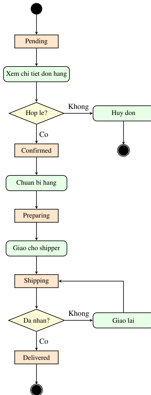
Hình 8.2: Activity Diagram - Quy trình xử lý đơn hàng
