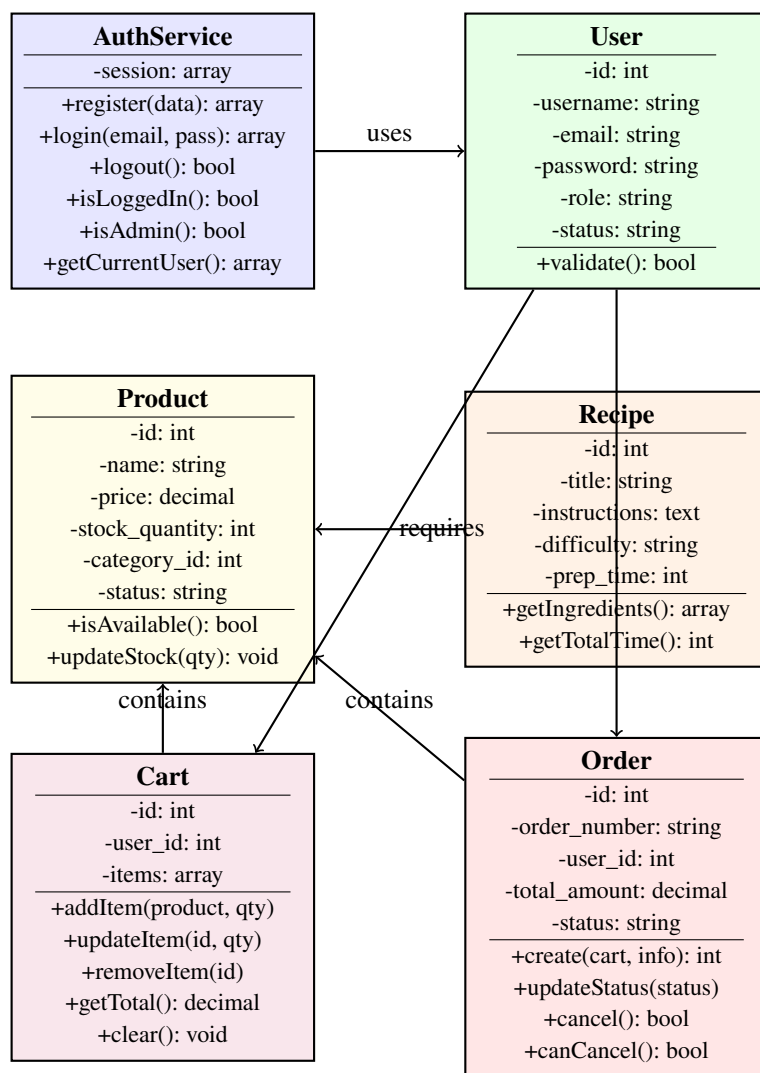
Hình 6.1: Class Diagram tổng quan của hệ thống
