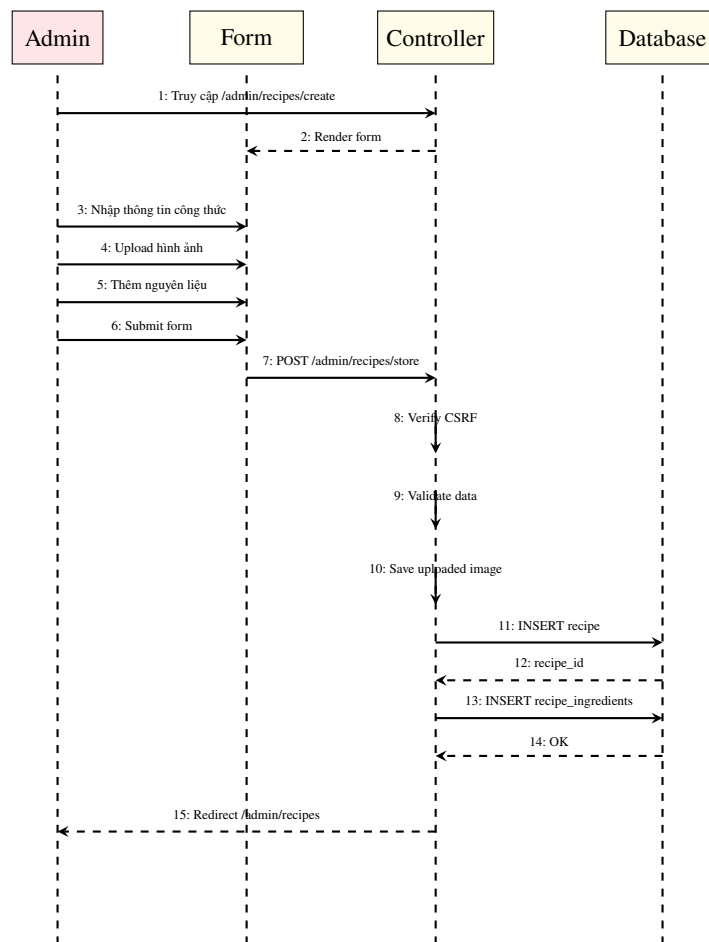
Hình 7.6: Sequence Diagram - Admin tạo công thức
