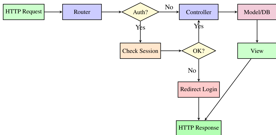
Hình 4.4: Luồng xử lý Request trong hệ thống
