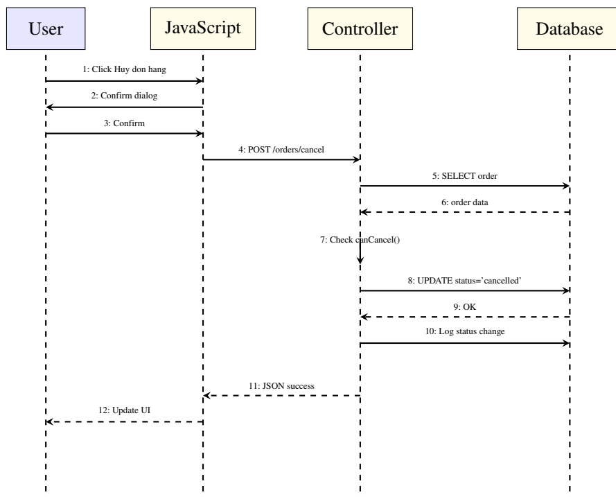
Hình 7.5: Sequence Diagram - Hủy đơn hàng
