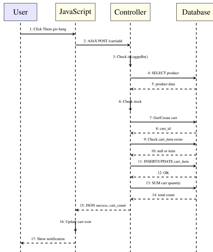
Hình 7.3: Sequence Diagram - Thêm vào giỏ hàng
