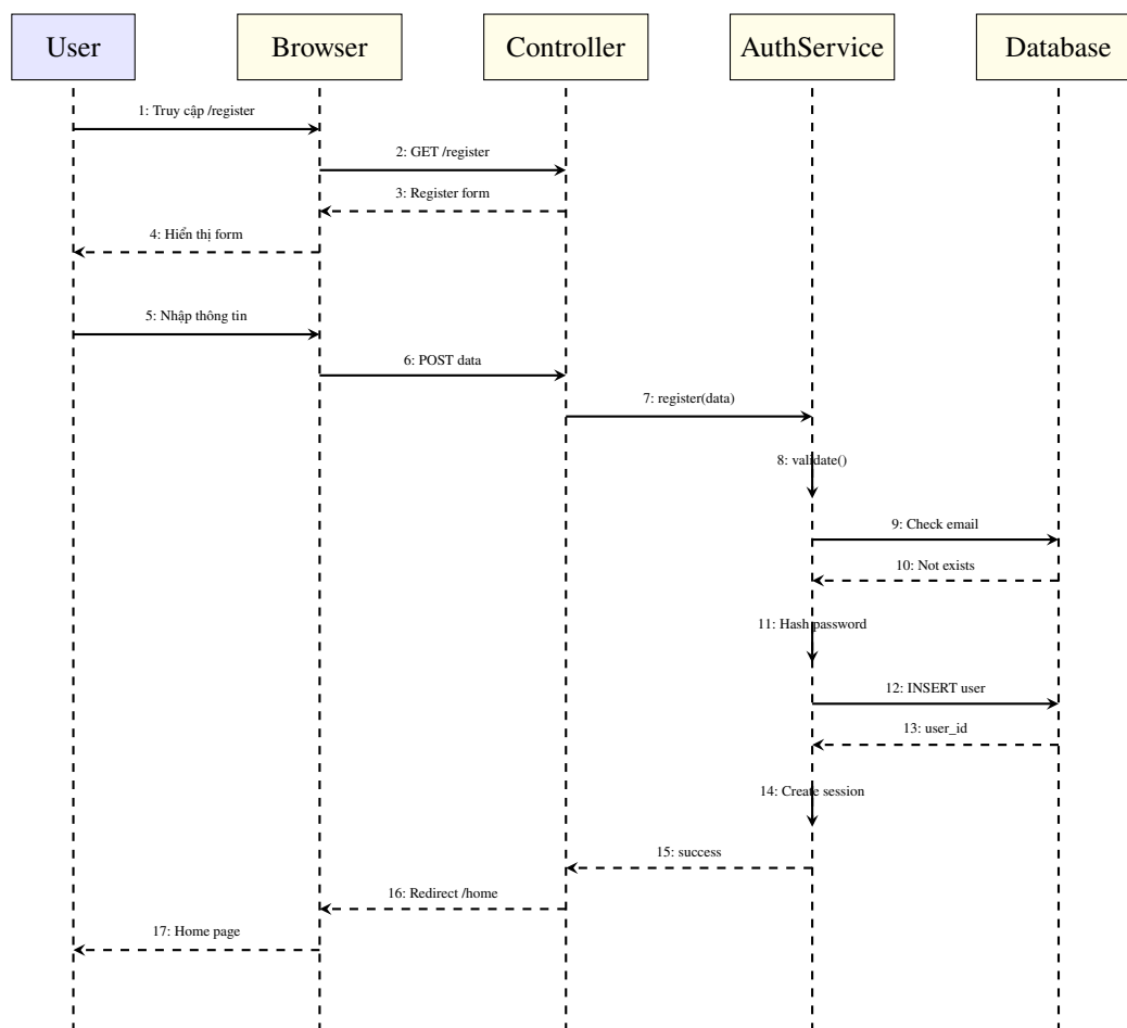
Hình 7.1: Sequence Diagram - Đăng ký tài khoản
