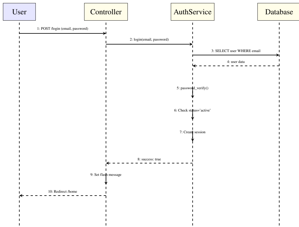
Hình 7.2: Sequence Diagram - Đăng nhập
