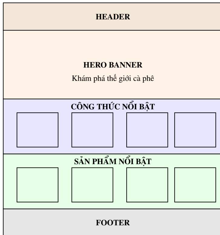
Hình 9.2: Layout Homepage
