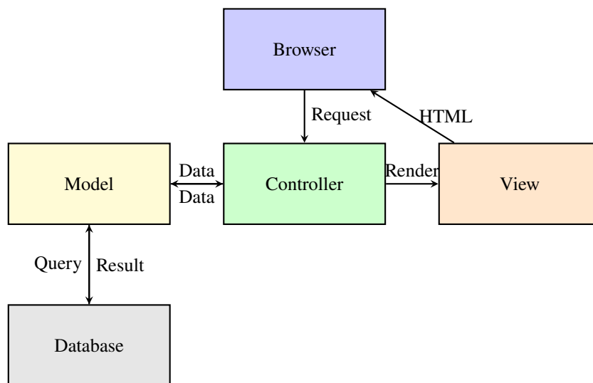
Hình 4.1: Mô hình MVC của hệ thống TheBarista
