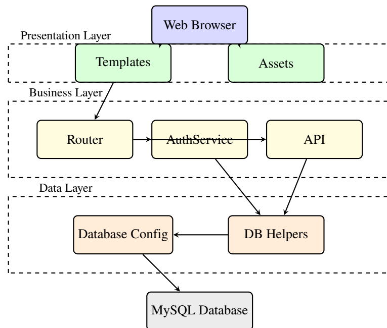
Hình 4.2: Component Diagram của hệ thống
