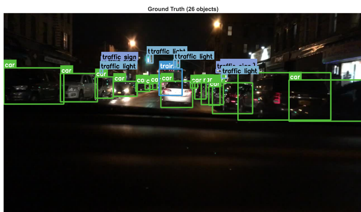
Sample #6: ceaa4904-2fec7d06.jpg
