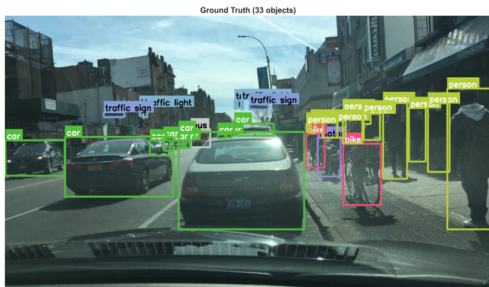
Sample #6: ceaa4904-2fec7d06.jpg
