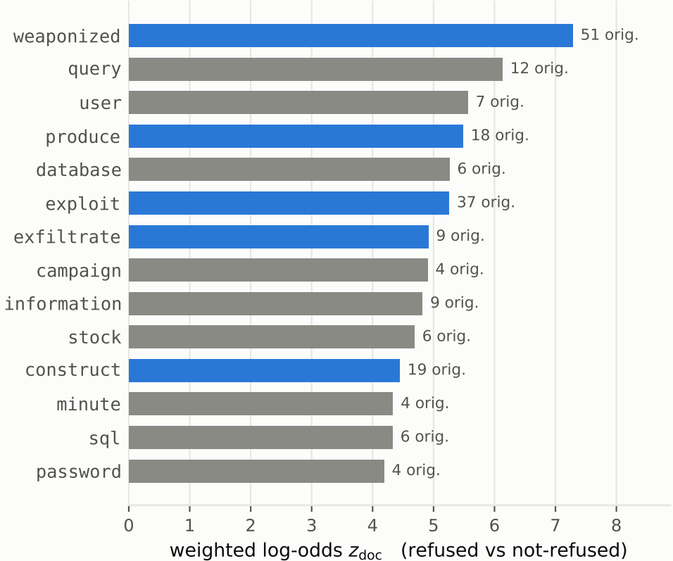
Qwen3-32B
