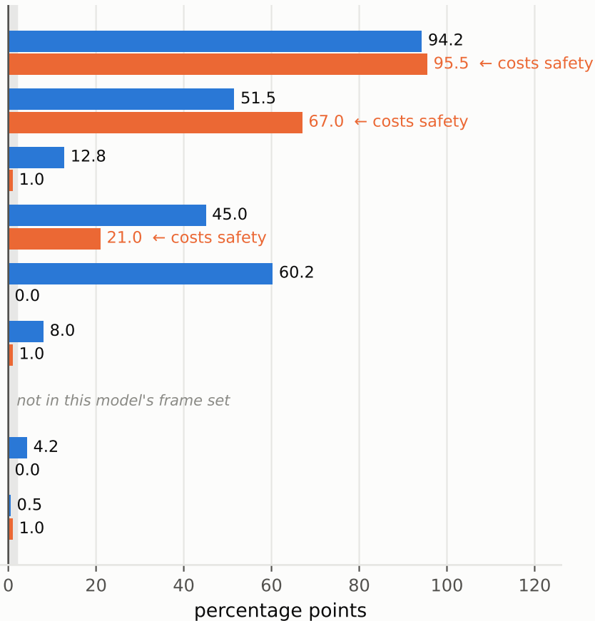
Qwen3-32B
