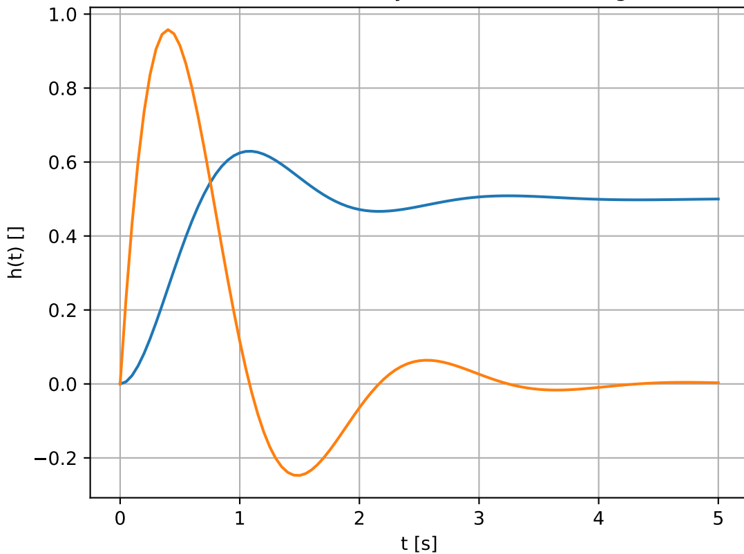
Stan układu dla wymuszenia skokowego
