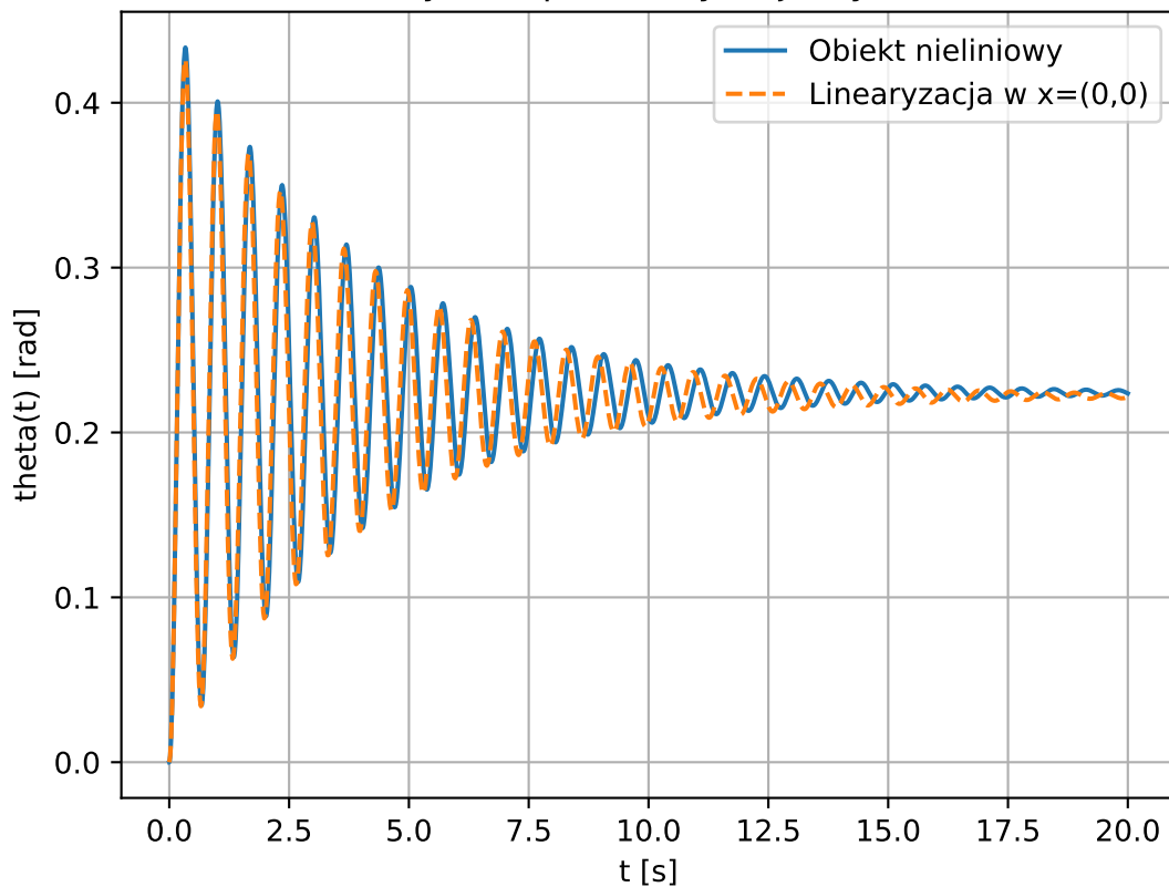
Model nieliniowy oraz po linearyzacji, wymuszenie u=20
