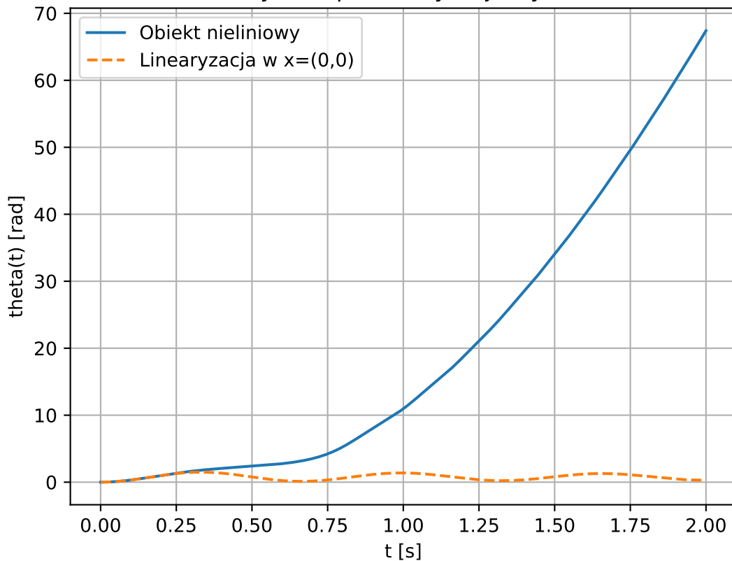
Model nieliniowy oraz po linearyzacji, wymuszenie u=70
