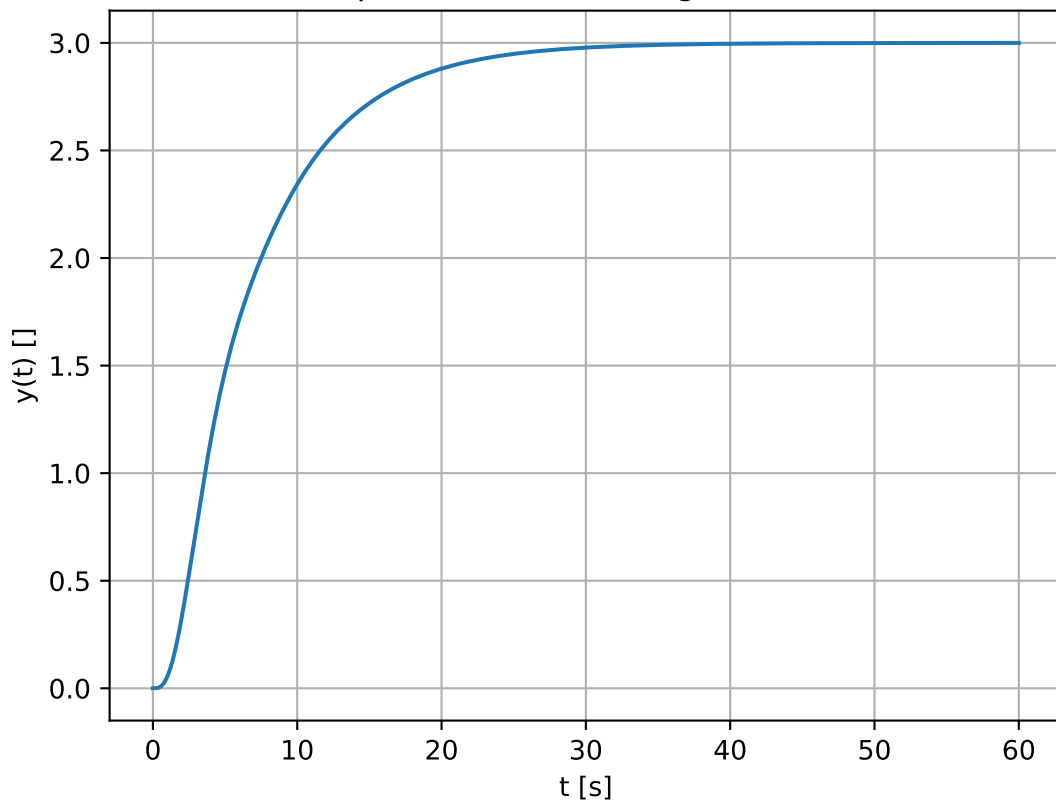
Odpowiedź układu z regulatorem I
