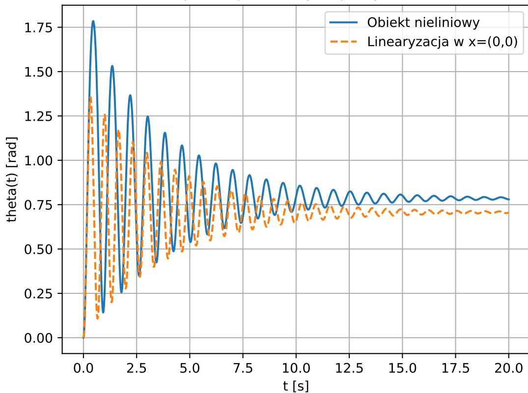
Model nieliniowy oraz po linearyzacji, wymuszenie u=45\sqrt{2}
