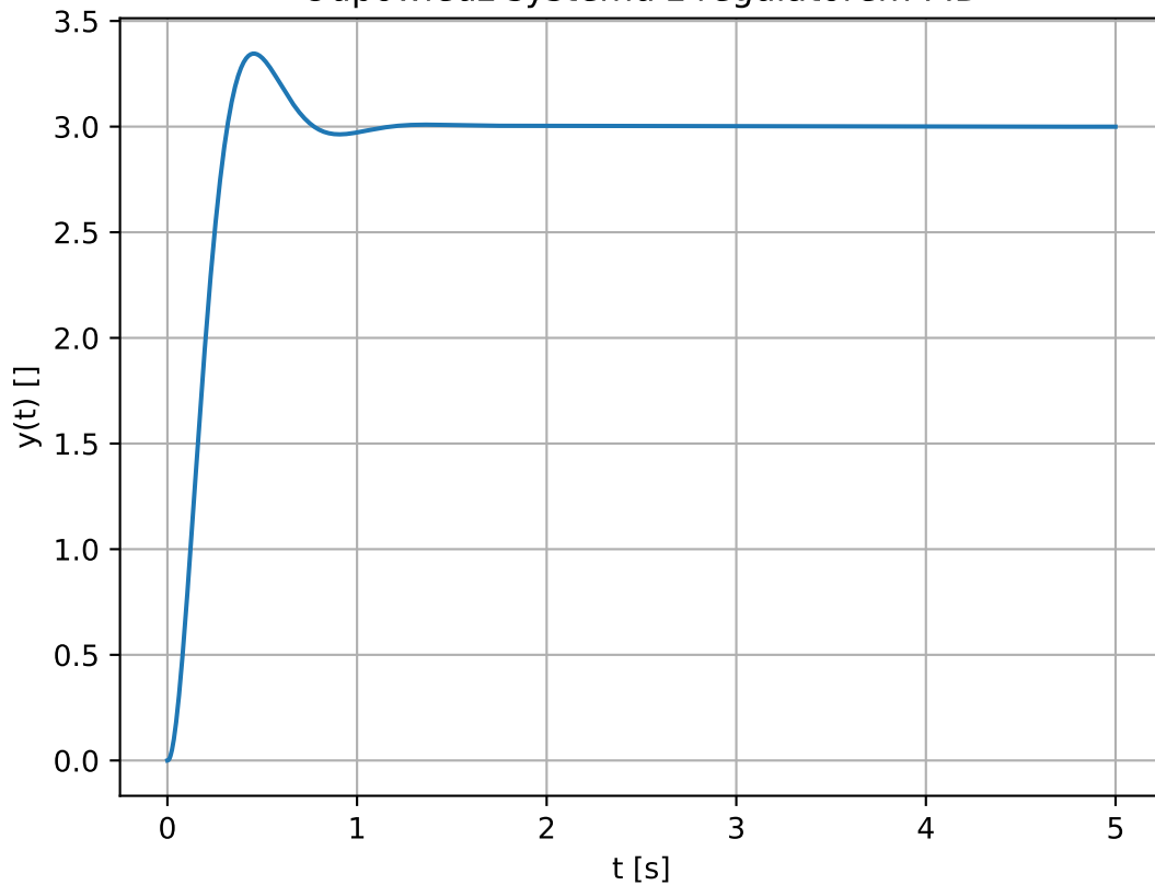
Odpowiedź systemu z regulatorem PID
