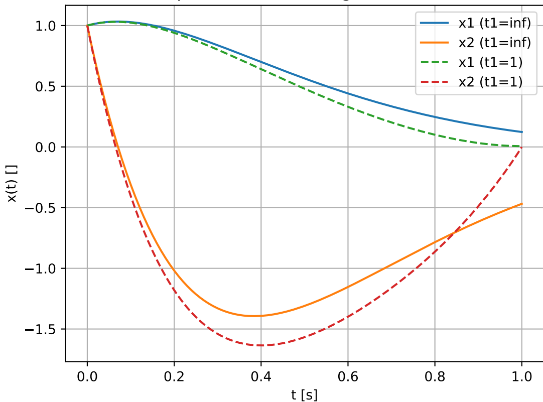
Porównanie odpowiedzi układu z regulatorami LQR dla t_1=1s
