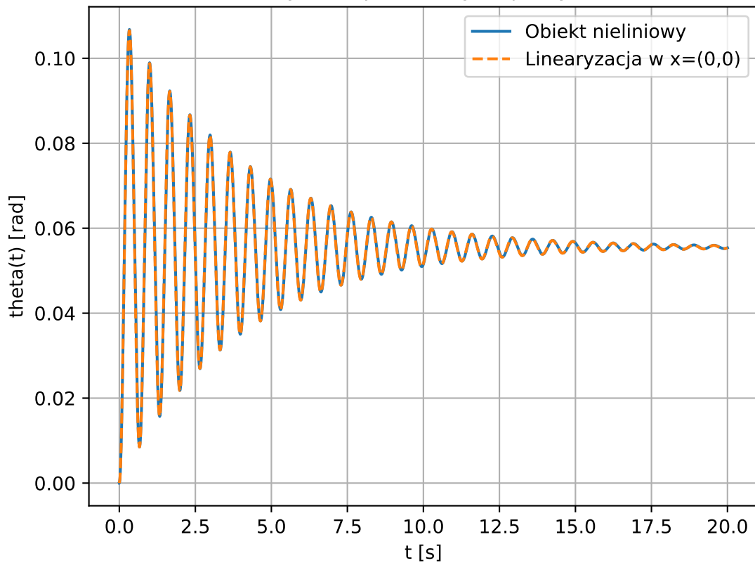
Model nieliniowy oraz po linearyzacji, wymuszenie u=5
