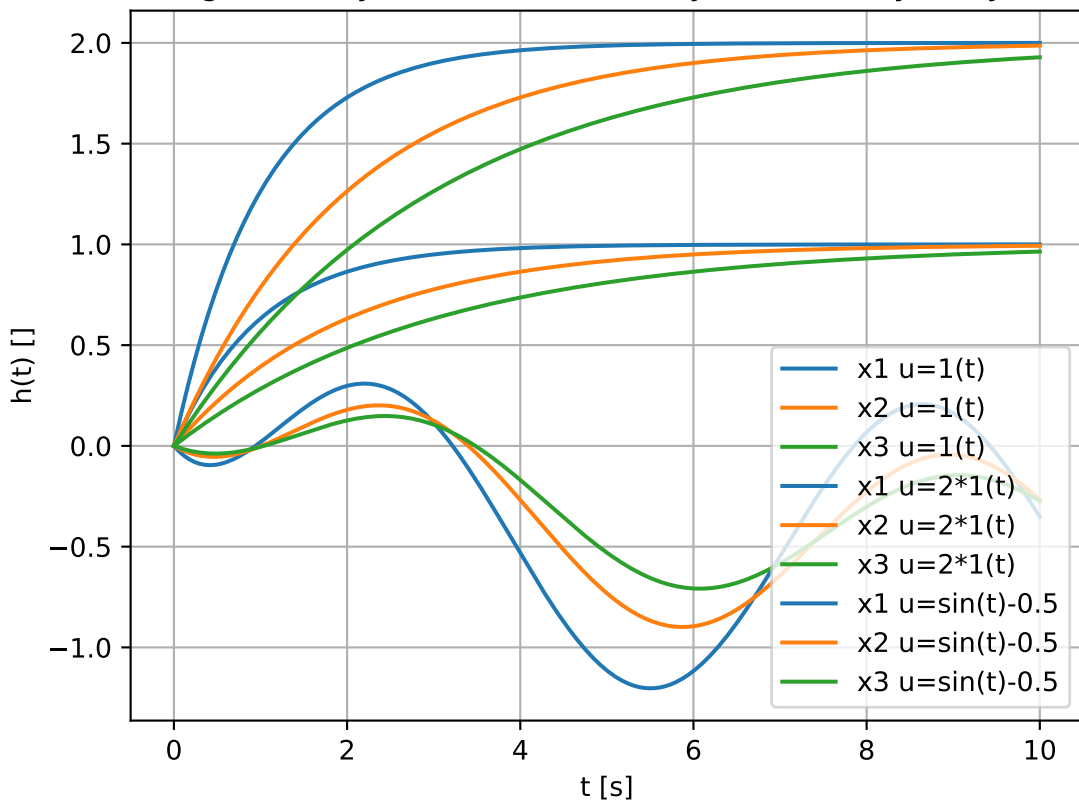
Przebiegi zmiennych stanu układu z Rys.2 dla różnych wymuszeń
