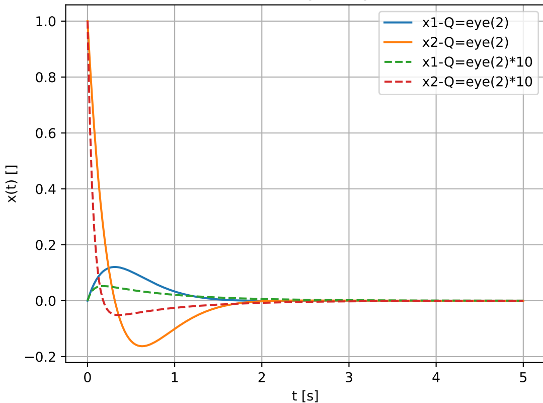
Stan układu zamkniętego z regulatorem LQR
