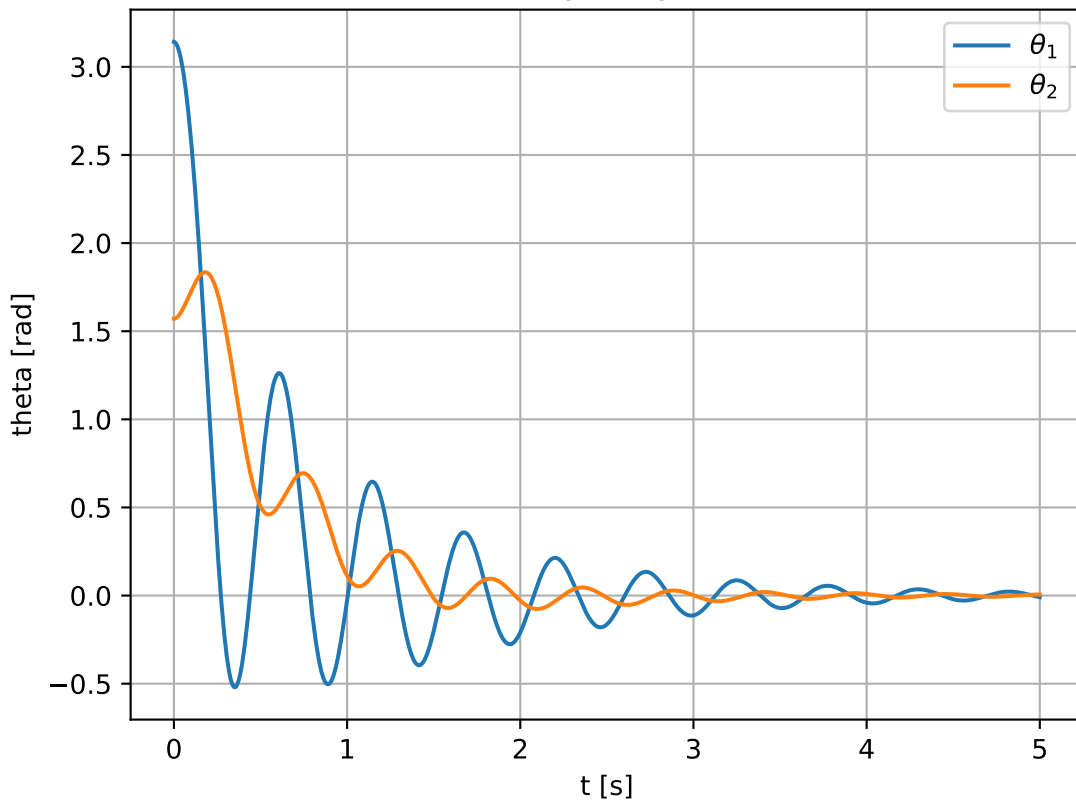
Układ nieliniowy z regulatorem LQR
