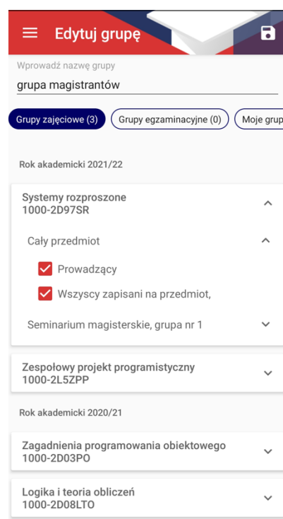
Rysunek 14 Okno dodawania studentów i prowadzących grup zajęciowych
