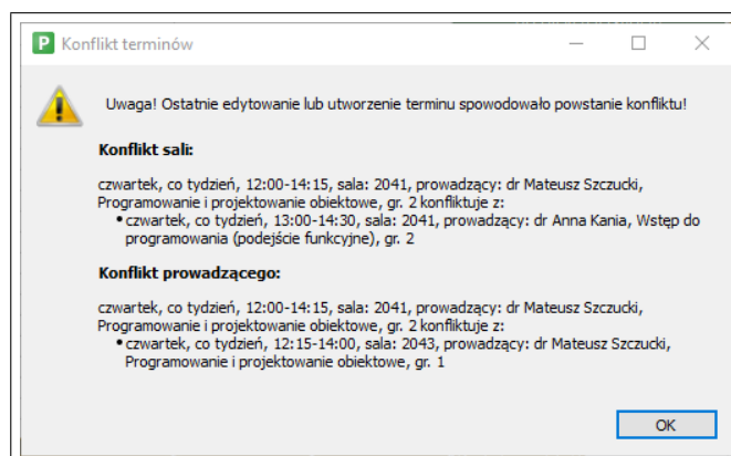
Rysunek 5.8: Komunikat konfliktu
