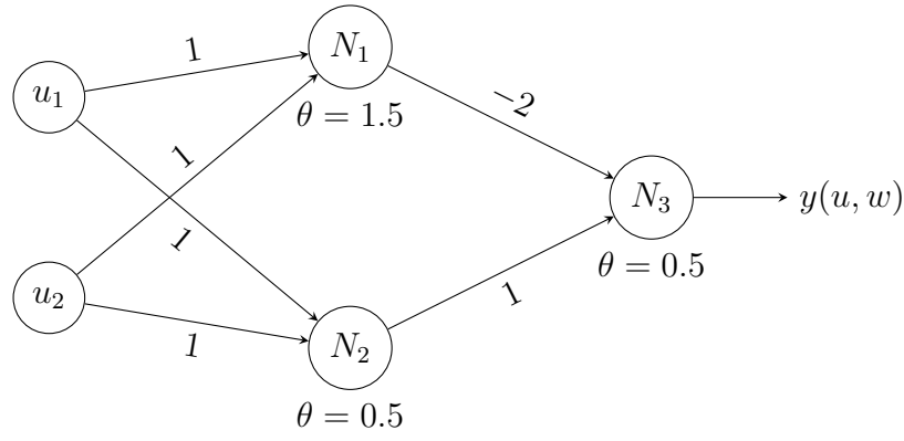
Figura 1: Rete neurale per risolvere il problema XOR
