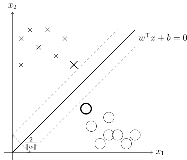
Figura 8: Support Vector Machine: l'iperpiano ottimo (linea piena), i margini (linee tratteggiate), e i support vectors (figure spesse).
