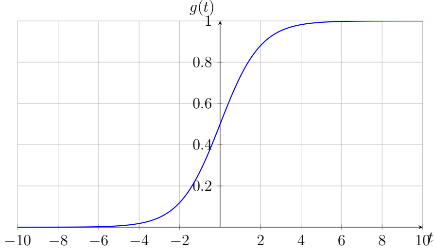
Figura 2: Grafico della funzione logistica g(t) = \frac{1}{1+e^{-t}} .
