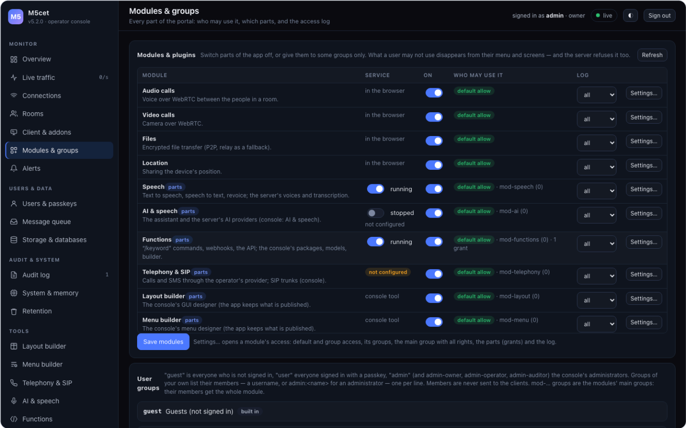
Obr. 22 — Konzole > Modules & groups (5.2): moduly aplikace i nástroje konzole, přepínače služeb (Speech a Functions běží, AI bez poskytovatele), kdo smí modul používat, hlavní skupiny ( mod-... ) a granty, úroveň logu.
