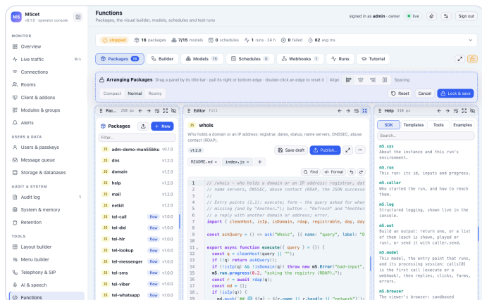
Obr. 61 — Functions > Packages odemčené: seznam, editor a nápověda jako panely s úchyty a krají k tažení.
