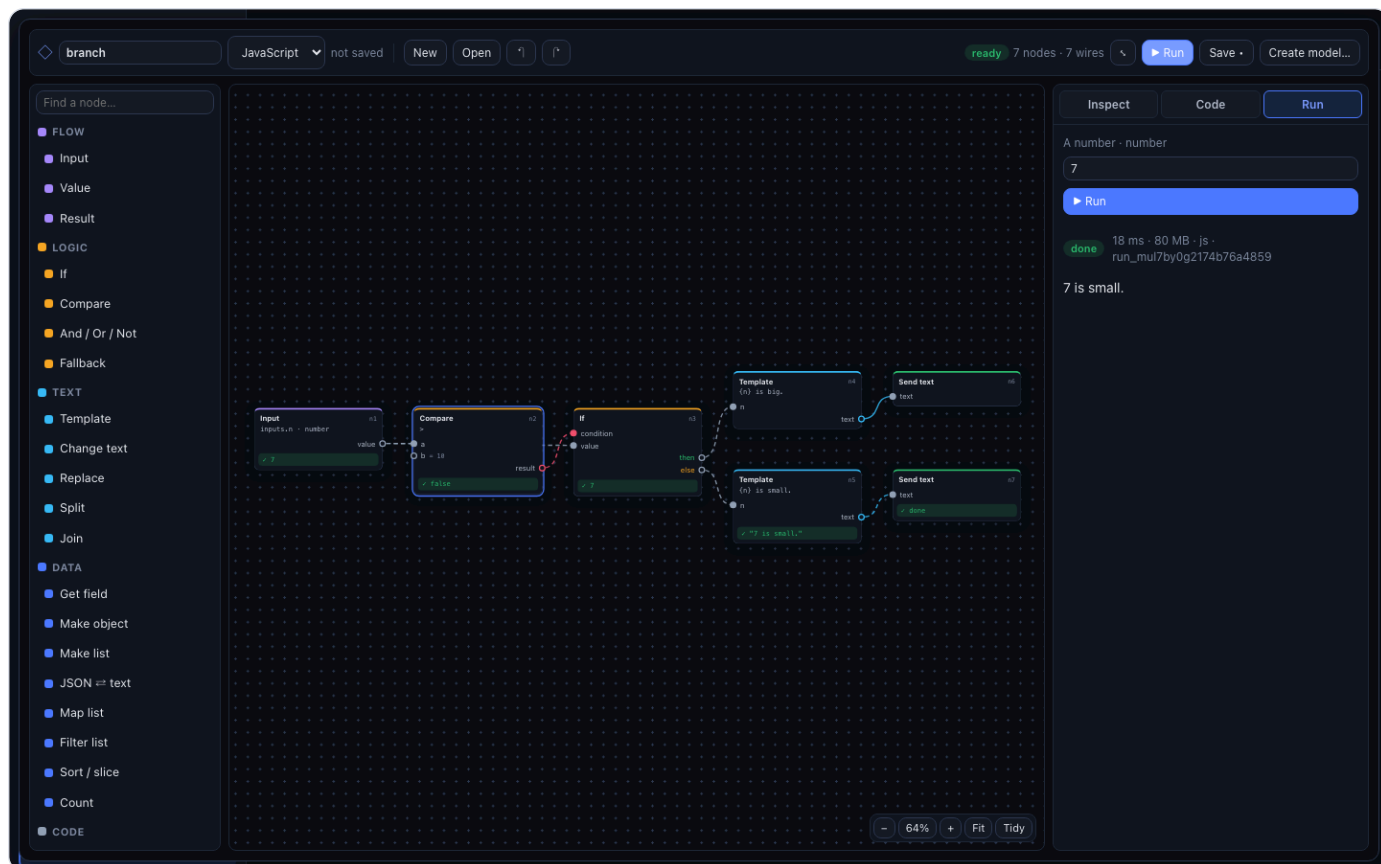
Obr. 41 — Vizualní tvůrce na celé obrazovce: příklad Branch po běhu s hodnotou 7 — každý uzel ukazuje svou hodnotu, větev „big“ neběžela.
