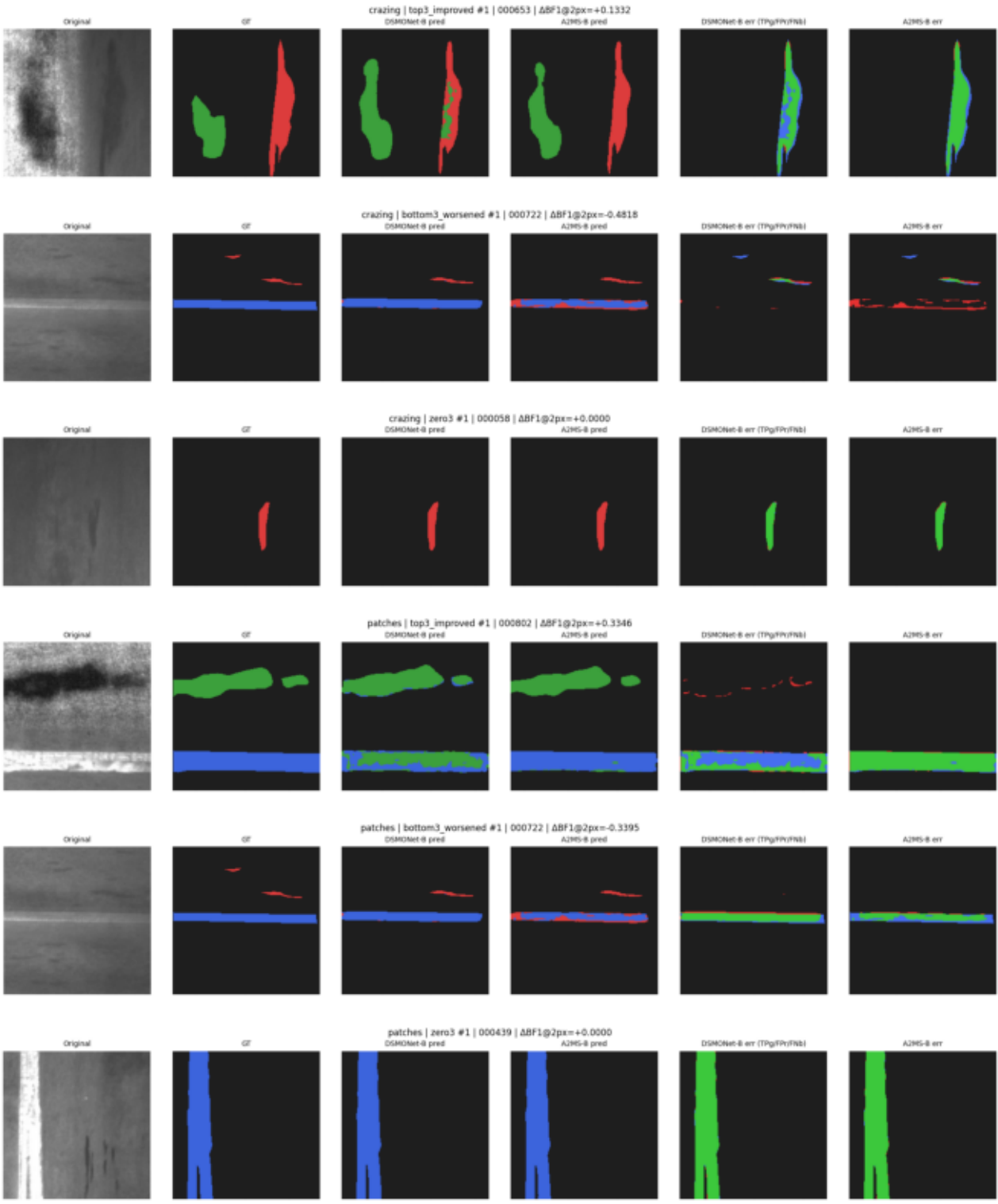
NEU-Seg 可视化 (每行: 原图 / GT / DSMoNet-B / A2MS-DSMoNet-B / DSMoNet-B 误差 / A2MS 误差)
