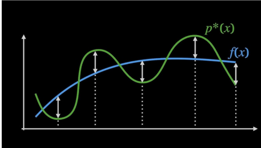
FIGURE 2 – Algo de Remez :on approche f par P , en minimisant l'erreur maximal
