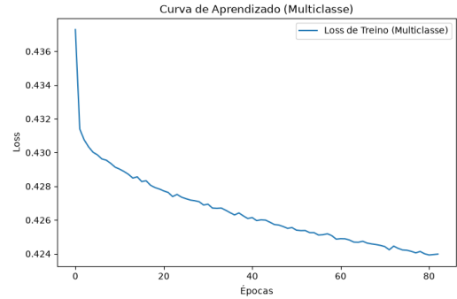
(b) Curva de Aprendizado (Multiclasse)
