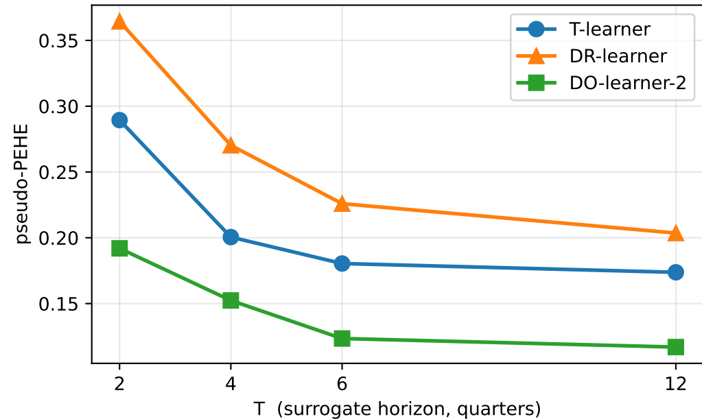
Pseudo-PEHE vs T
