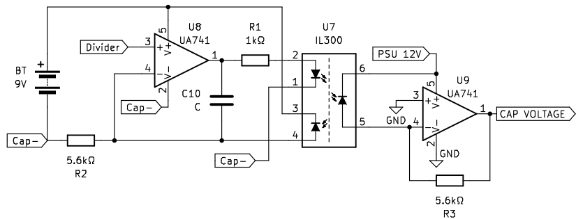
Linear Optocoupler Circuit
