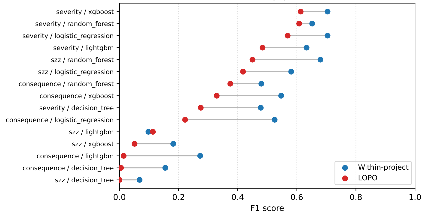
Generalization gap: F1 score
