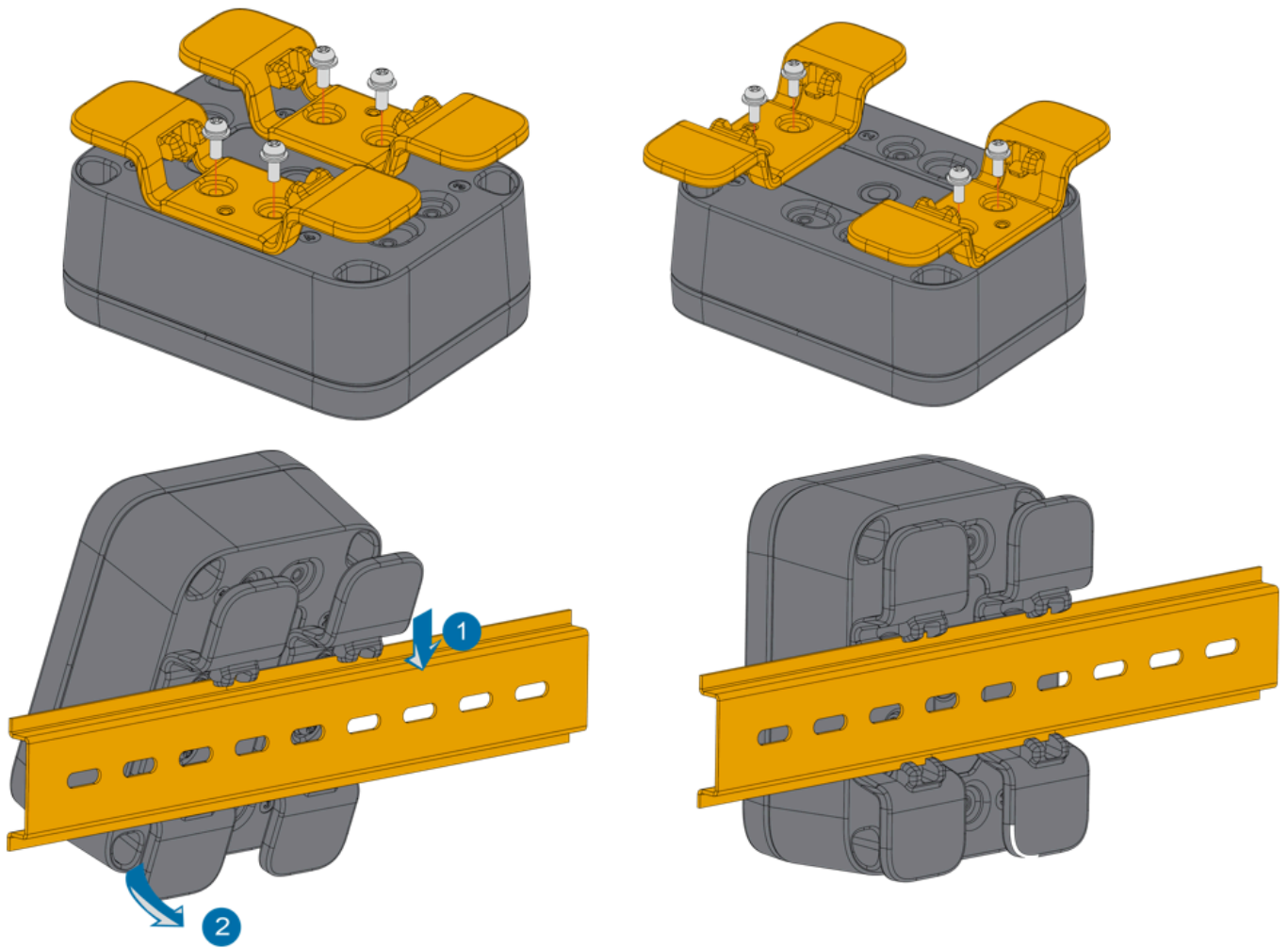
Figure 8: DIN mount
