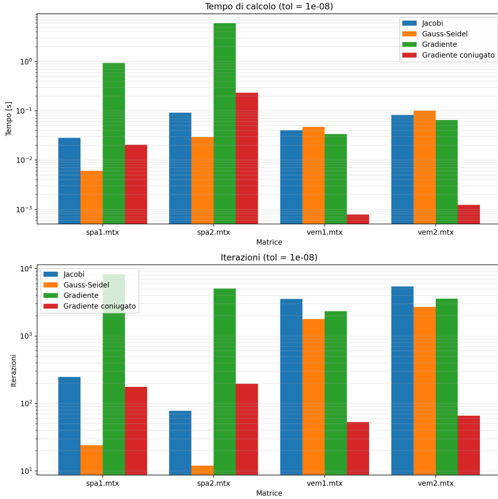
Figura 6: Confronto a barre del tempo (sopra) e delle iterazioni (sotto) a \text{tol} = 10^{-8} . Assi delle ordinate in scala logaritmica.
