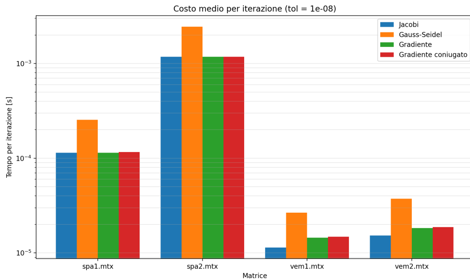
Figura 5: Tempo medio per iterazione a \text{tol} = 10^{-8} . Asse delle ordinate in scala logaritmica.
