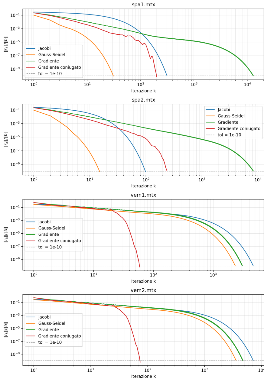
Figura 4: Storia del residuo scalato \|\mathbf{r}_k\|/\|\mathbf{b}\| in funzione dell'iterazione k ( \text{tol} = 10^{-10} , entrambi gli assi in scala logaritmica, una riga per matrice; la linea tratteggiata segna la tolleranza).
