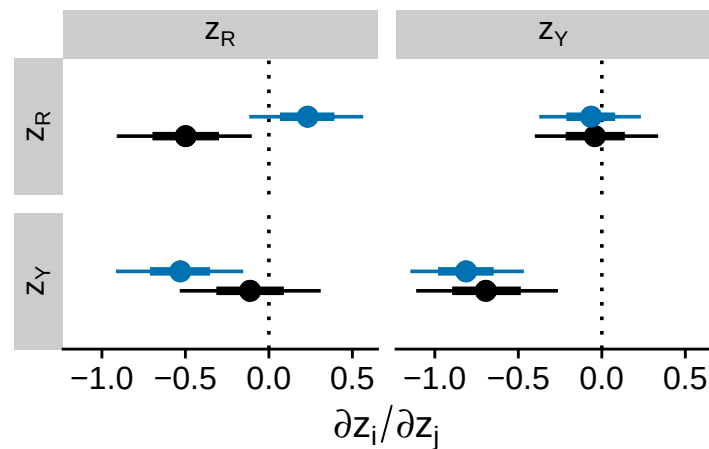
Evolutionary feedback (D)
