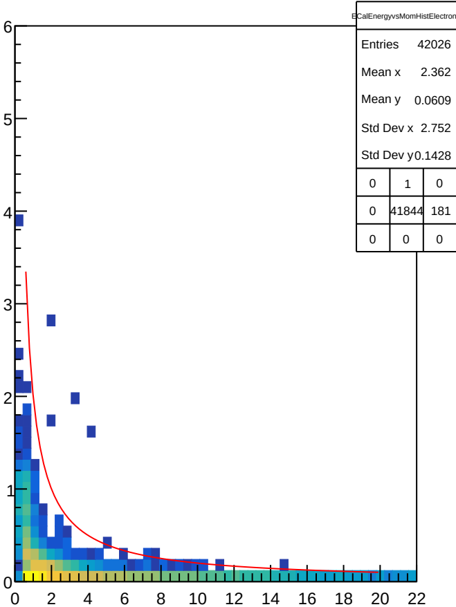
ECalEnergyvsMomHistElectrons
