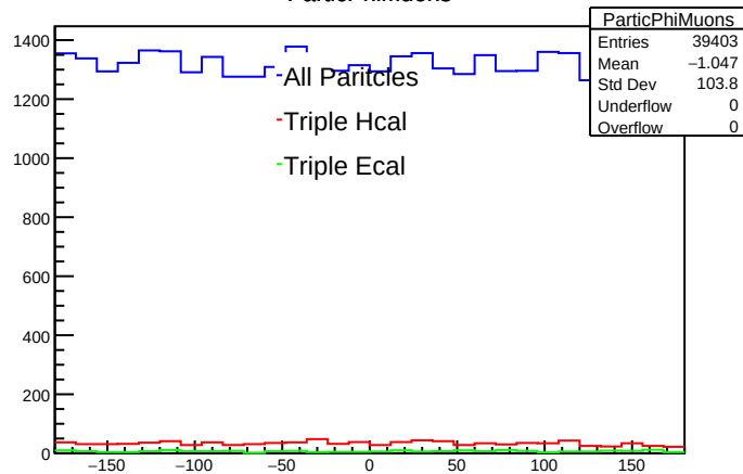
ParticPhiMuons
