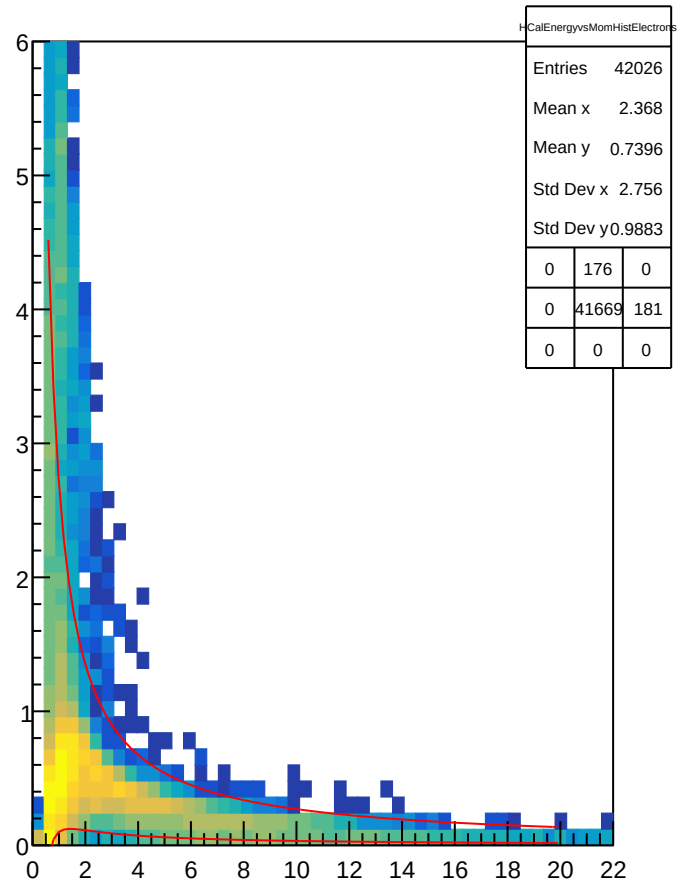
HCalEnergyvsMomHistElectrons
