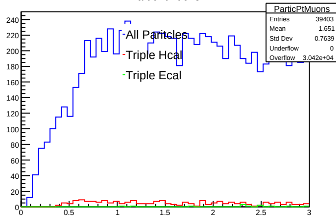
ParticPtMuons
