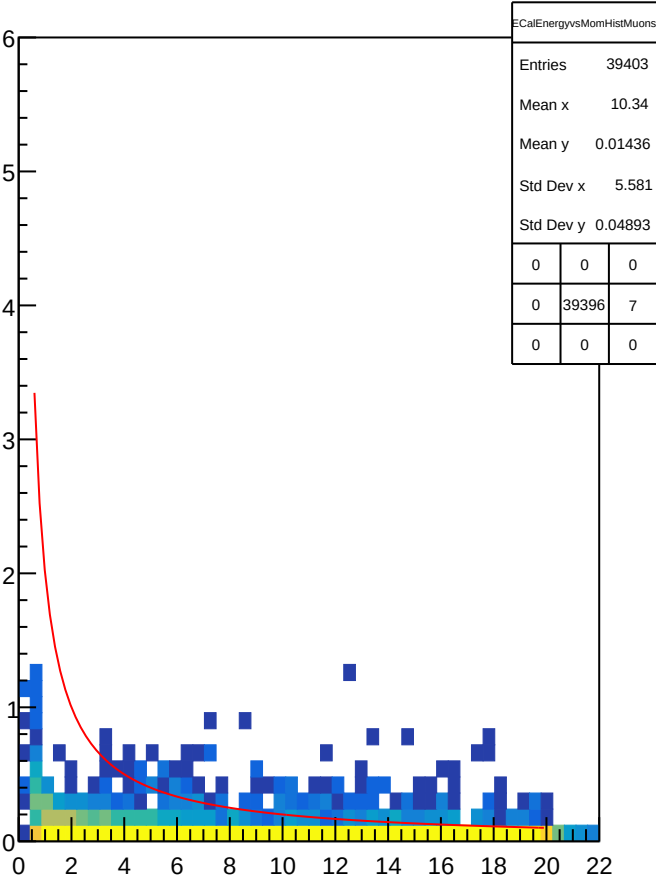
ECalEnergyvsMomHistMuons
