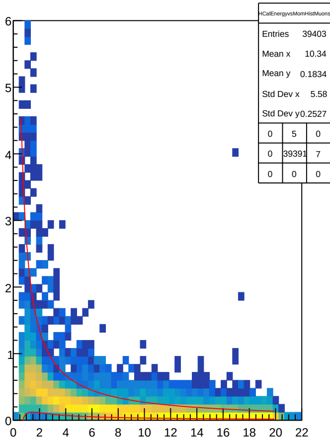
HCalEnergyvsMomHistMuons
