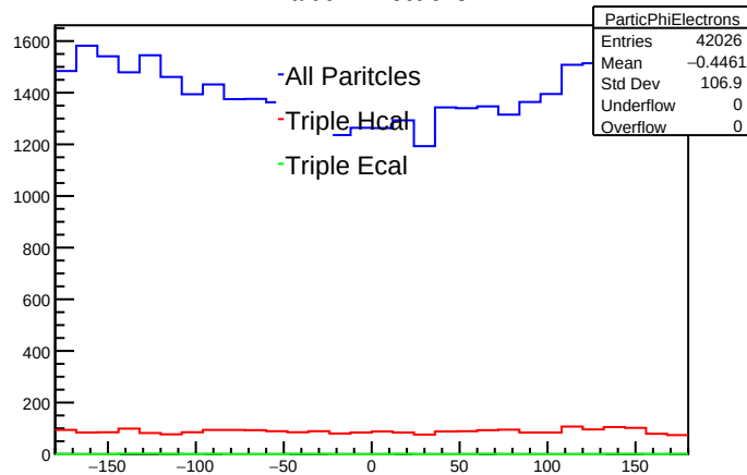
ParticPhiElectrons
