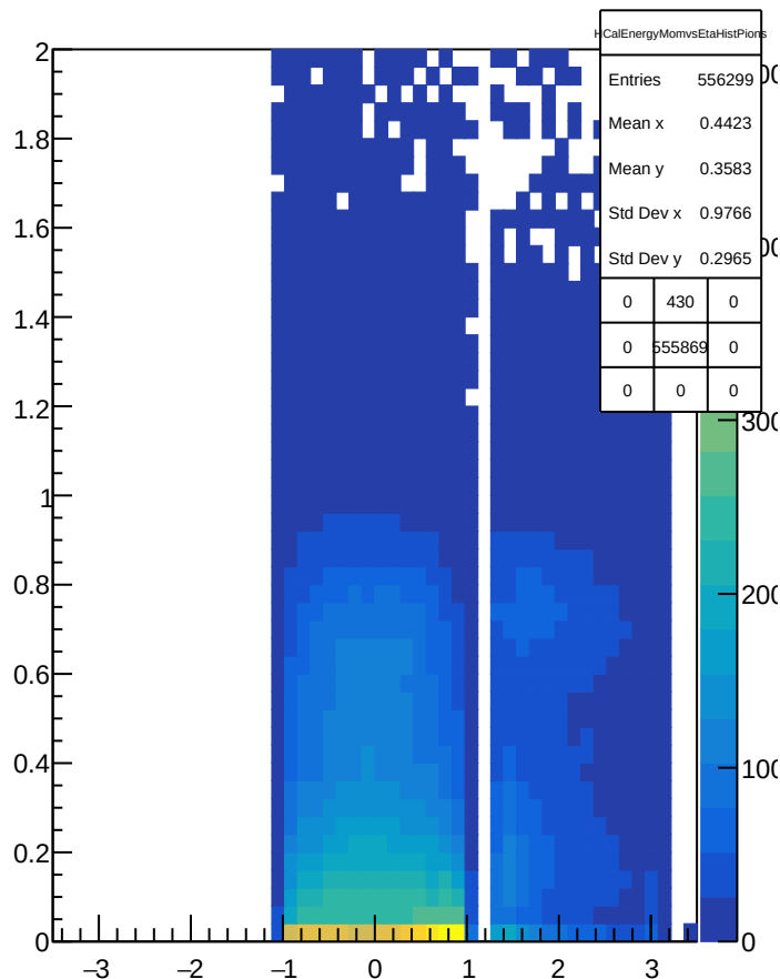
HCalEnergyMomvsEtaistPions
