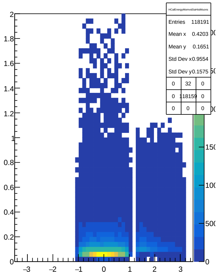
HCalEnergyMomvsEtaistMuons
