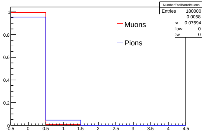
NumberEcalBarrelMuons
