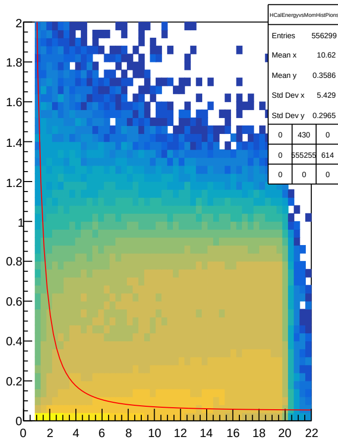
HCalEnergyvsMomHistPions
