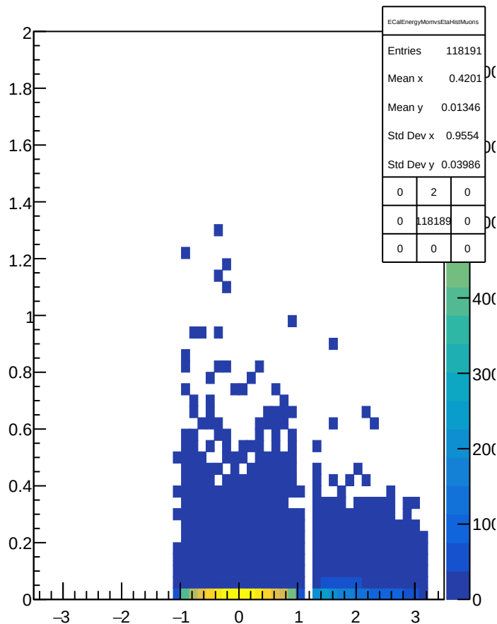
ECalEnergyMomvsEtaistMuons
