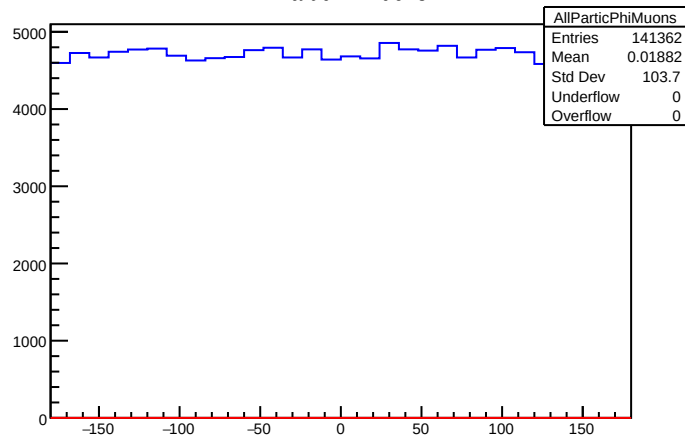
AllParticPhiMuons
