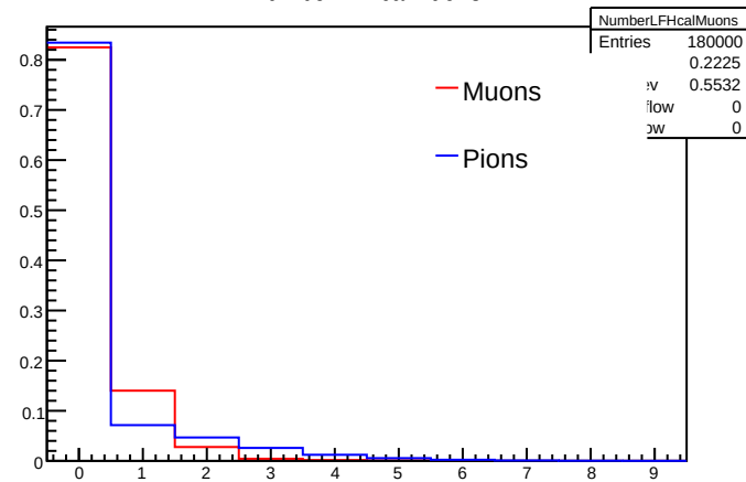
NumberLFHcalMuons
