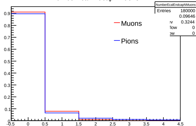
NumberEcalEndcapNMuons
