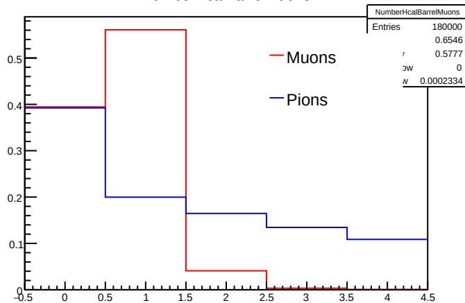
NumberHcalBarrelMuons
