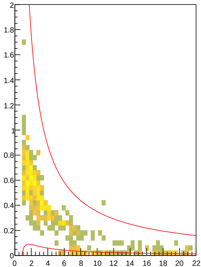
HCalEnergyvsMomHistPions
