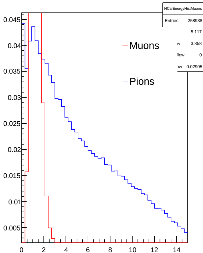
HCalEnergyHistMuons
