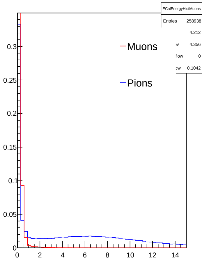
ECalEnergyHistMuons
