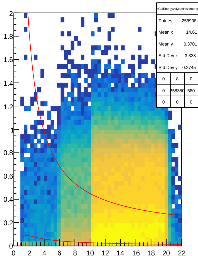
HCalEnergyvsMomHistMuons
