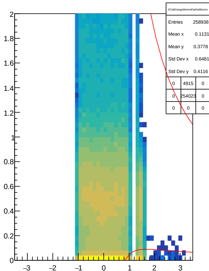
ECalEnergyMomvsEtaistMuons
