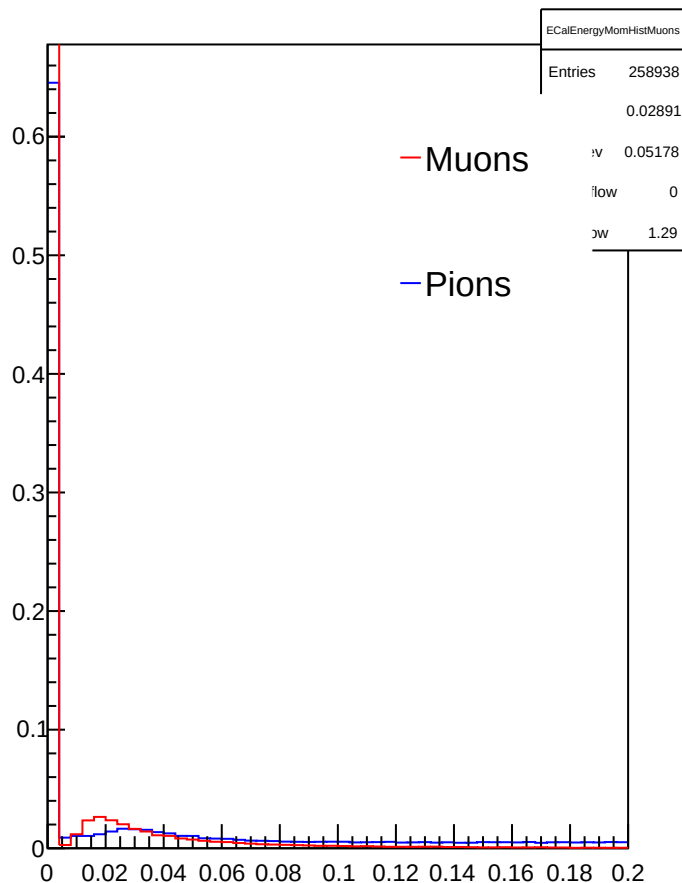
ECalEnergyMomHistMuons
