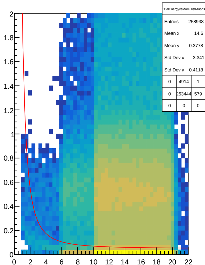
ECalEnergyvsMomHistMuons
