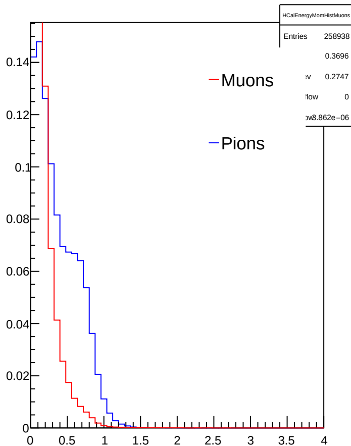
HCalEnergyMomHistMuons
