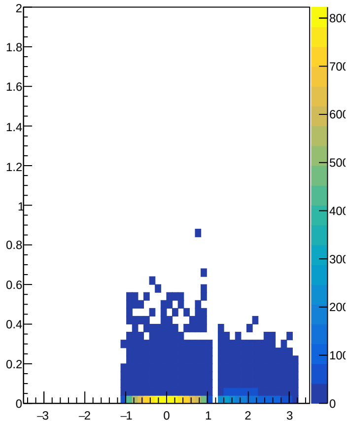
ECalEnergyMomvsEtaistMuons
