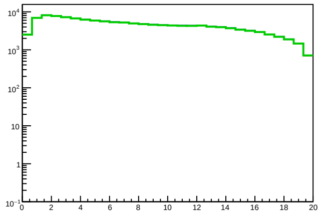
AllParticPtMuons
