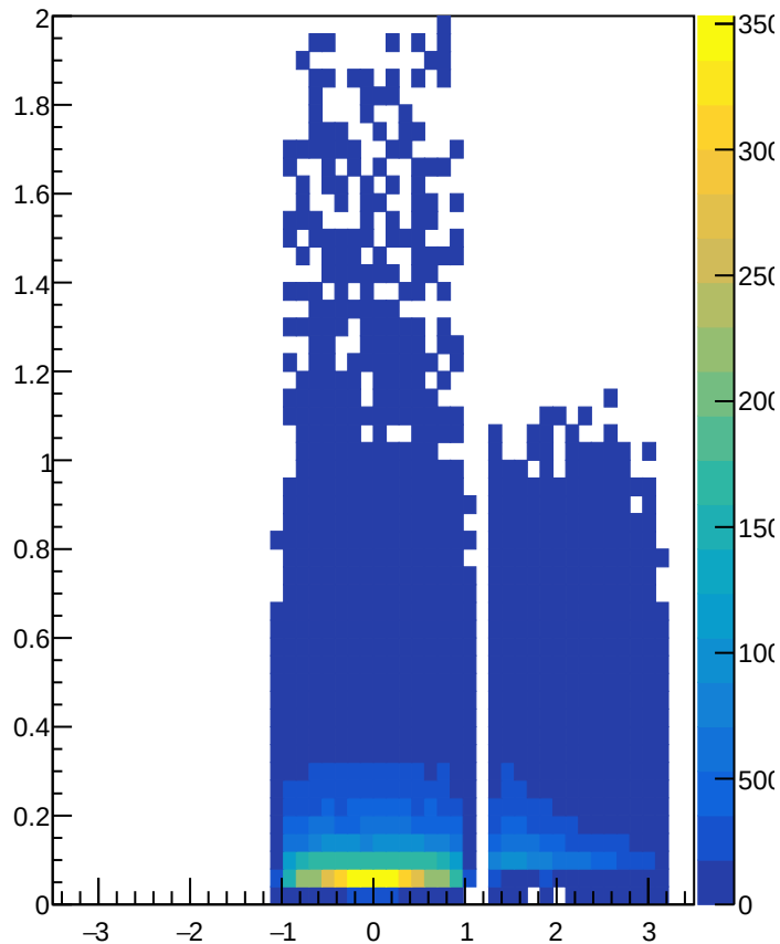
HCalEnergyMomvsEtaistMuons
