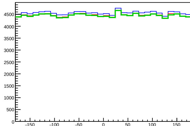
AllParticPhiMuons
