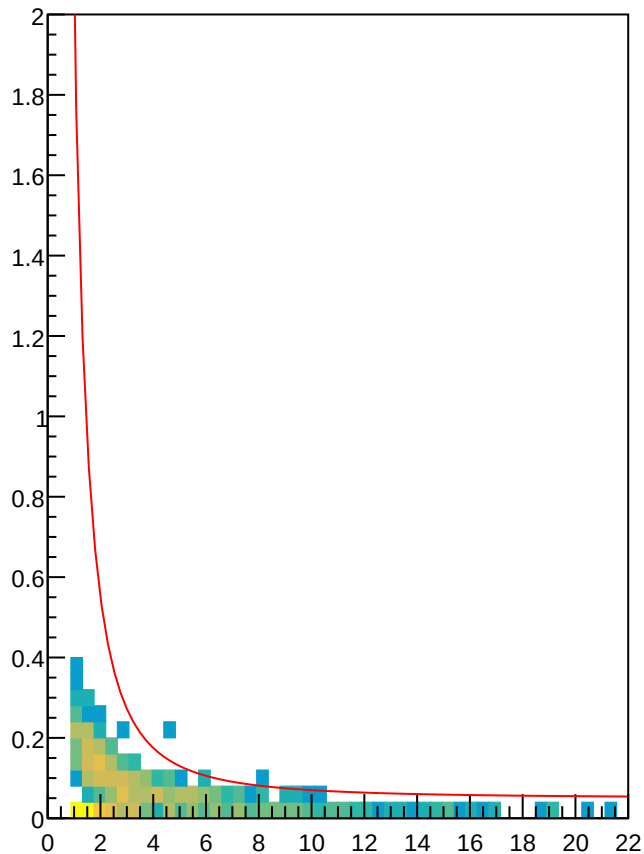
ECalEnergyvsMomHistMuons
