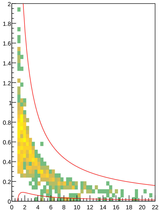
HCalEnergyvsMomHistMuons
