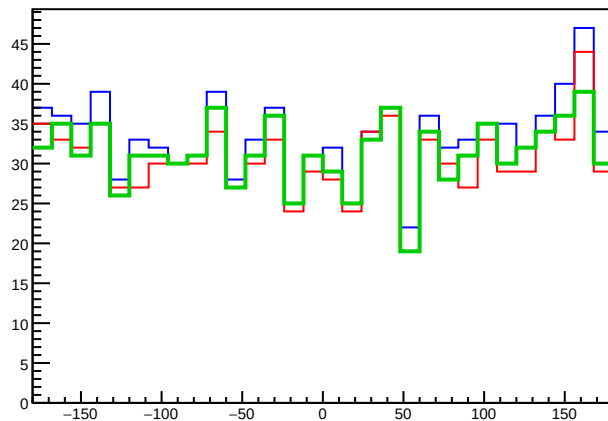
AllParticPhiMuons
