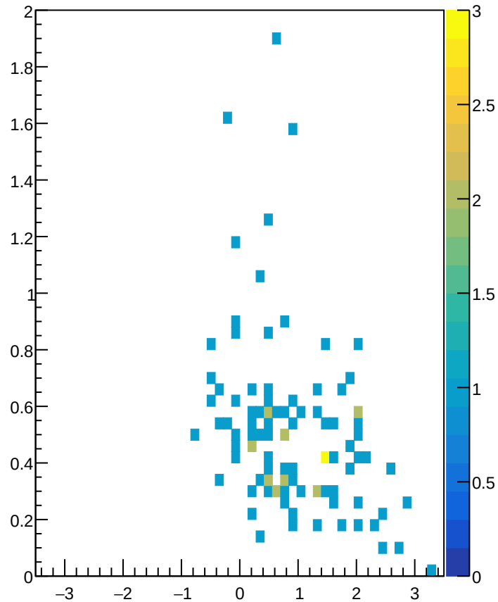
HCalEnergyMomvsEtaistPions
