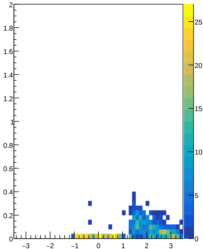
ECalEnergyMomvsEtaistMuons
