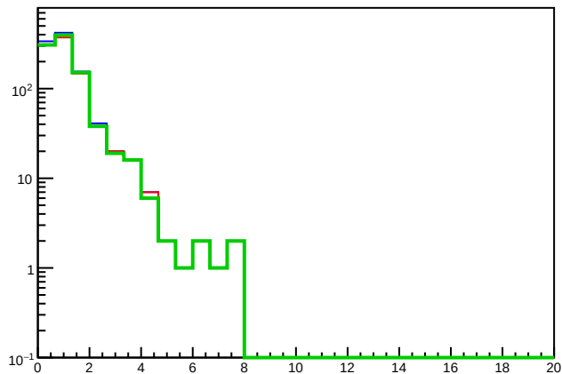
AllParticPtMuons
