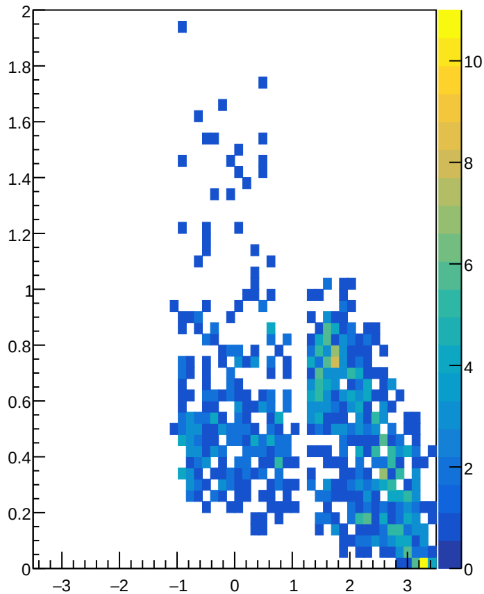
HCalEnergyMomvsEtaistMuons
