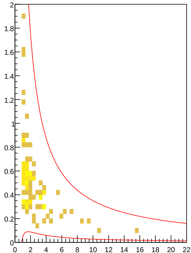
HCalEnergyvsMomHistPions
