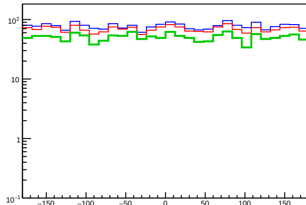
AllParticPhiPions
