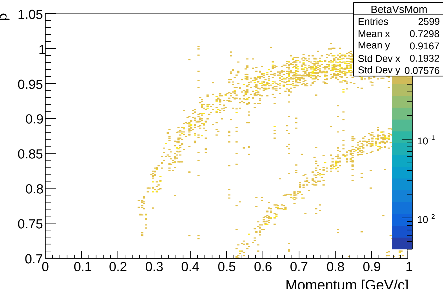
BetaVsMom
