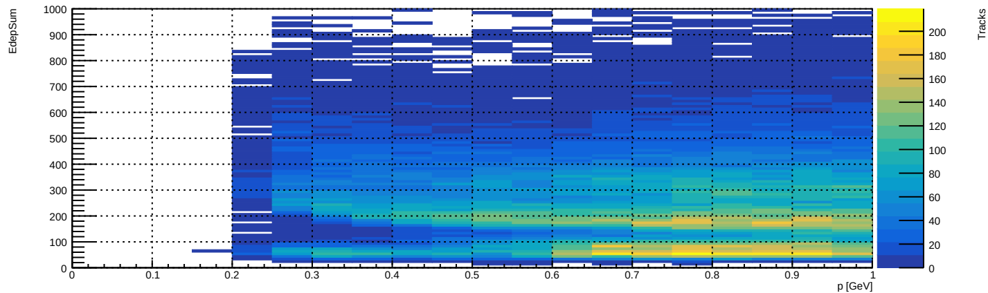
EdepSum vs P - Muon
