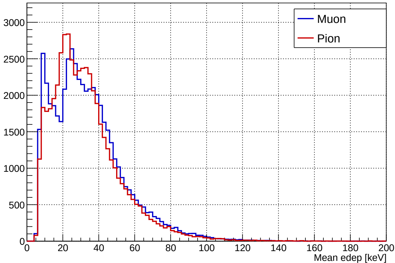
Mean edep per hit
