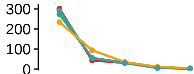
TcMar-MITE (DNA)
