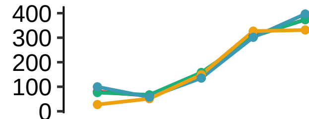
nMITE (DNA)
