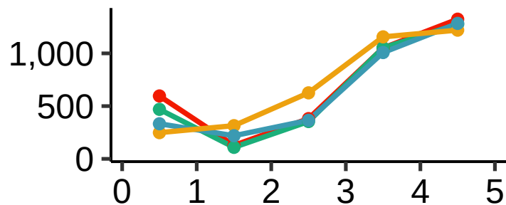
Gypsy (LTR)
