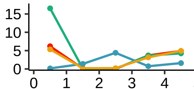
MIR (SINE)
