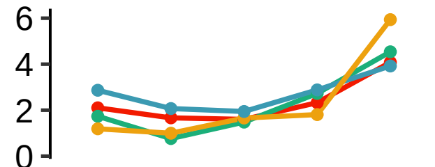
Mutator-nMITE (DNA)
