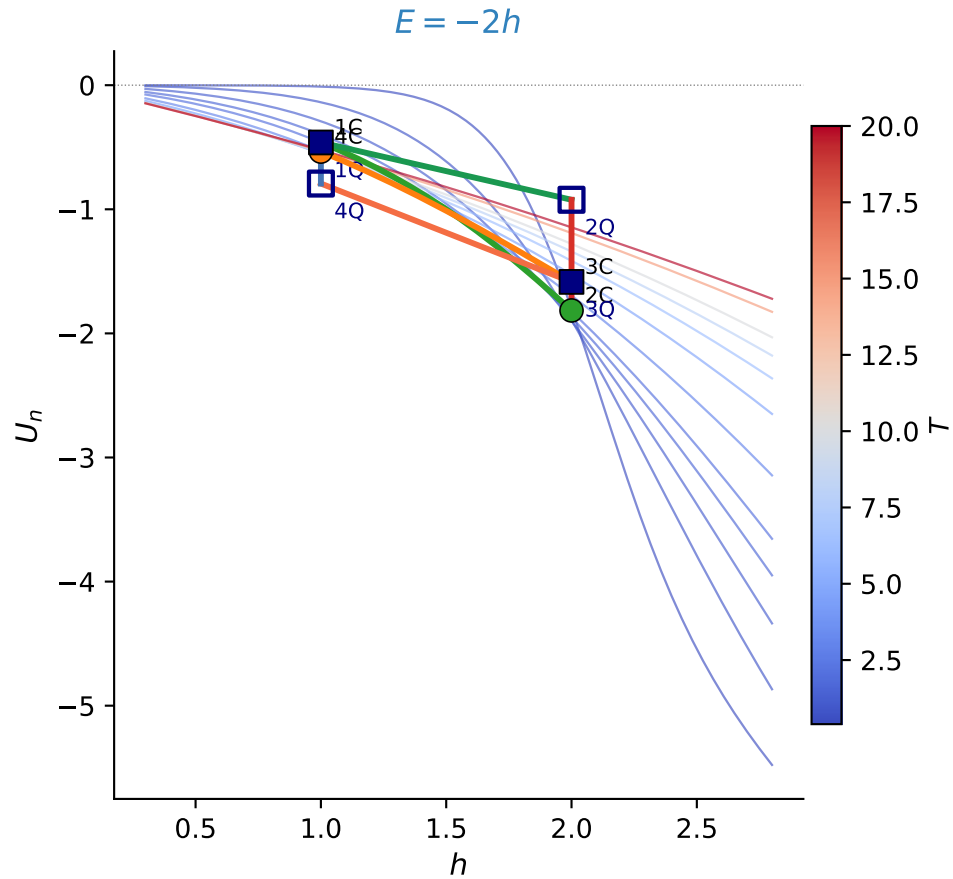
Ciclo de Otto no espaço (h, U_n) — iso- T de fundo J=0.51 h_i=1.0 h_f=2.0 T_c=2.0 T_h=4.0
