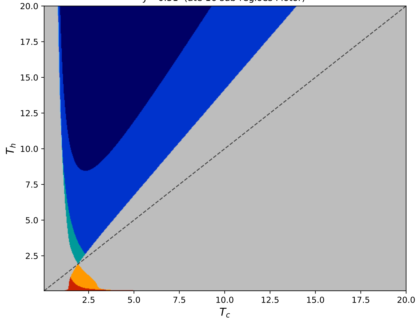
Thermodynamics — Strong J = 0.51 (até 16 sub-regiões Motor)
