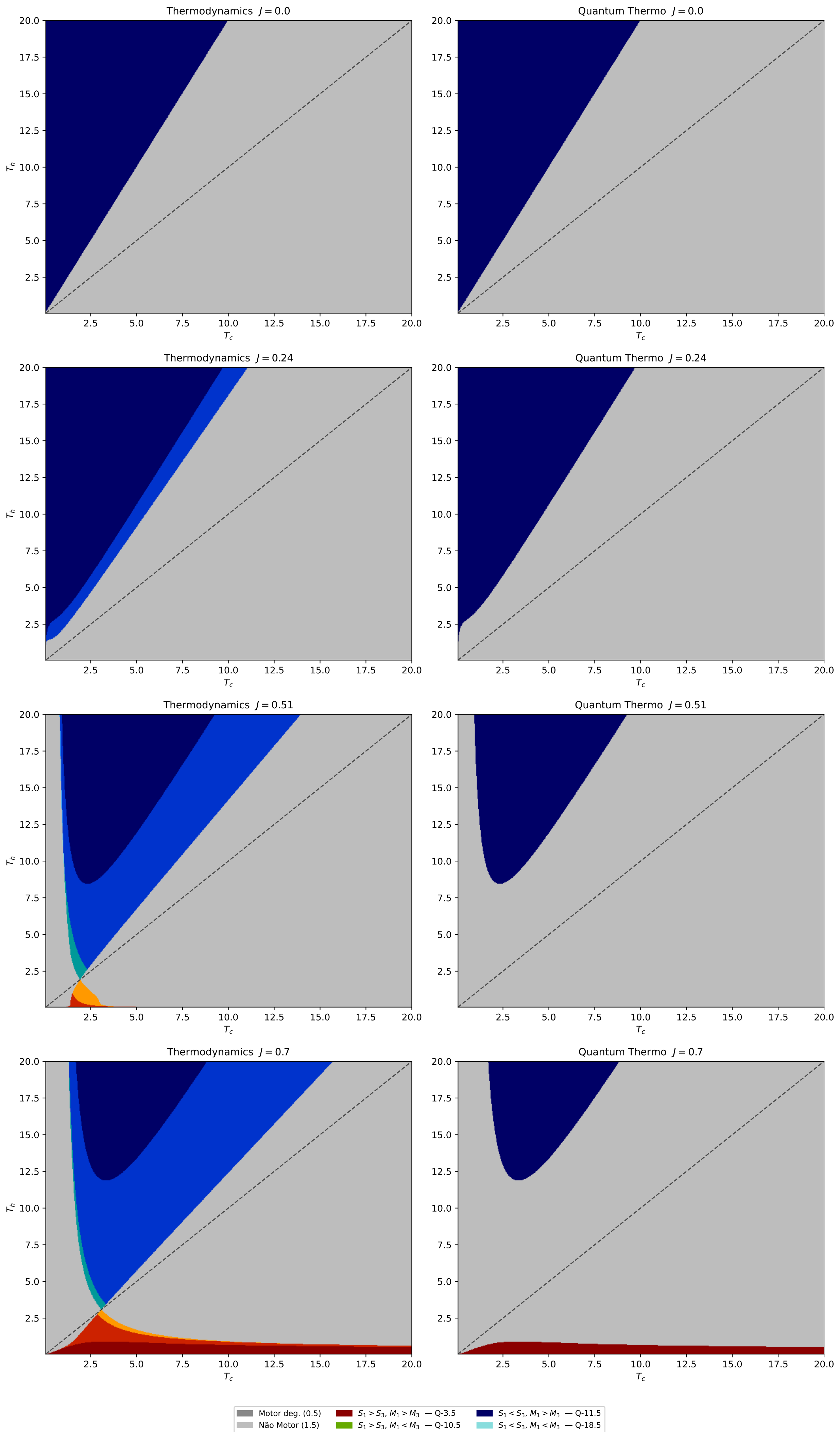
Strong Conditions — Thermodynamics (left) vs Quantum Thermodynamics (right) Esquerda: até 16 sub-regiões Motor | Direita: M_2 = M_1, M_4 = M_3 \rightarrow 4 sub-regiões
