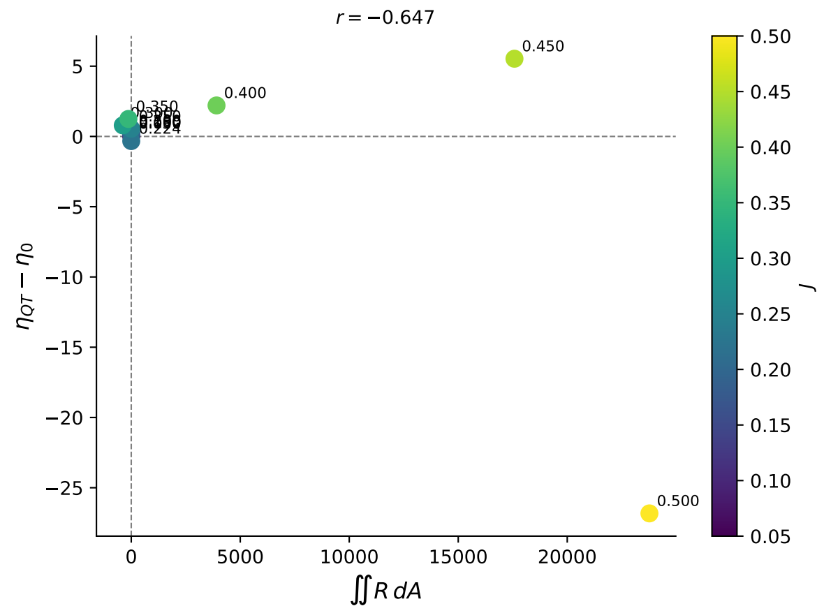
Correlação: curvatura de Ruppeiner vs ganho de eficiência h_{lo} = 1.0 , h_{hi} = 2.0 , T_c = 0.10 , T_h = 1.00
