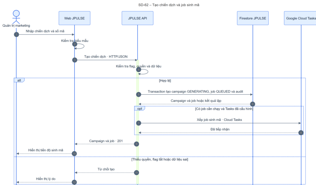
Hình 4-79: SD-62 tạo chiến dịch và job sinh mã
