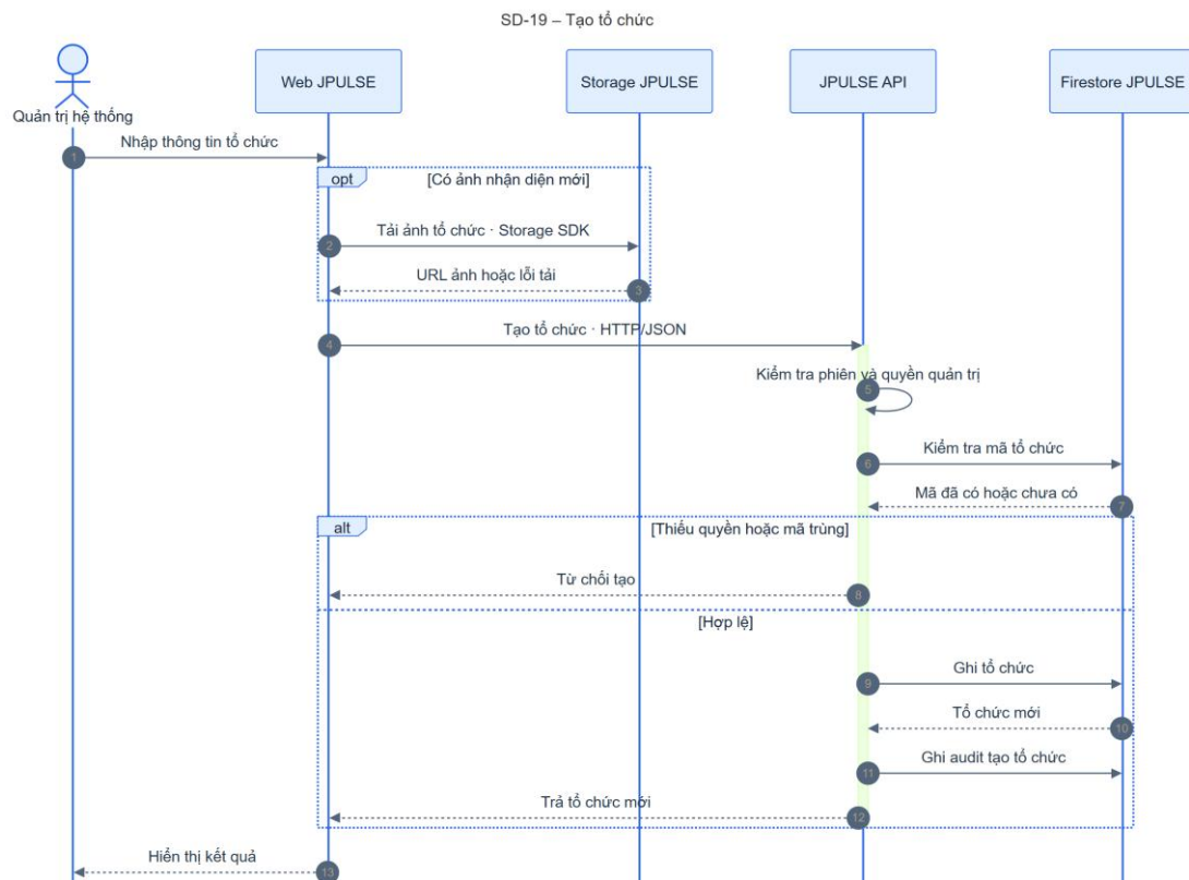
Hình 4-51: SD-19 tạo tổ chức
