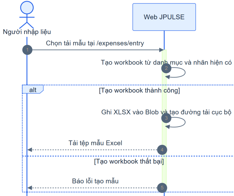
Hình 4-102: SD-85 tải mẫu Excel
