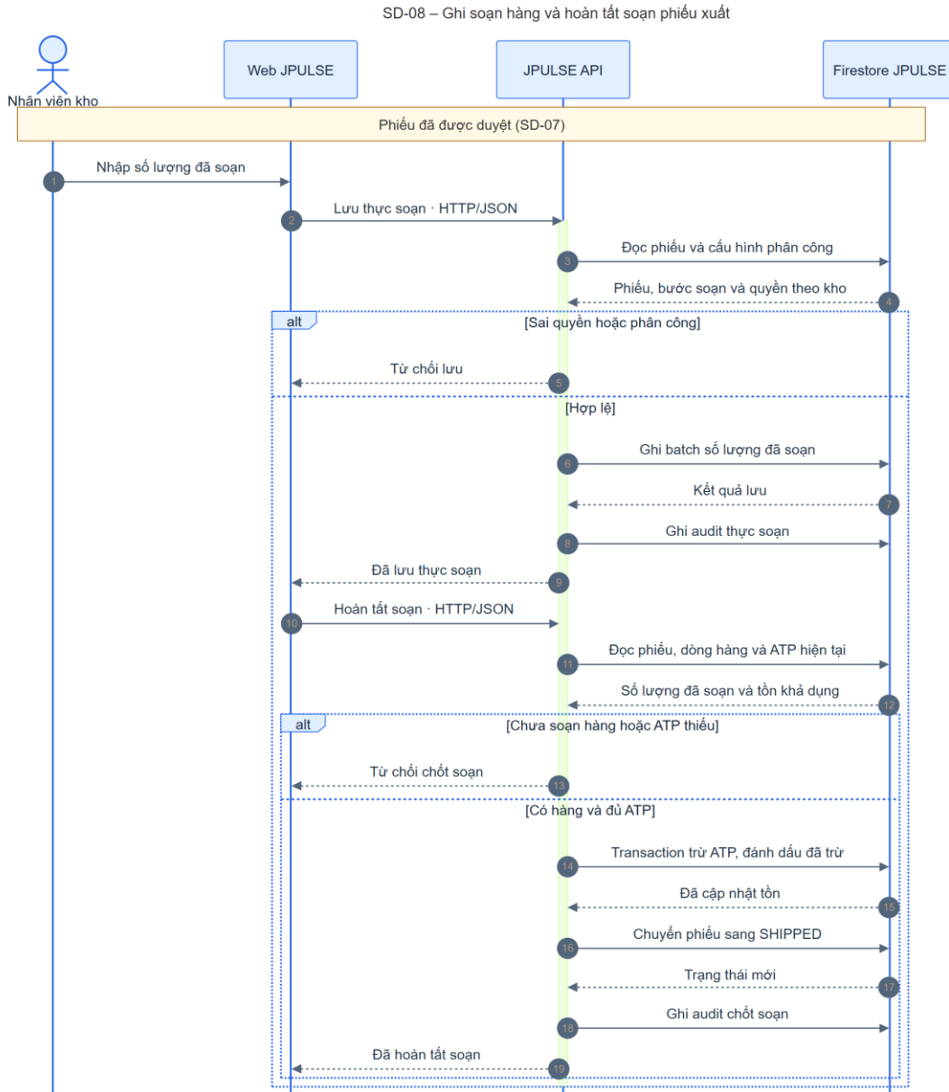
Hình 4-13: SD-08 soạn phiếu xuất
