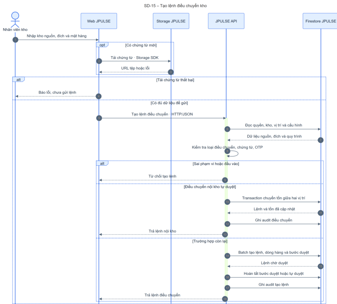
Hình 4-21: SD-15 tạo lệnh điều chuyển
