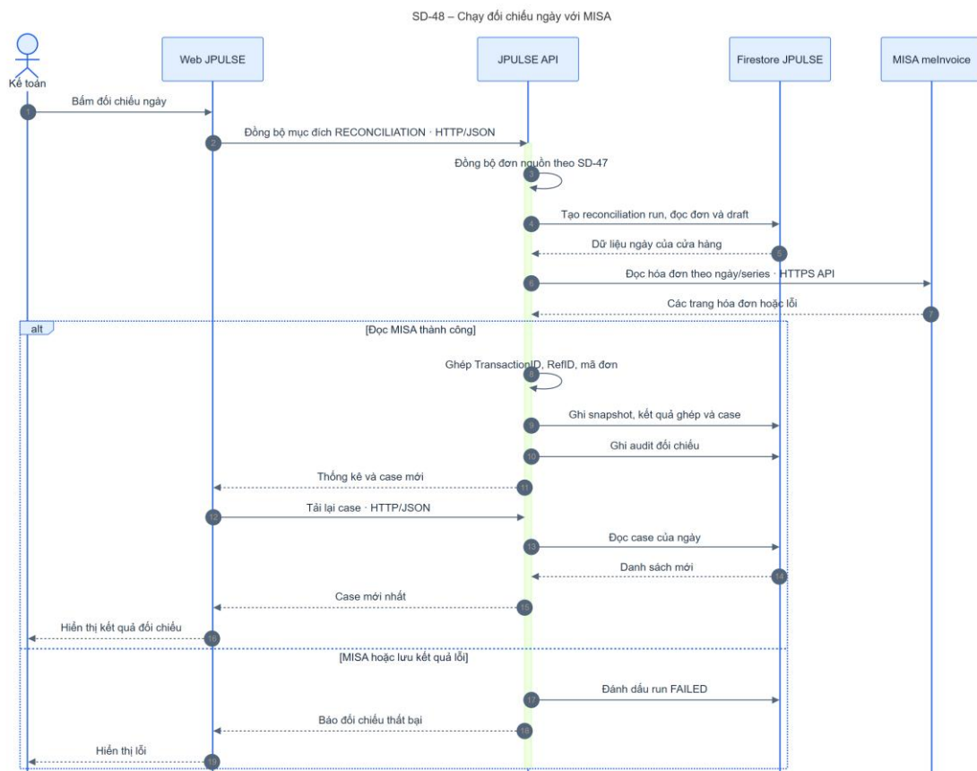
Hình 4-33: SD-48 chạy đối chiếu ngày với MISA
