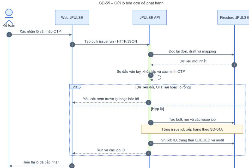
Hình 4-41: SD-55 gửi lô hóa đơn để phát hành
