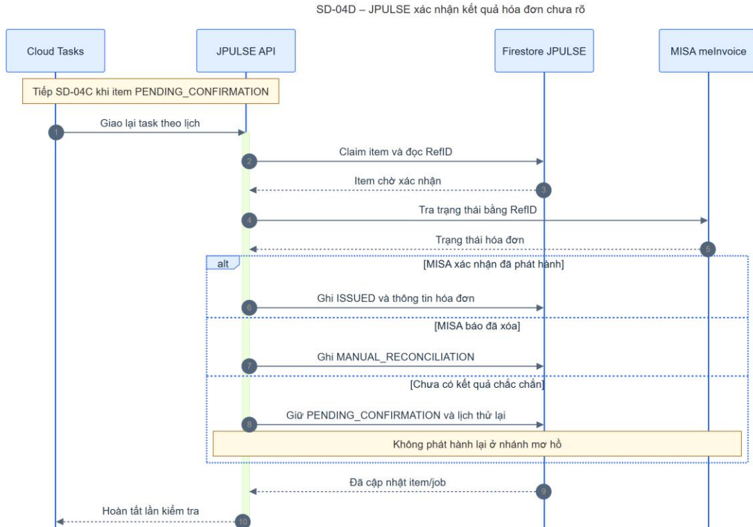
Hình 4-30: SD-04D xác nhận hóa đơn chưa rõ
