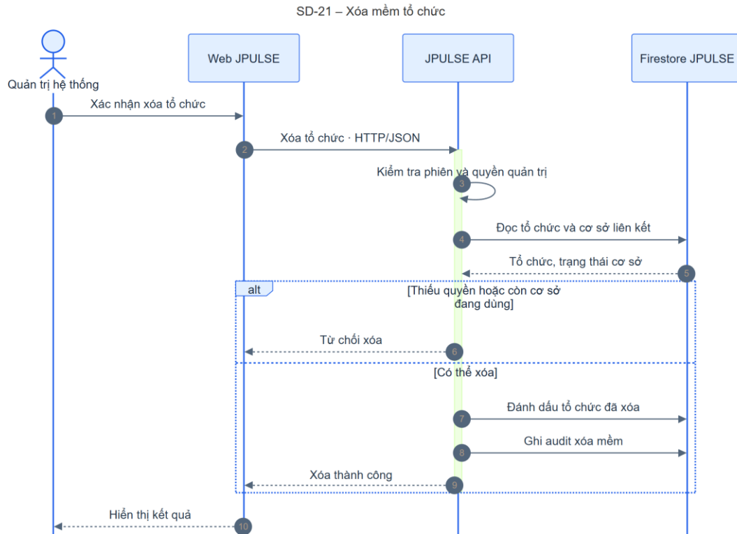
Hình 4-53: SD-21 xóa mềm tổ chức
