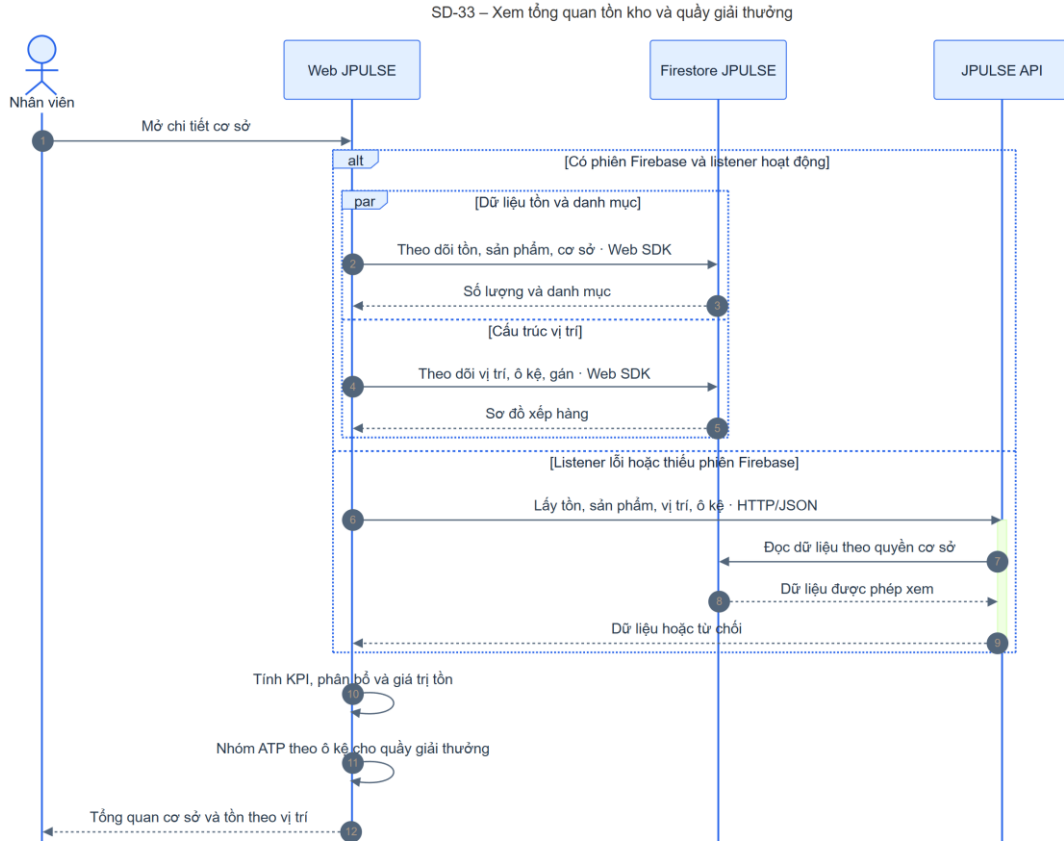
Hình 4-65: SD-33 xem tổng quan tồn kho và quầy giải thưởng
