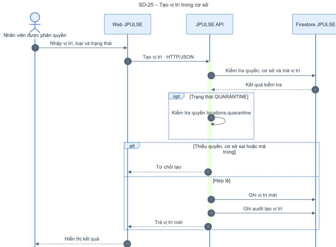
Hình 4-57: SD-25 tạo vị trí trong cơ sở
