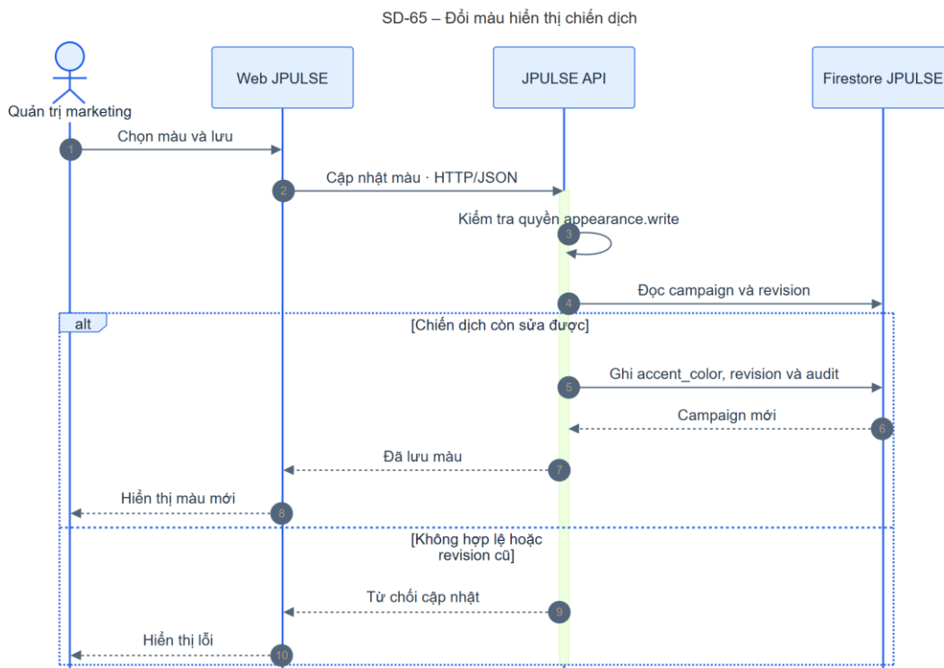
Hình 4-82: SD-65 đổi màu hiển thị chiến dịch
