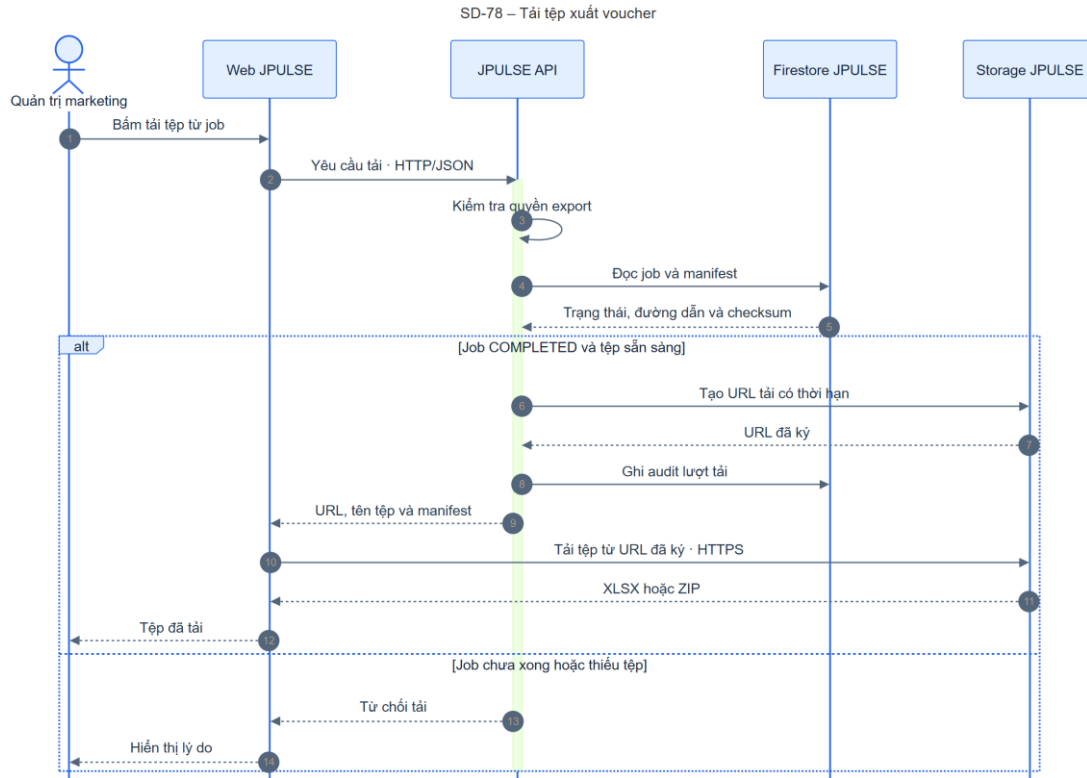
Hình 4-95: SD-78 tải tệp xuất voucher
