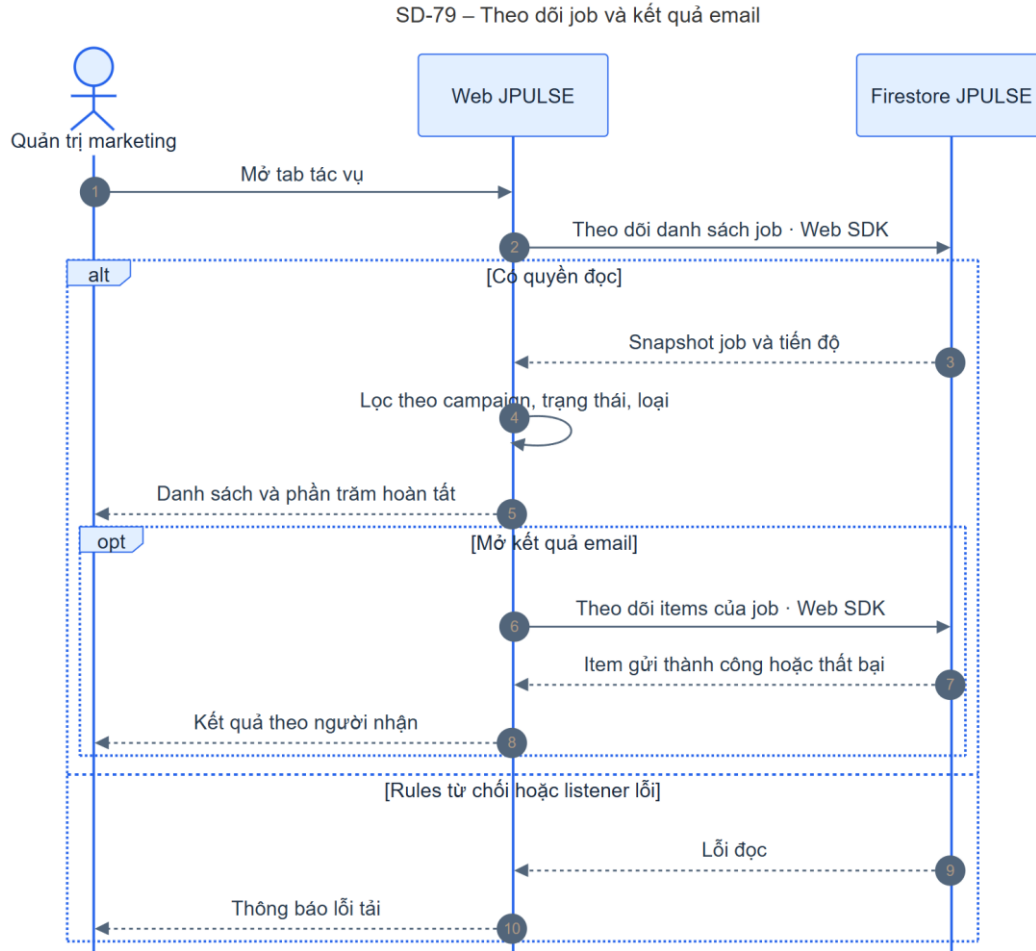
Hình 4-96: SD-79 theo dõi job và kết quả email
