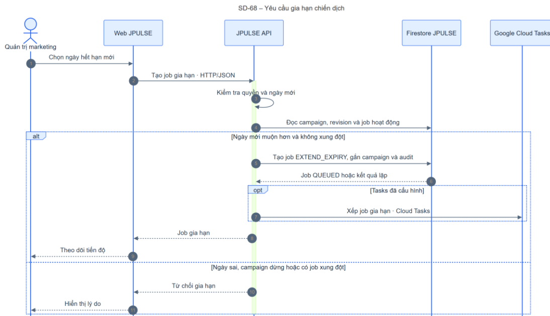
Hình 4-85: SD-68 yêu cầu gia hạn chiến dịch
