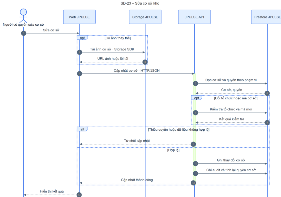
Hình 4-55: SD-23 sửa cơ sở kho
