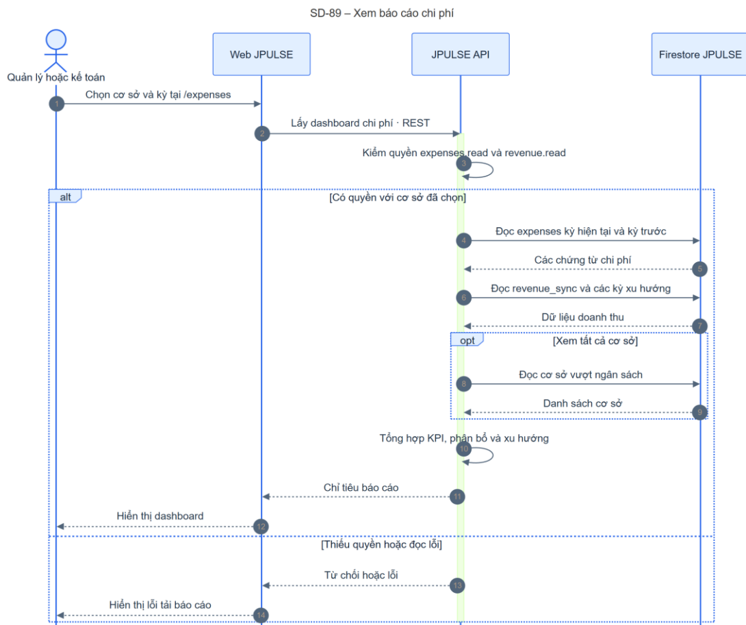
Hình 4-106: SD-89 xem báo cáo chi phí
