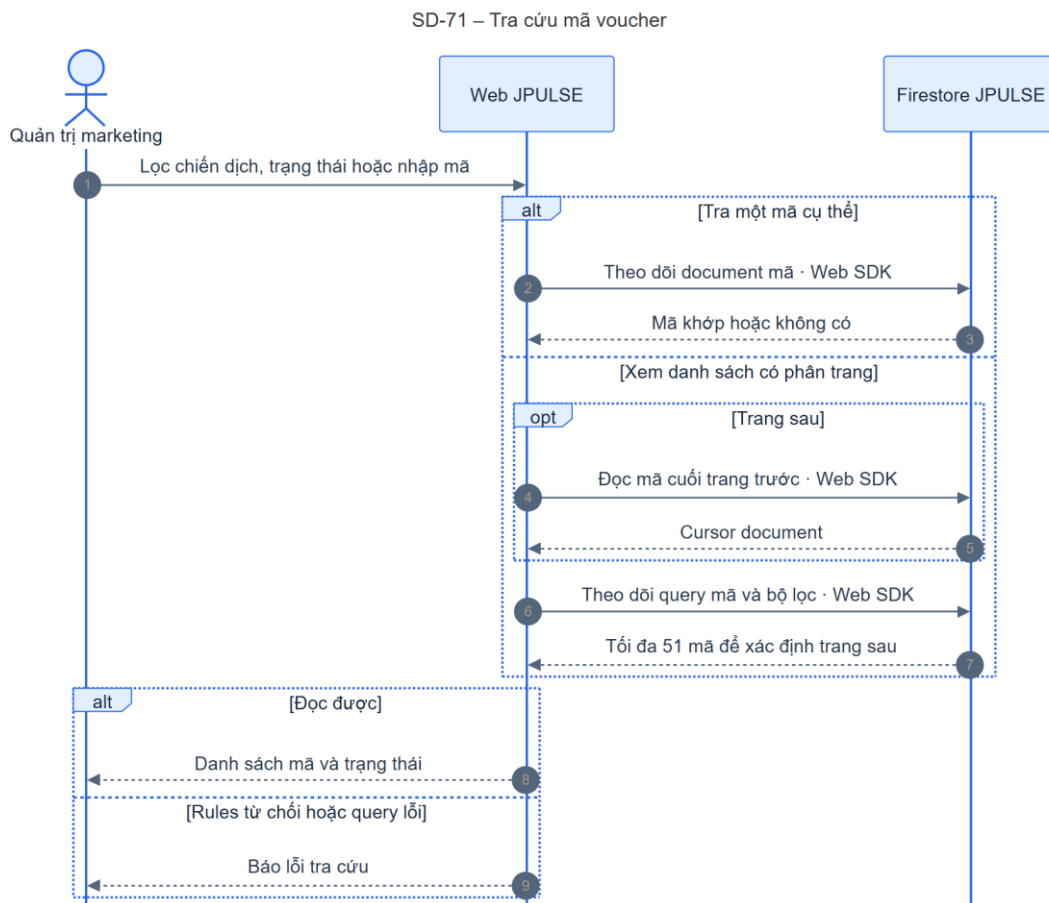
Hình 4-88: SD-71 tra cứu mã voucher
