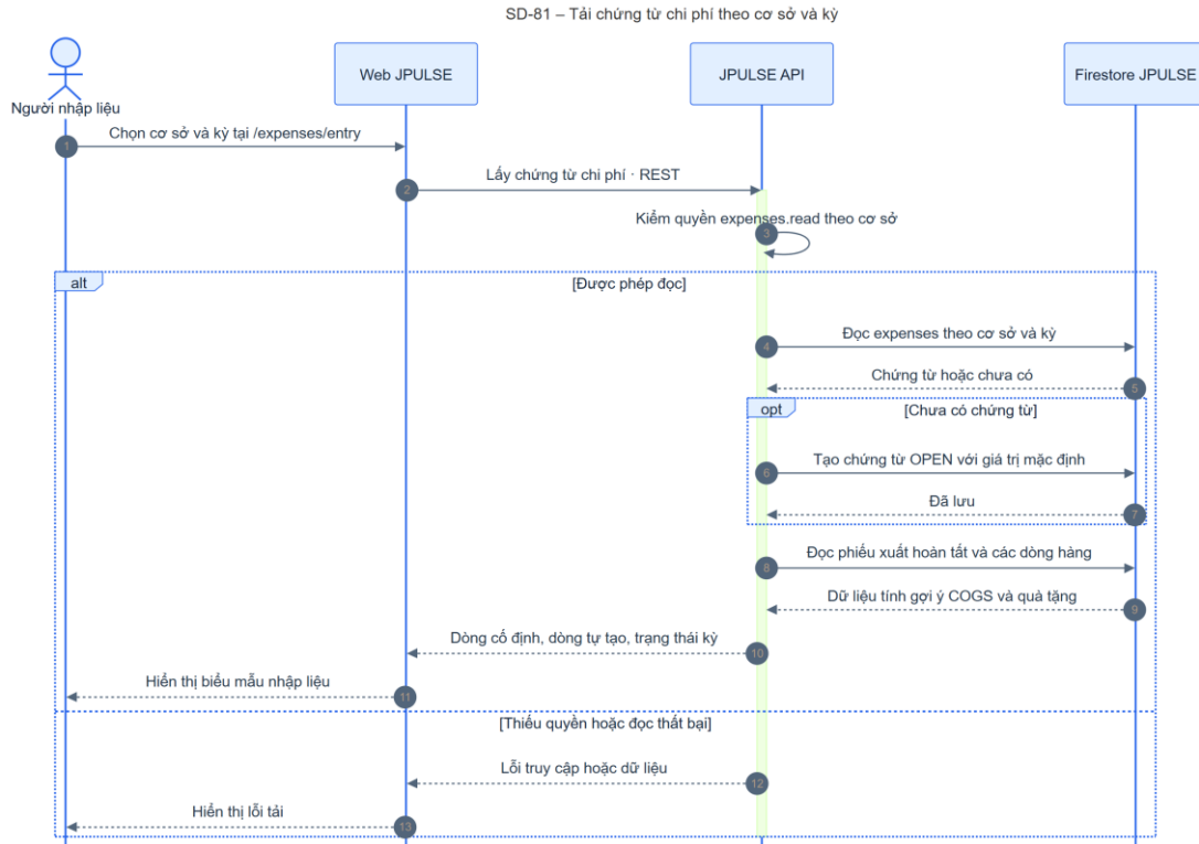
Hình 4-98: SD-81 tải chứng từ chi phí
