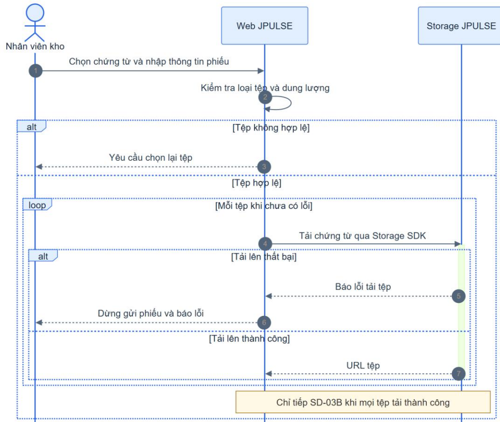
Hình 4-7: SD-03A tải chứng từ phiếu nhập
