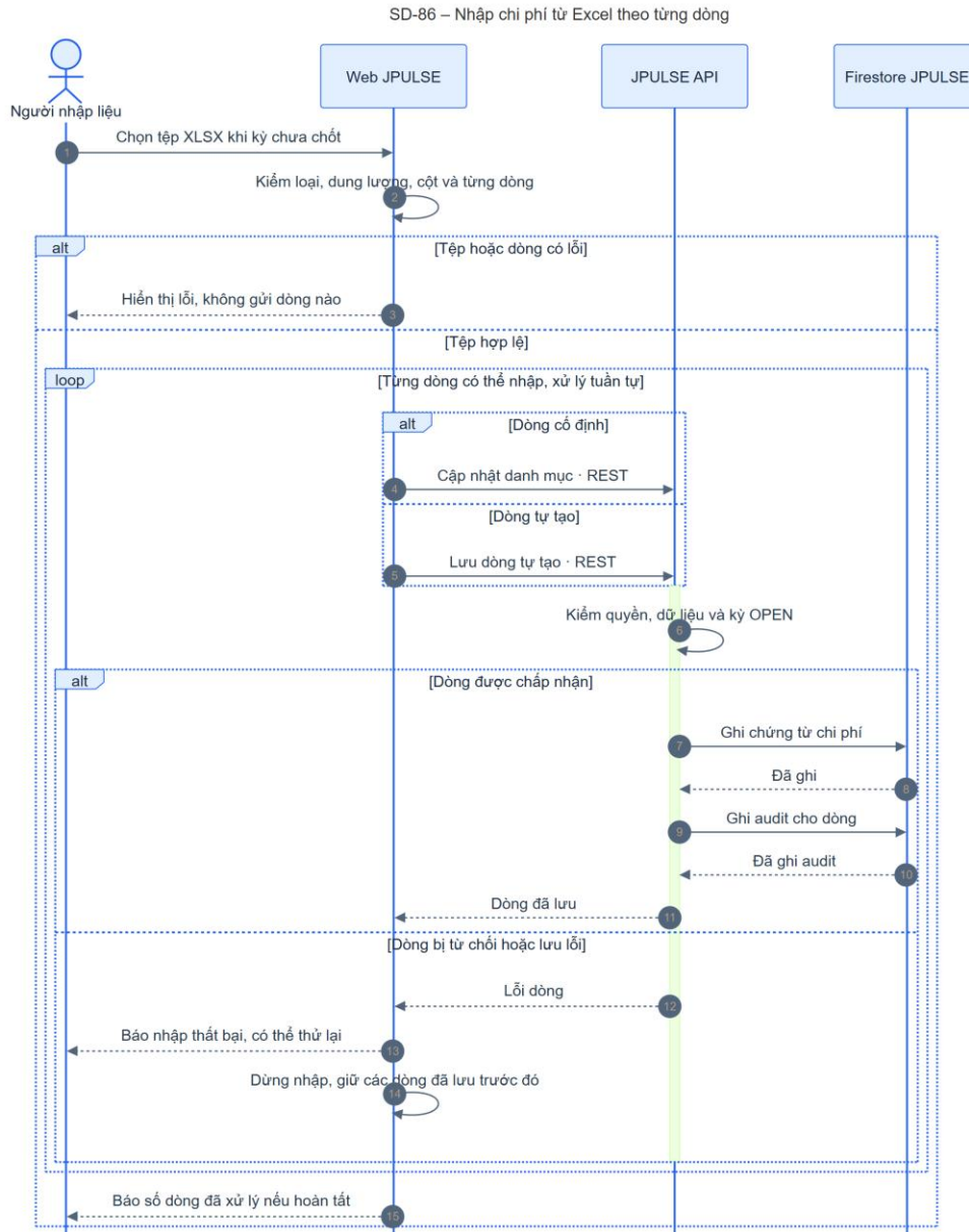
Hình 4-103: SD-86 nhập Excel
