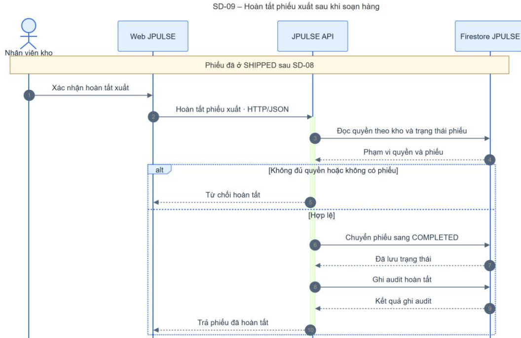
Hình 4-14: SD-09 hoàn tất phiếu xuất
