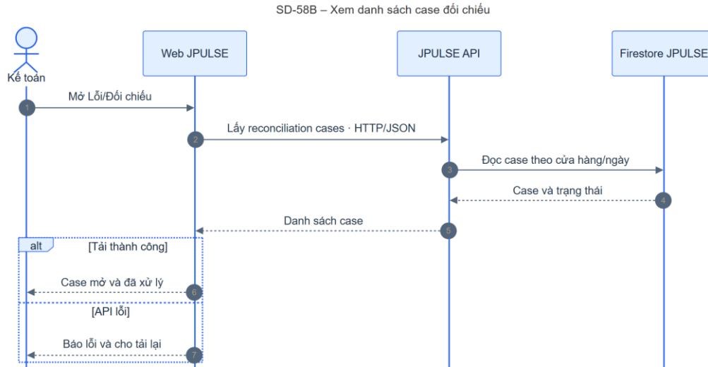
Hình 4-45: SD-58B xem danh sách case đối chiếu
