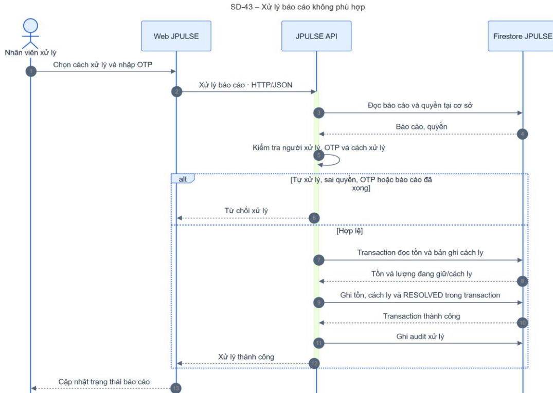
Hình 4-75: SD-43 xử lý báo cáo không phù hợp
