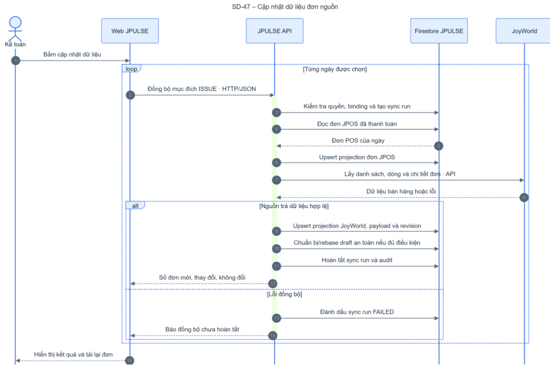
Hình 4-32: SD-47 cập nhật dữ liệu đơn nguồn
