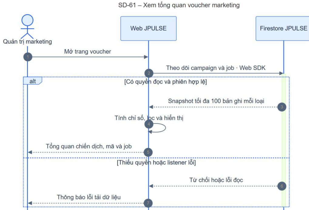
Hình 4-78: SD-61 xem tổng quan voucher marketing
