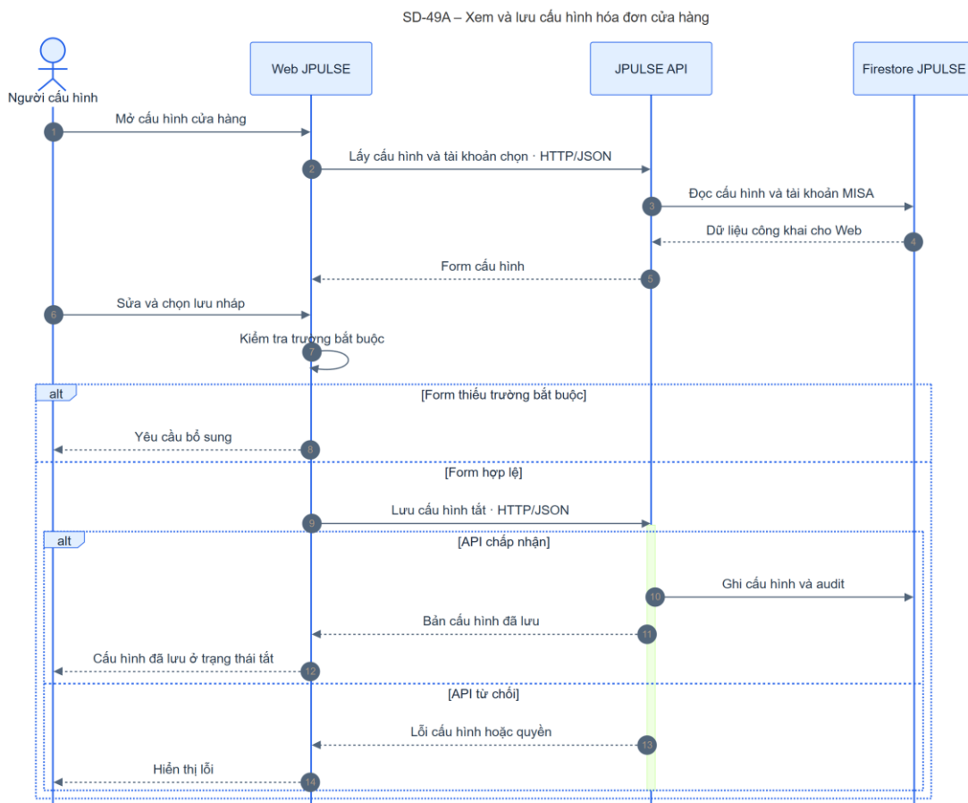
Hình 4-34: SD-49A xem và lưu cấu hình hóa đơn cửa hàng
