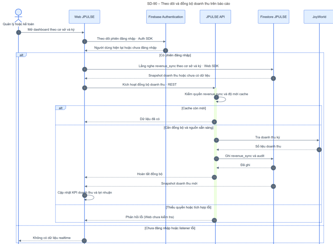
Hình 4-107: SD-90 đồng bộ doanh thu
