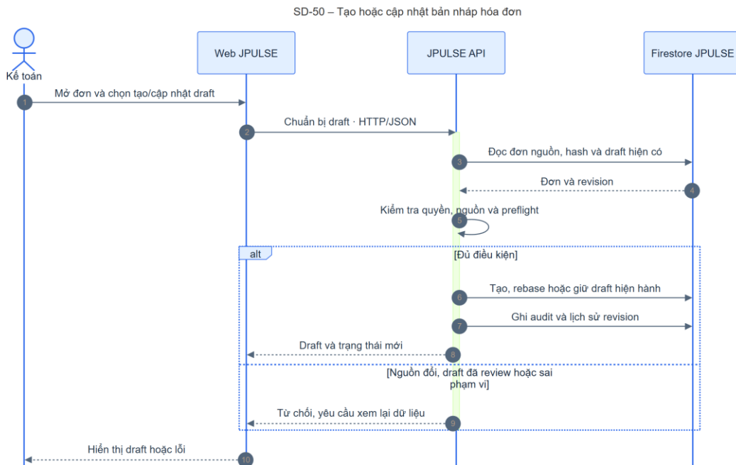
Hình 4-36: SD-50 tạo hoặc cập nhật bản nháp hóa đơn
