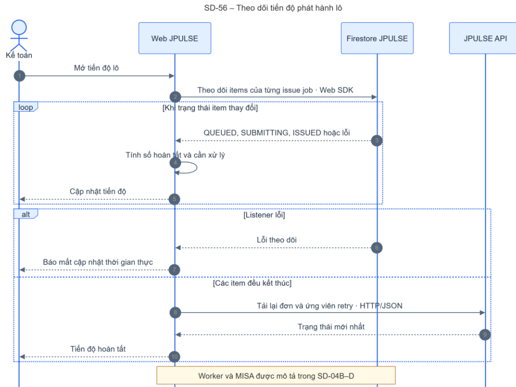
Hình 4-42: SD-56 theo dõi tiến độ phát hành lô
