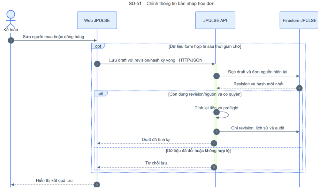
Hình 4-37: SD-51 chỉnh thông tin bản nháp hóa đơn
