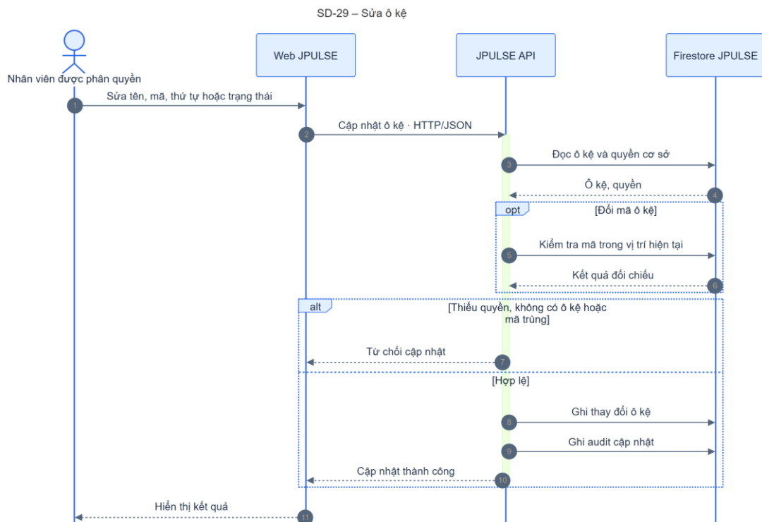
Hình 4-61: SD-29 sửa ô kê
