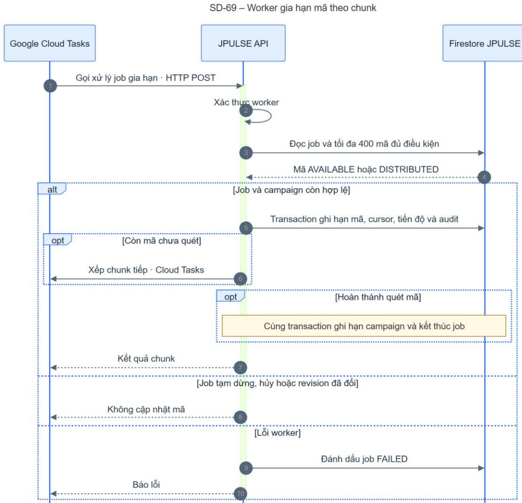
Hình 4-86: SD-69 worker gia hạn mã theo chunk
