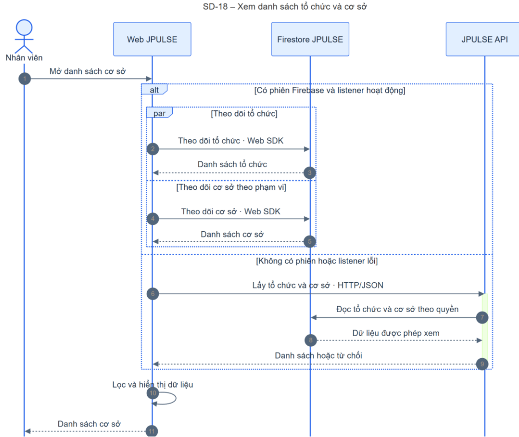
Hình 4-50: SD-18 xem danh sách tổ chức và cơ sở
