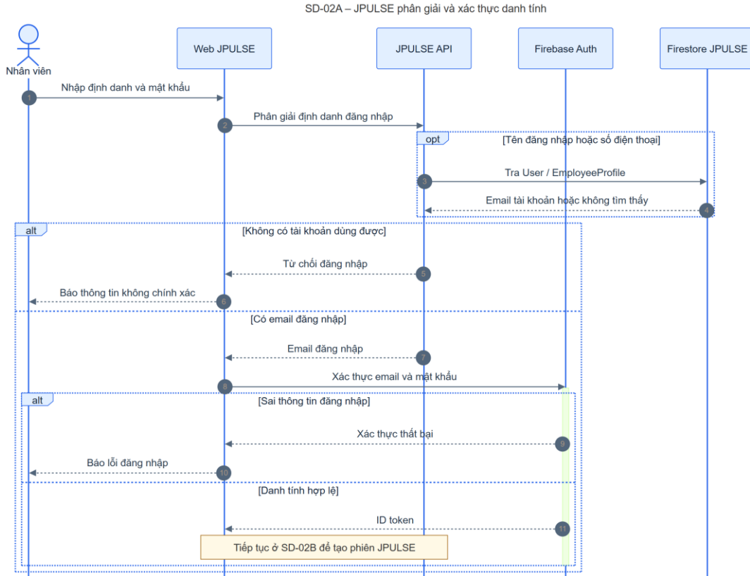
Hình 4-4: SD-02A jPULSE xác thực danh tính
