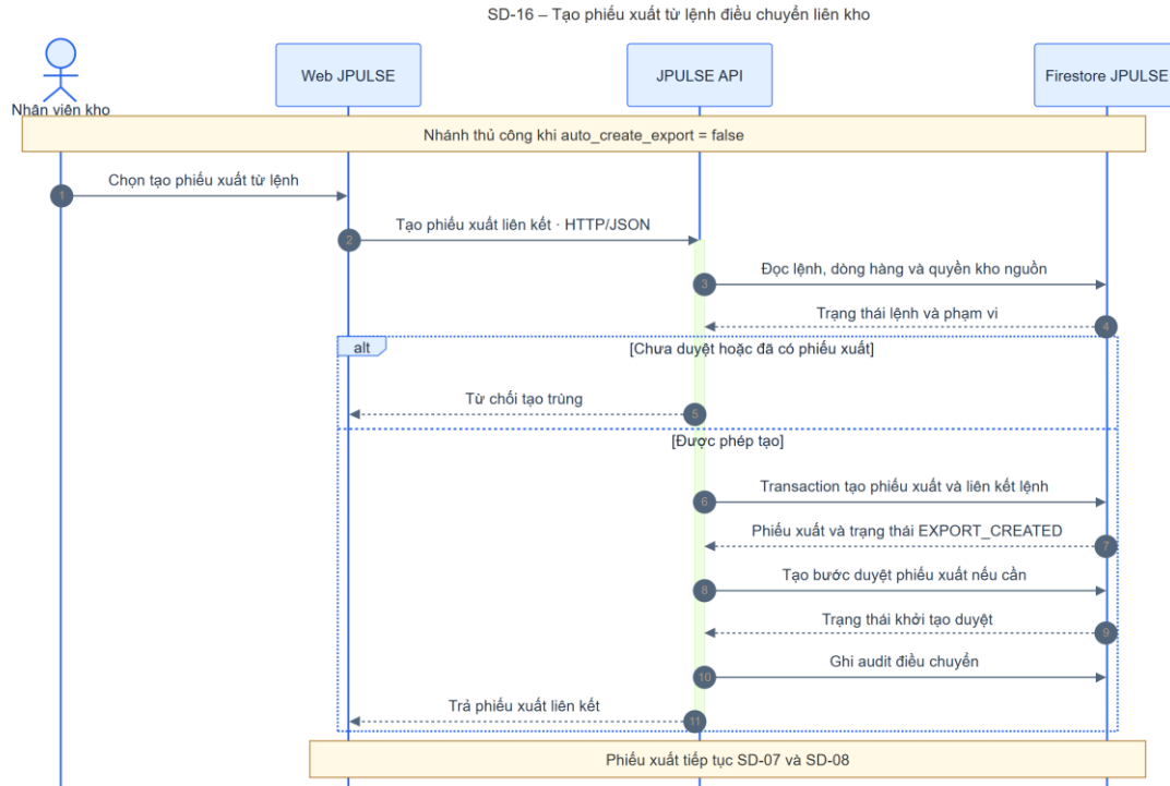
Hình 4-22: SD-16 tạo phiếu xuất từ lệnh điều chuyển
