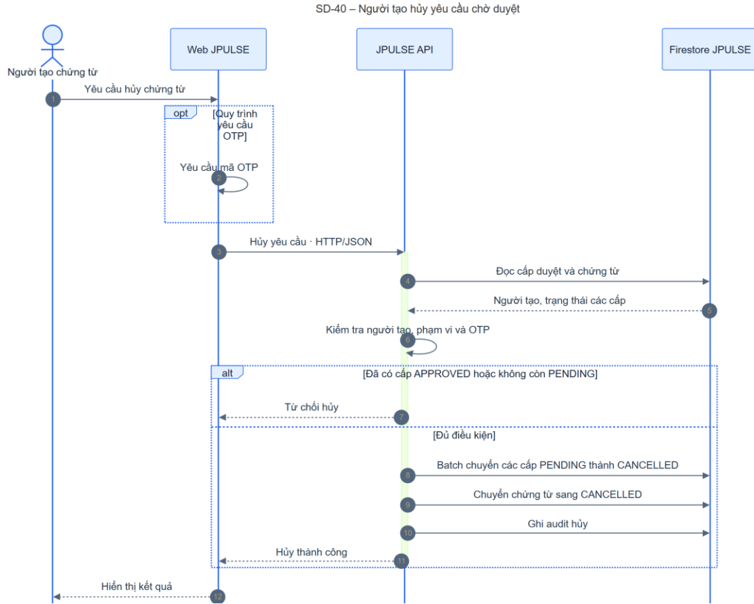
Hình 4-72: SD-40 người tạo hủy yêu cầu chờ duyệt
