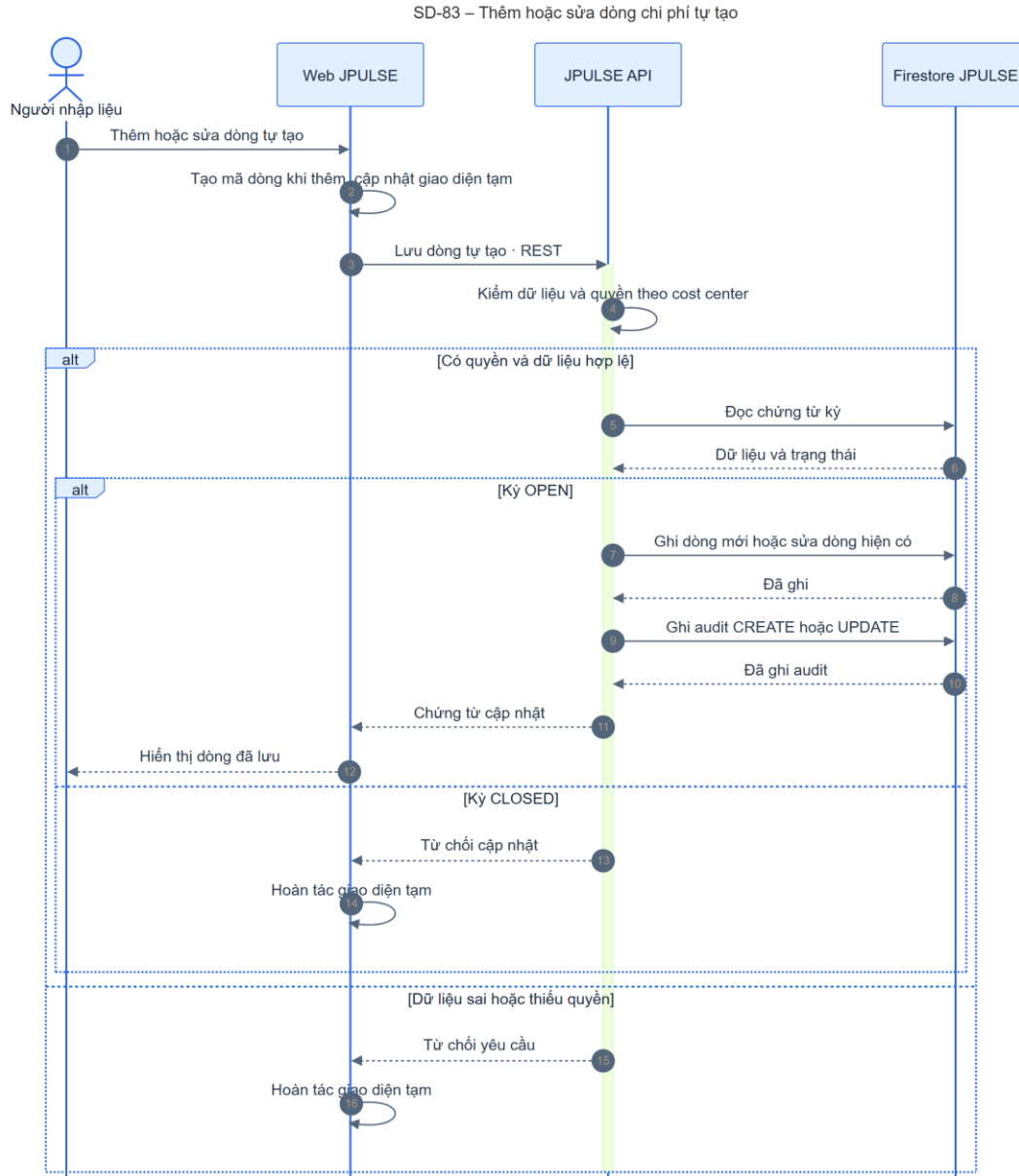
Hình 4-100: SD-83 lưu dòng tự tạo
