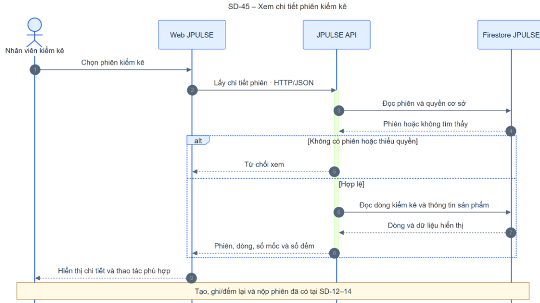
Hình 4-77: SD-45 xem chi tiết phiên kiểm kê
