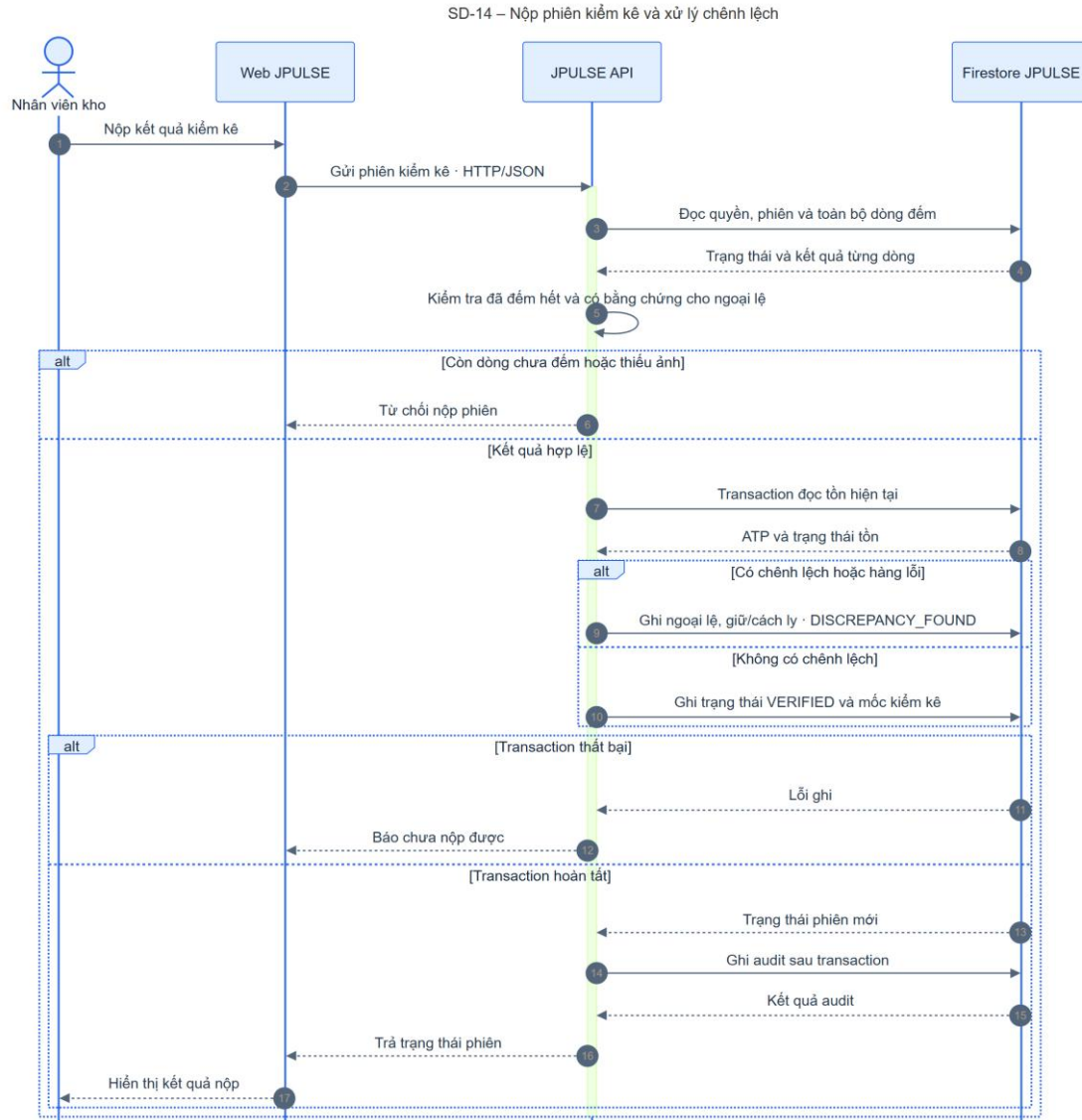
Hình 4-20: SD-14 nộp phiên kiểm kê
