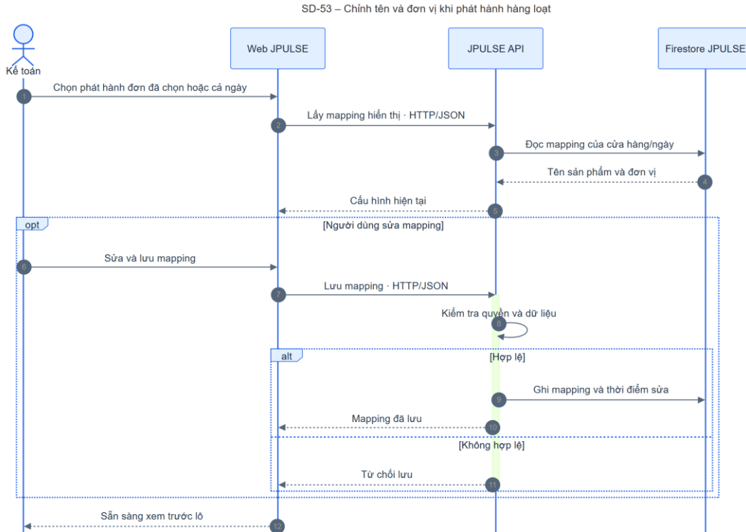
Hình 4-39: SD-53 chỉnh tên và đơn vị khi phát hành hàng loạt
