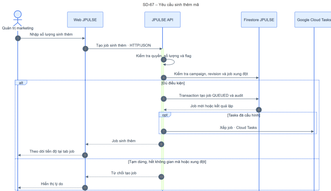
Hình 4-84: SD-67 yêu cầu sinh thêm mã
