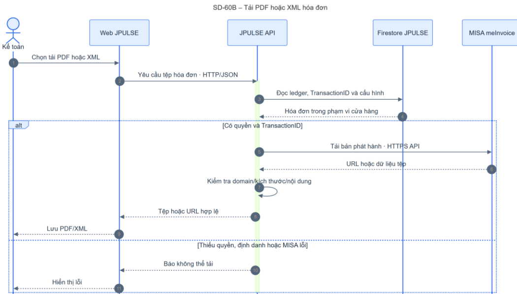
Hình 4-48: SD-60B tải PDF hoặc XML hóa đơn
