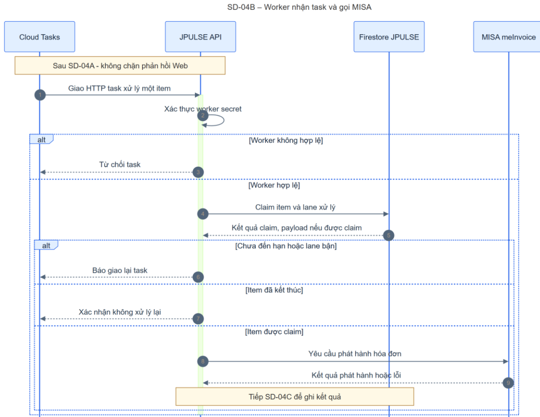
Hình 4-28: SD-04B worker nhận task và gọi MISA
