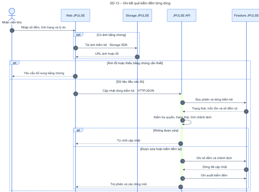
Hình 4-19: SD-13 ghi dòng kiểm kê
