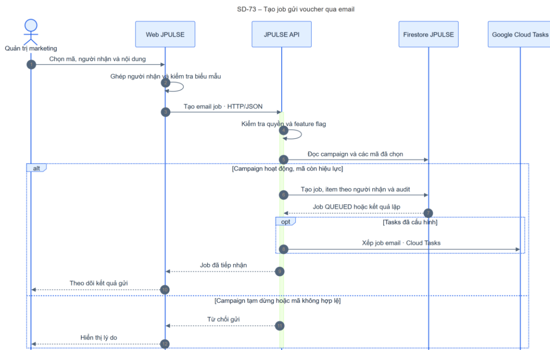
Hình 4-90: SD-73 tạo job gửi voucher qua email
