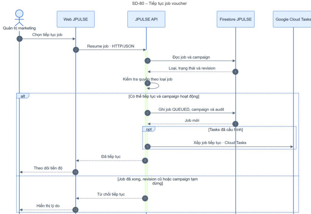
Hình 4-97: SD-80 tiếp tục job voucher
