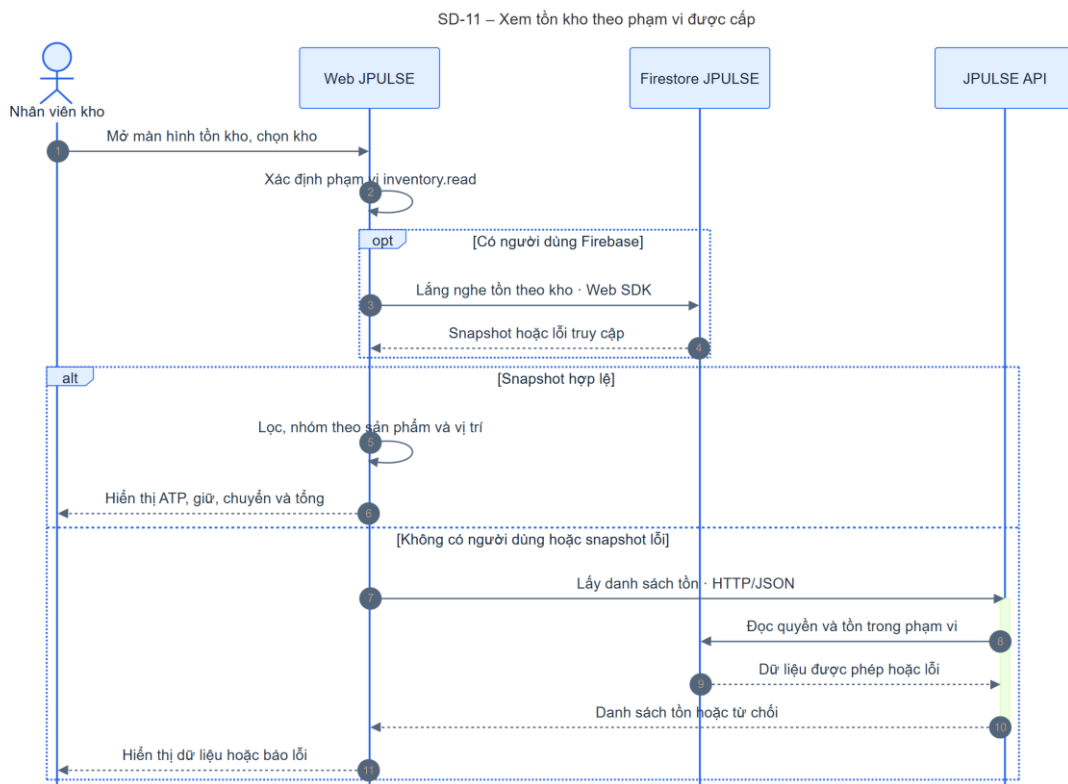
Hình 4-17: SD-11 xem tồn kho
