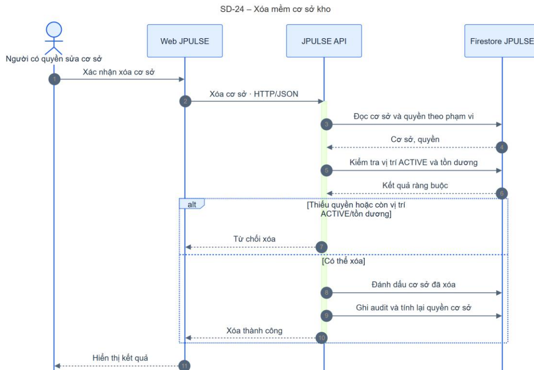
Hình 4-56: SD-24 xóa mềm cơ sở kho
