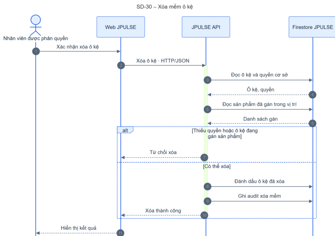
Hình 4-62: SD-30 xóa mềm ô kê
