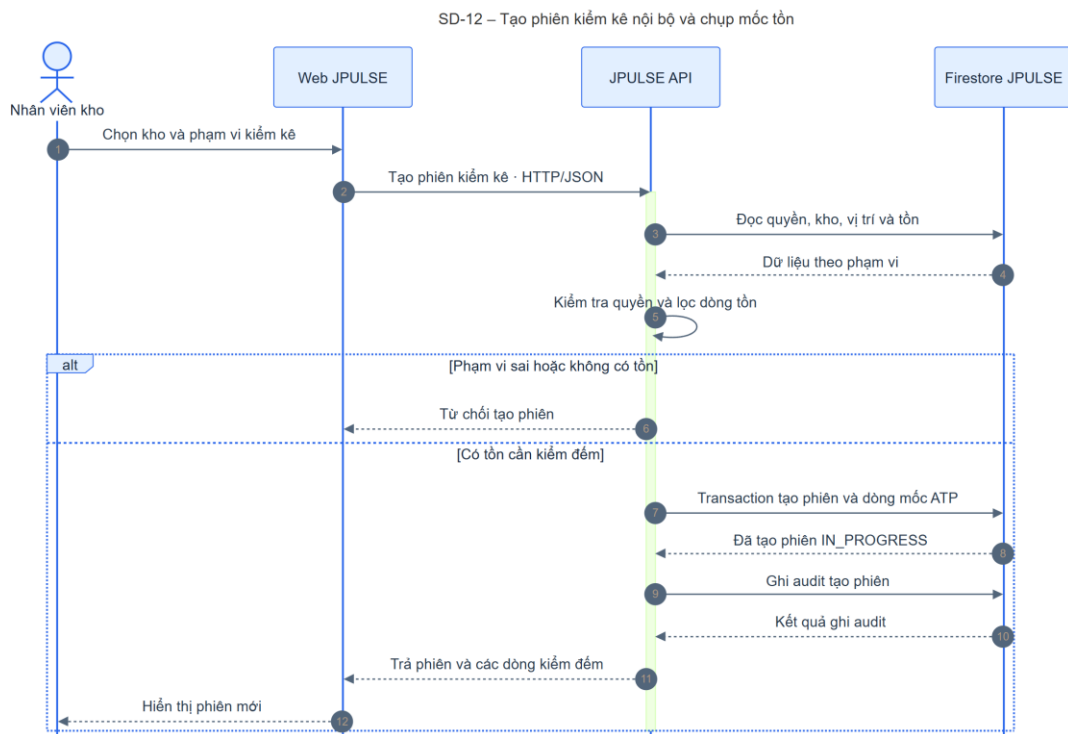
Hình 4-18: SD-12 tạo phiên kiểm kê
