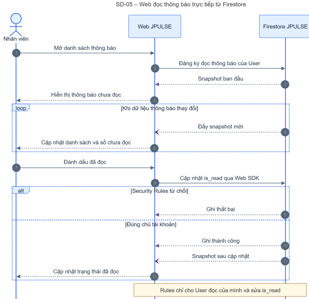
Hình 4-49: SD-05 thông báo realtime
