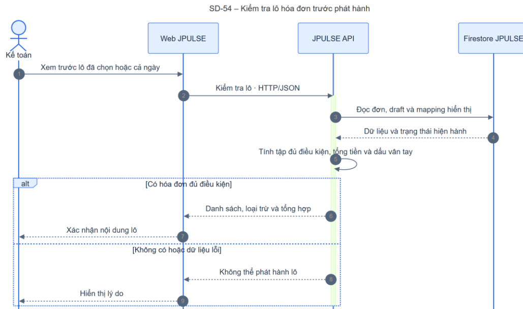
Hình 4-40: SD-54 kiểm tra lô hóa đơn trước phát hành
