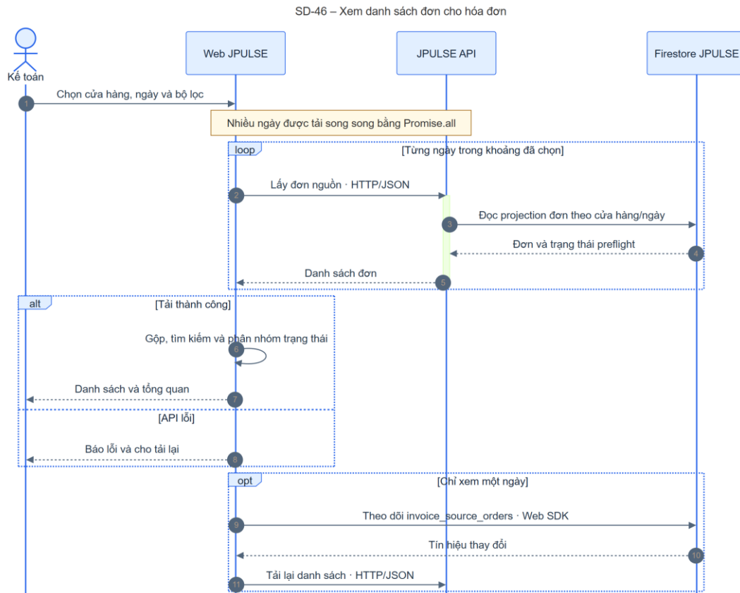
Hình 4-31: SD-46 xem danh sách đơn cho hóa đơn
