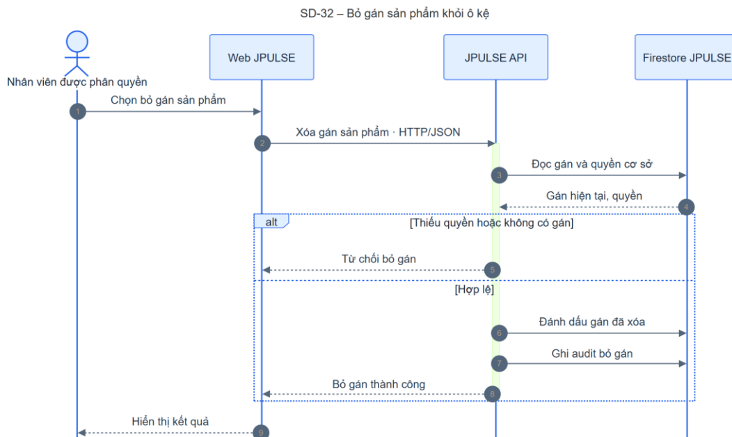
Hình 4-64: SD-32 bỏ gán sản phẩm khỏi ô kệ
