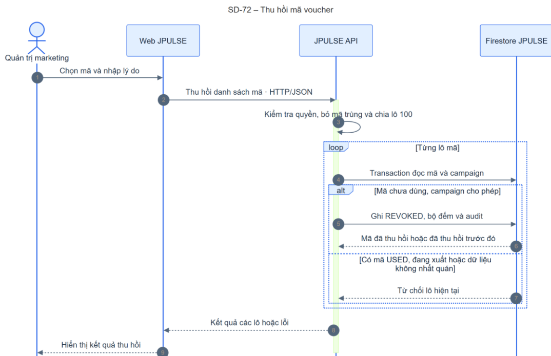
Hình 4-89: SD-72 thu hồi mã voucher
