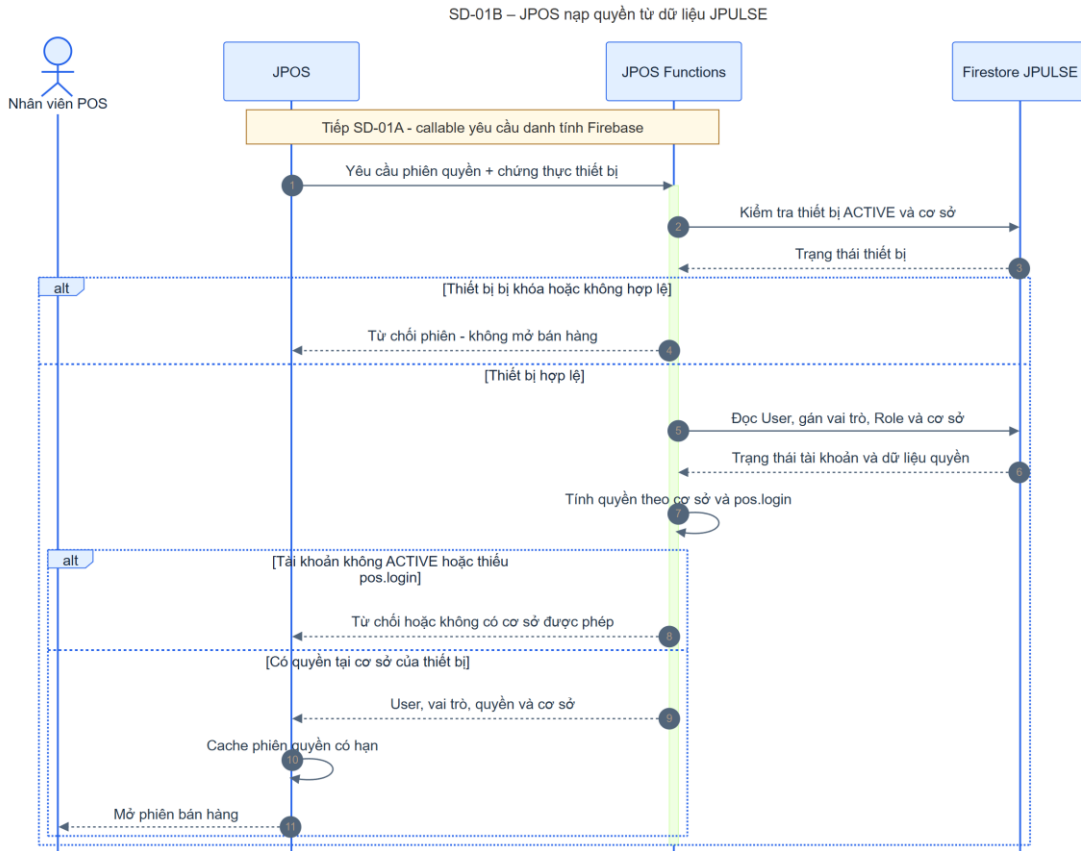
Hình 4-25: SD-01B JPOS nạp quyền từ dữ liệu JPULSE
