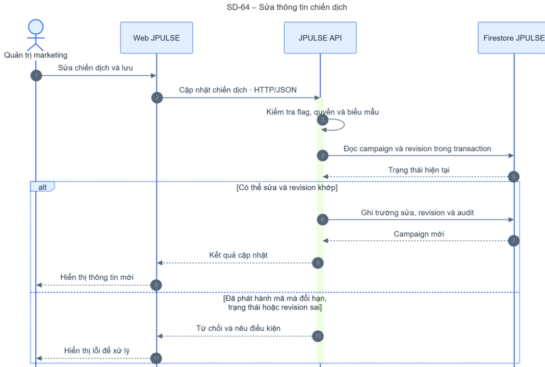
Hình 4-81: SD-64 sửa thông tin chiến dịch
