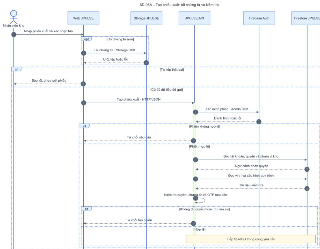
Hình 4-10: SD-06A kiểm tra phiếu xuất
