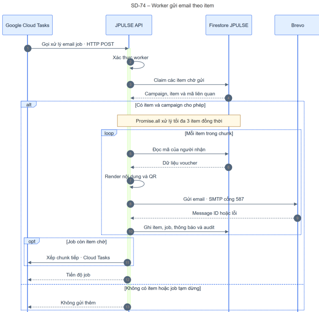
Hình 4-91: SD-74 worker gửi email theo item
