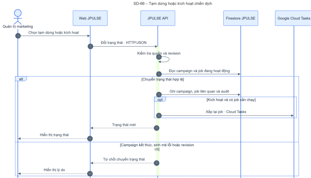
Hình 4-83: SD-66 tạm dừng hoặc kích hoạt chiến dịch
