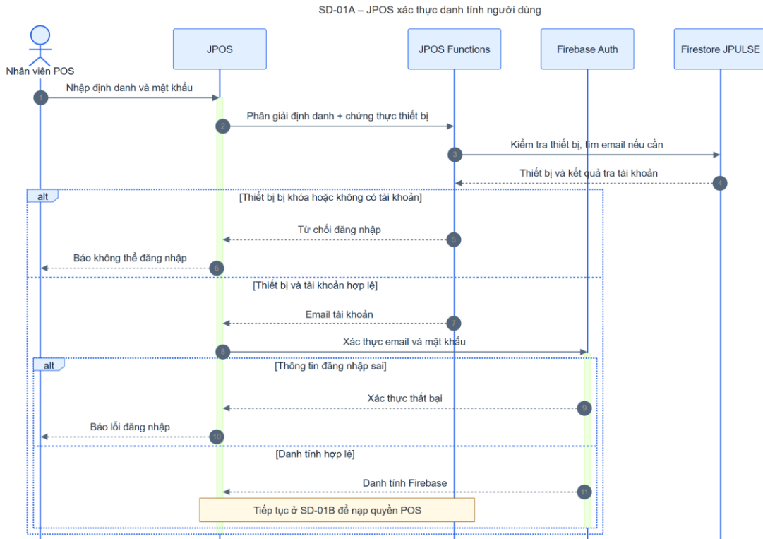
Hình 4-24: SD-01A jPOS xác thực danh tính
