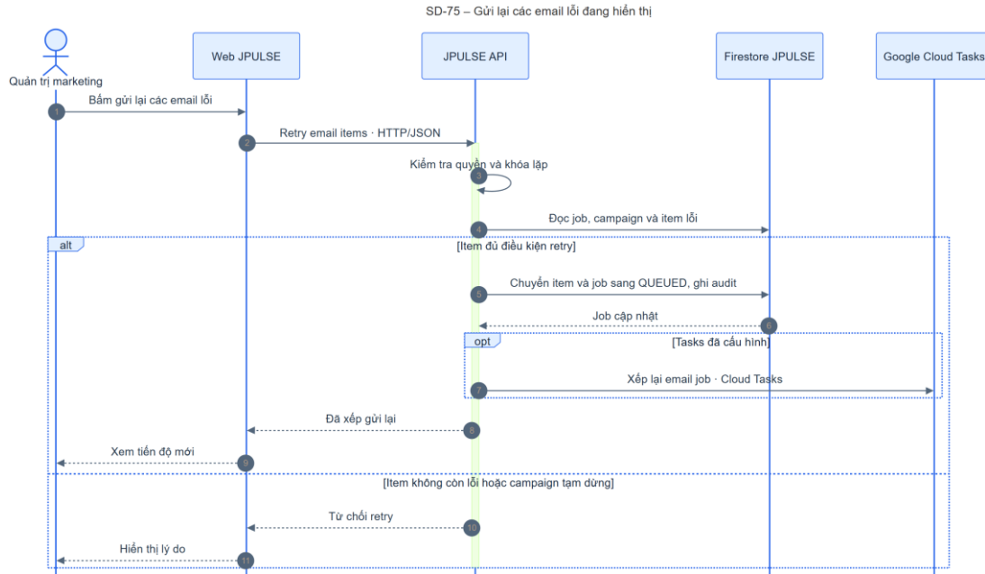
Hình 4-92: SD-75 gửi lại các email lỗi đang hiển thị
