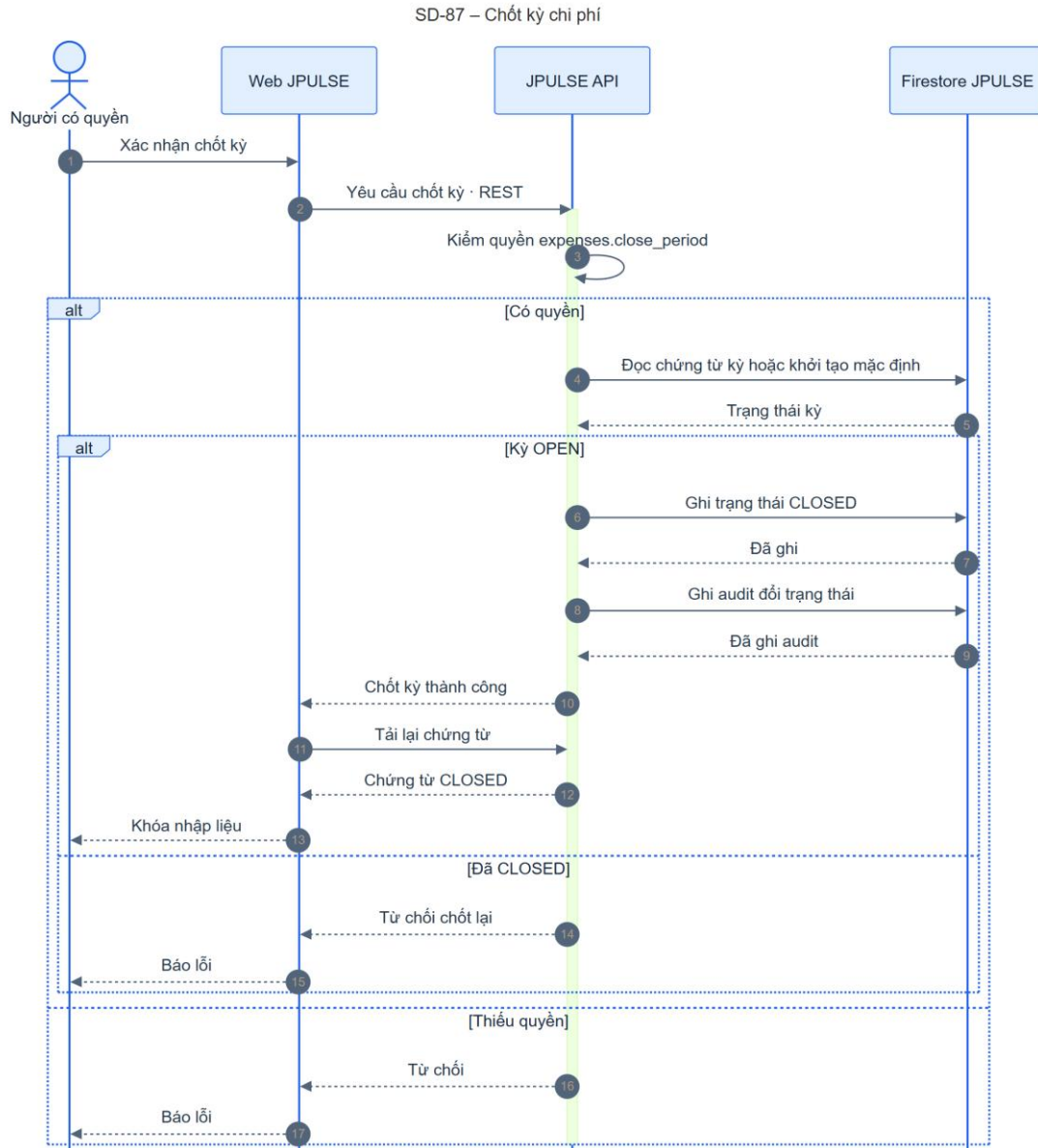
Hình 4-104: SD-87 chốt kỳ
