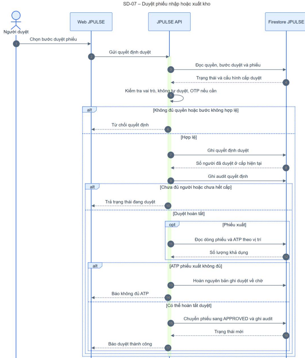
Hình 4-12: SD-07 duyệt phiếu kho
