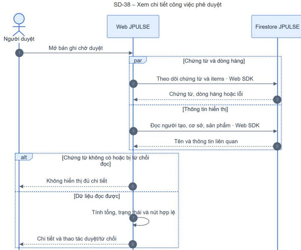
Hình 4-70: SD-38 xem chi tiết công việc phê duyệt
