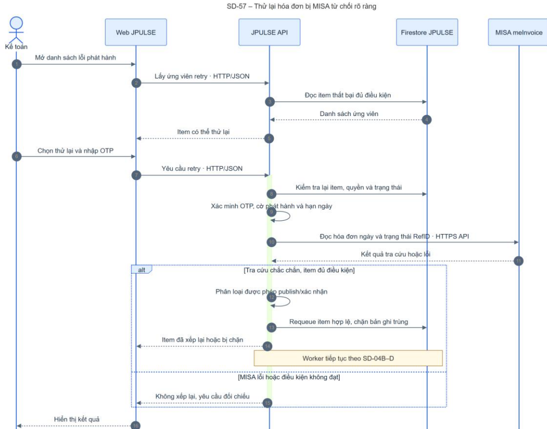
Hình 4-43: SD-57 thử lại hóa đơn bị MISA từ chối rõ ràng
