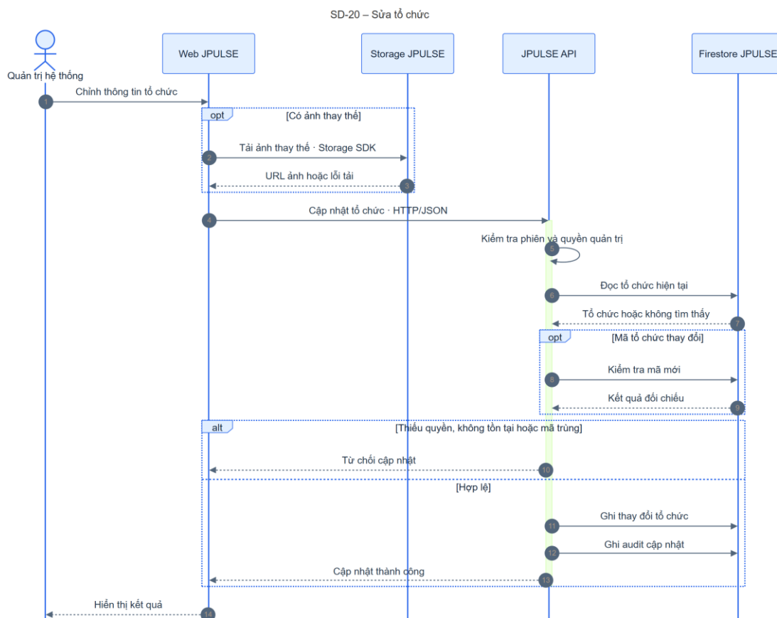
Hình 4-52: SD-20 sửa tổ chức
