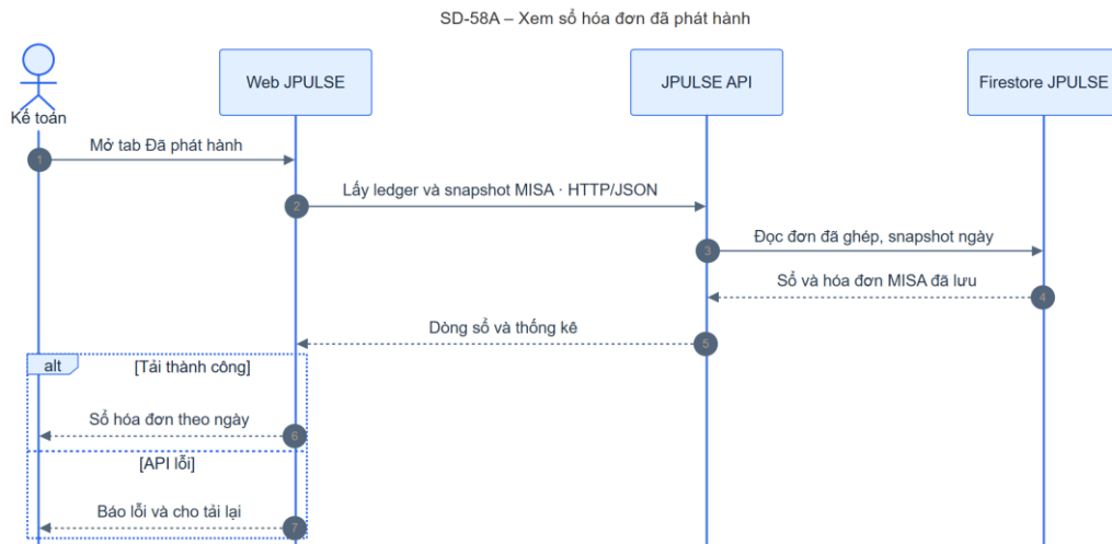
Hình 4-44: SD-58A xem sổ hóa đơn đã phát hành
