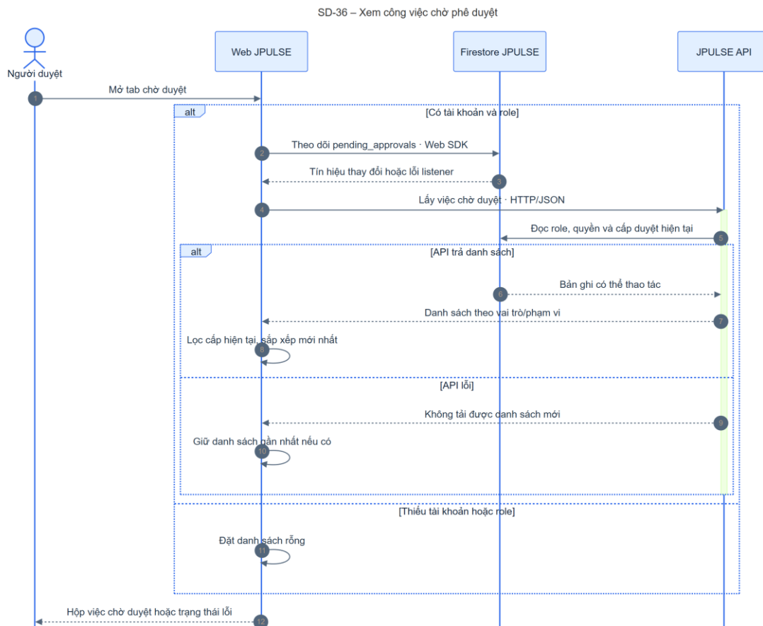
Hình 4-68: SD-36 xem công việc chờ phê duyệt
