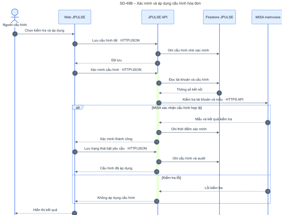
Hình 4-35: SD-49B xác minh và áp dụng cấu hình hóa đơn
