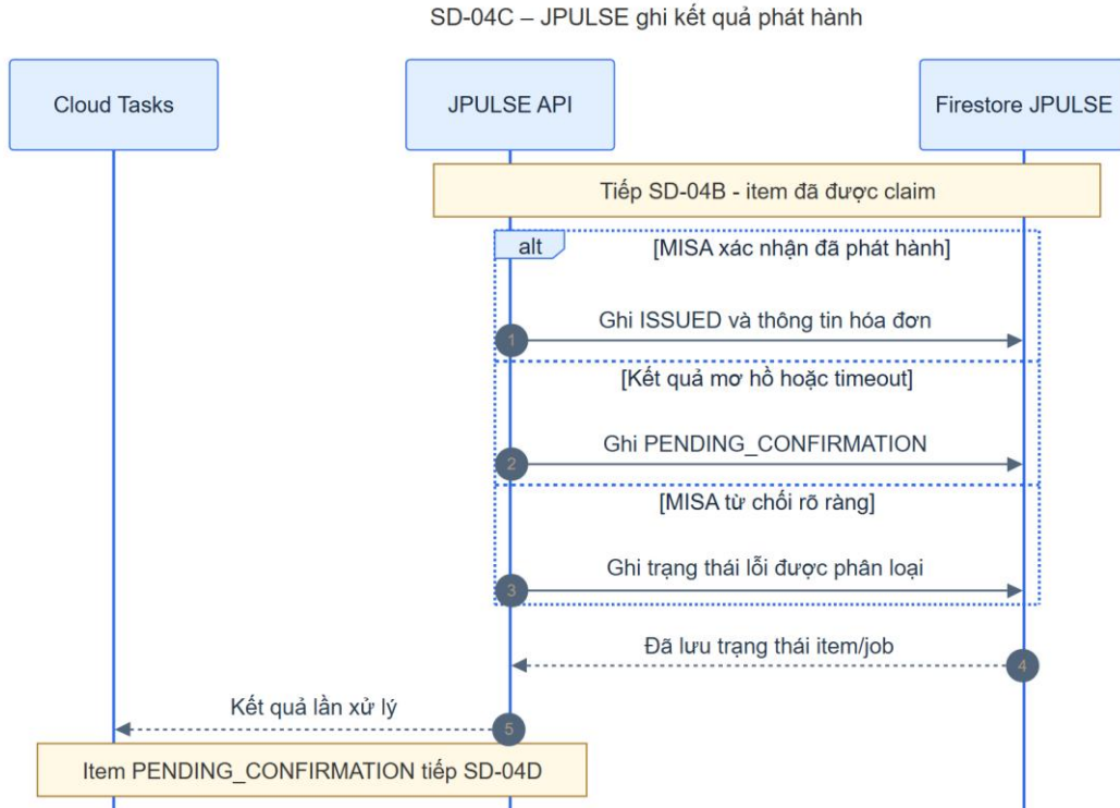
Hình 4-29: SD-04C ghi kết quả phát hành hóa đơn
