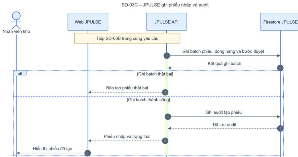
Hình 4-9: SD-03C ghi phiếu nhập và audit
