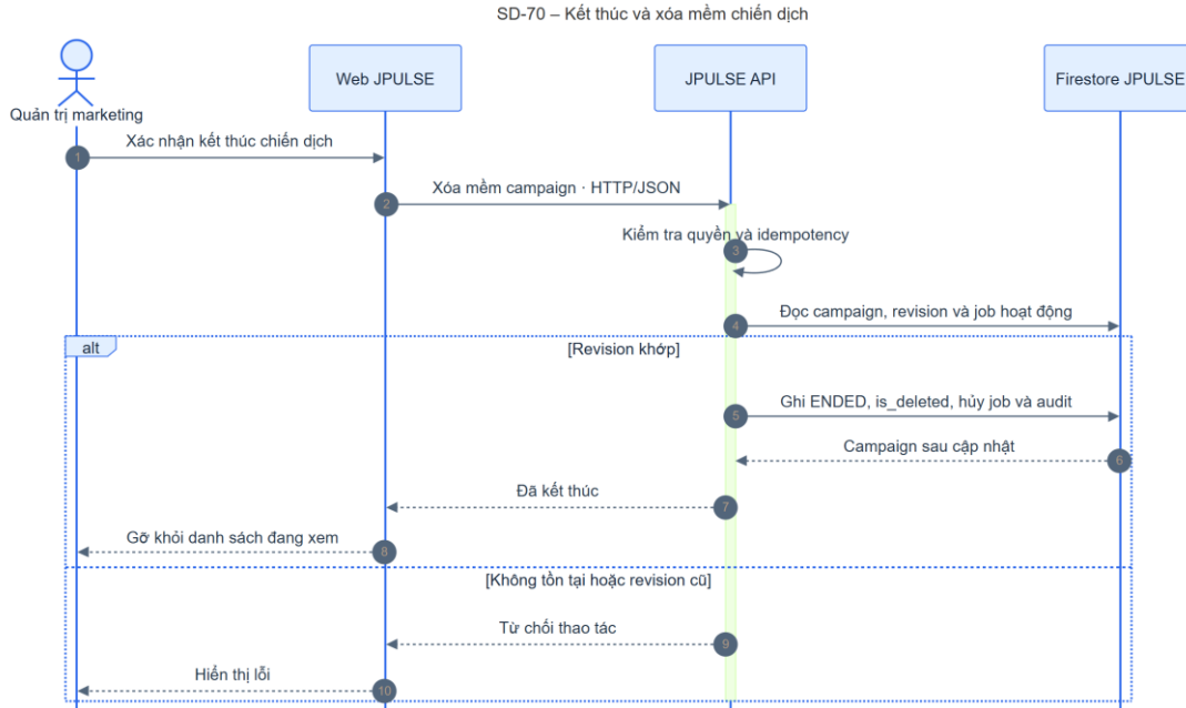
Hình 4-87: SD-70 kết thúc và xóa mềm chiến dịch
