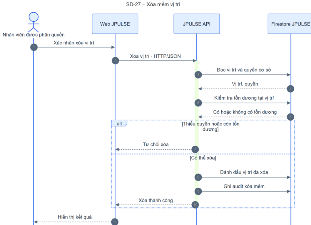
Hình 4-59: SD-27 xóa mềm vị trí
