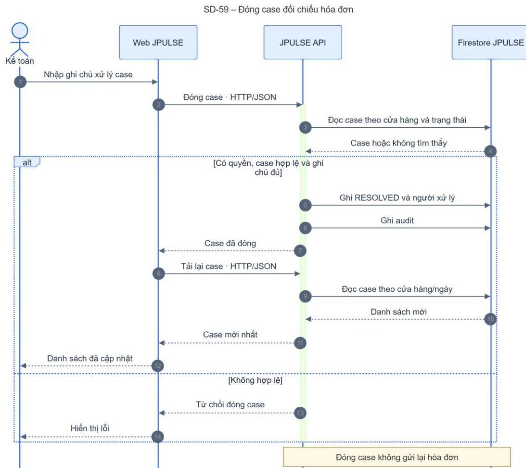
Hình 4-46: SD-59 đóng case đối chiếu hóa đơn
