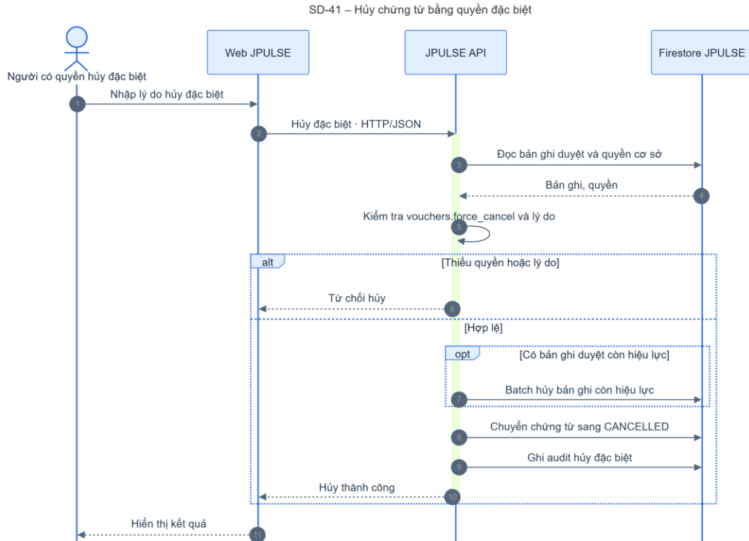
Hình 4-73: SD-41 hủy chứng từ bằng quyền đặc biệt
