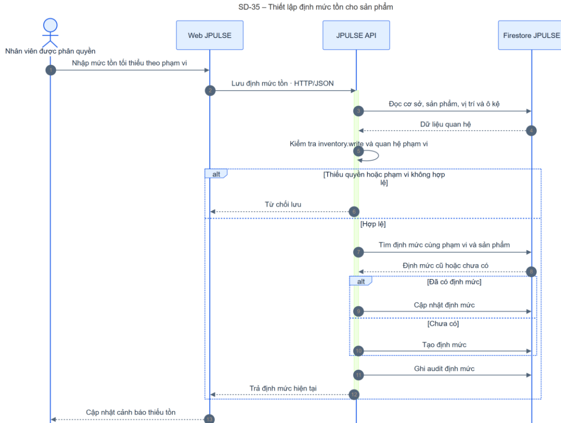
Hình 4-67: SD-35 thiết lập định mức tồn cho sản phẩm
