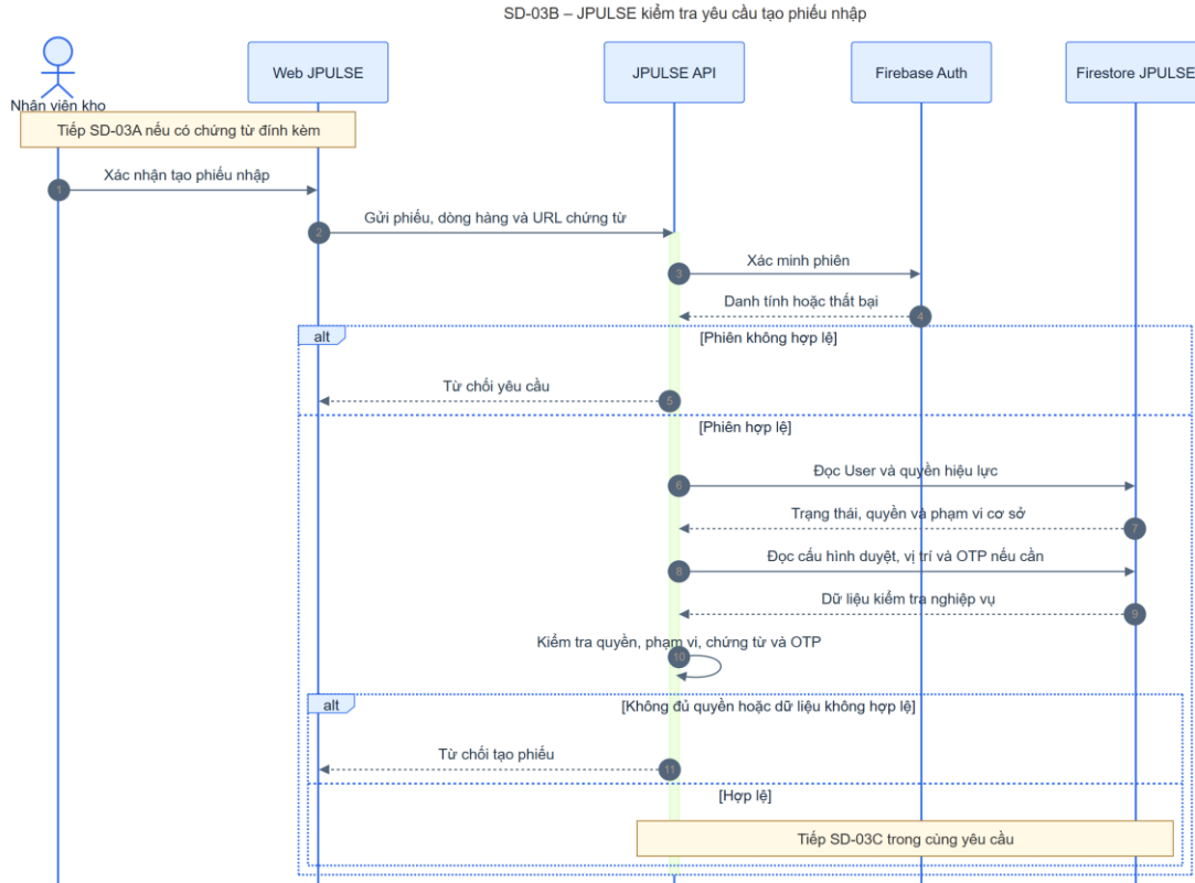
Hình 4-8: SD-03B kiểm tra phiếu nhập
