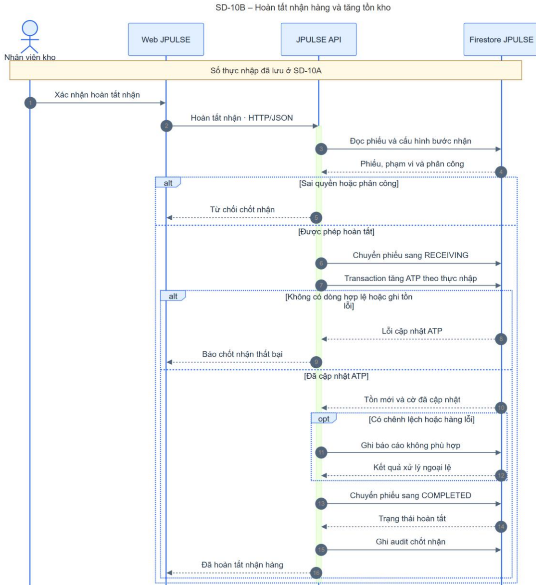
Hình 4-16: SD-10B hoàn tất nhận hàng
