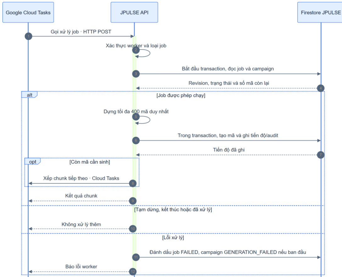
Hình 4-80: SD-63 worker sinh mã voucher
