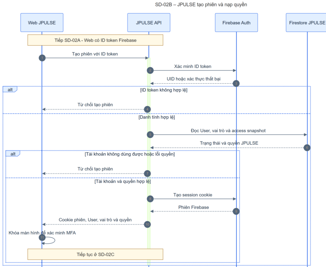
Hình 4-5: SD-02B tạo phiên và nạp quyền JPULSE
