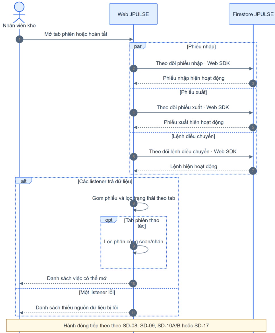
SD-37 – Xem việc soạn, nhận và hoàn tất chứng từ
