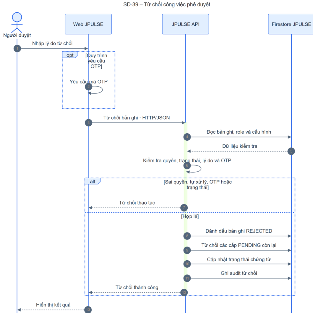
Hình 4-71: SD-39 từ chối công việc phê duyệt
