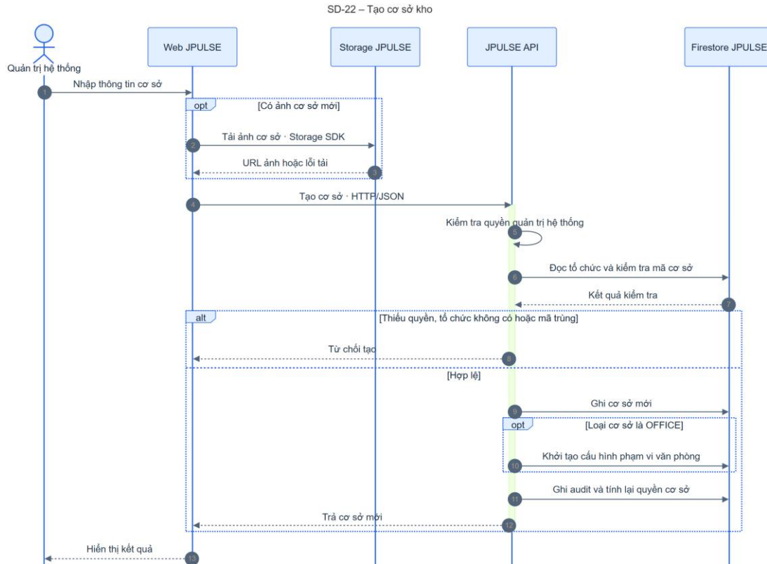
Hình 4-54: SD-22 tạo cơ sở kho
