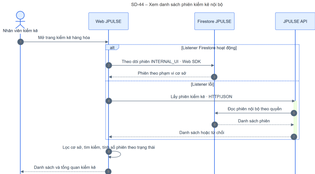
Hình 4-76: SD-44 xem danh sách phiên kiểm kê nội bộ
