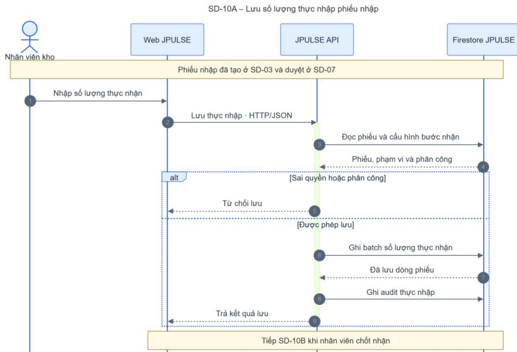
Hình 4-15: SD-10A lưu số thực nhập
