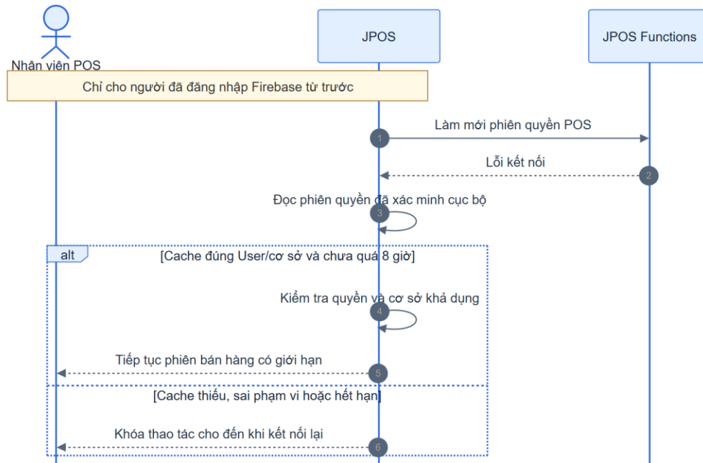
Hình 4-26: SD-01C jPOS khôi phục phiên quyền
