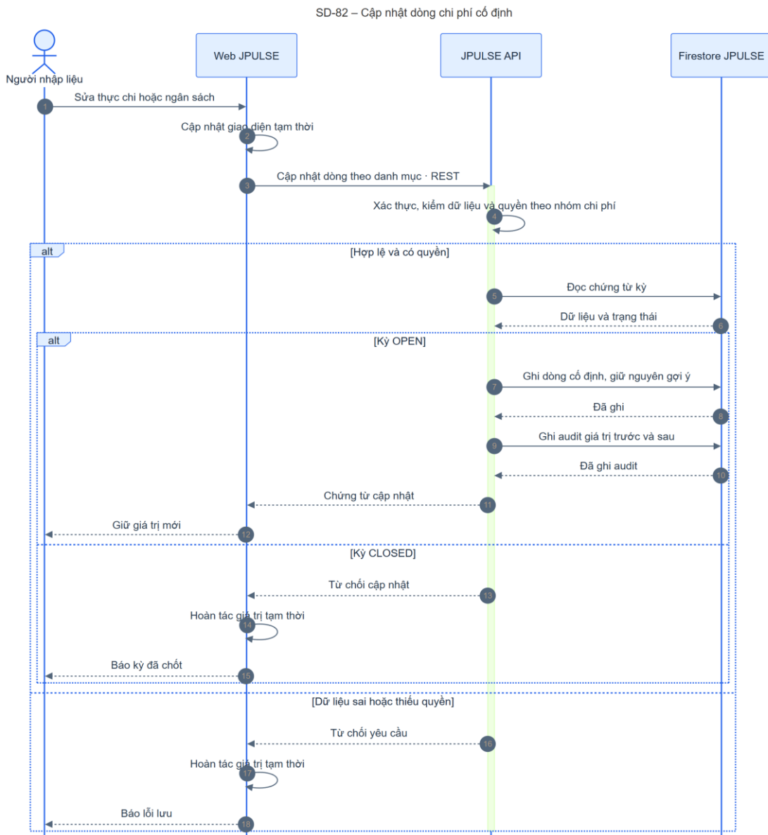
Hình 4-99: SD-82 cập nhật dòng cố định
