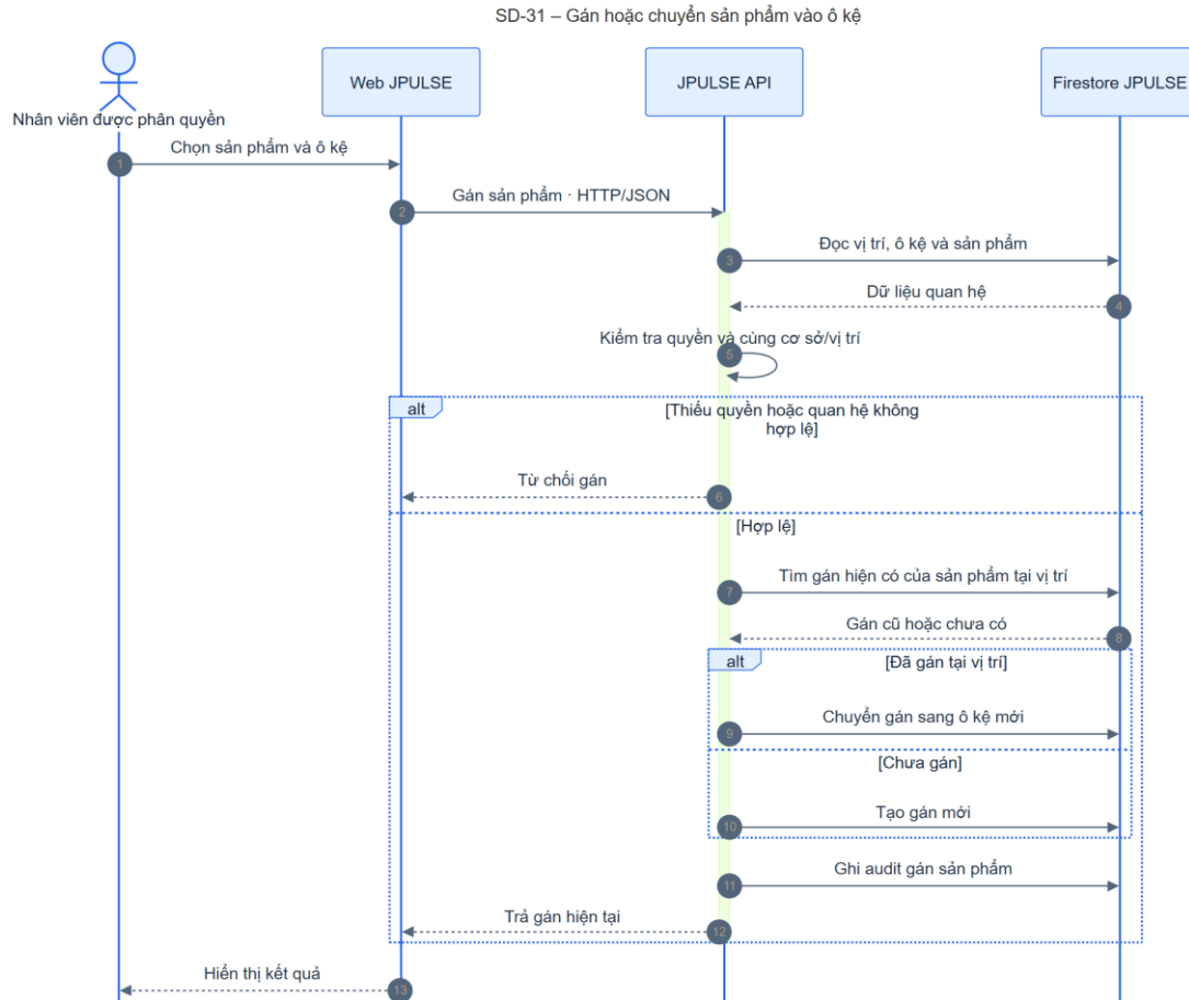
Hình 4-63: SD-31 gán hoặc chuyển sản phẩm vào ô kệ
