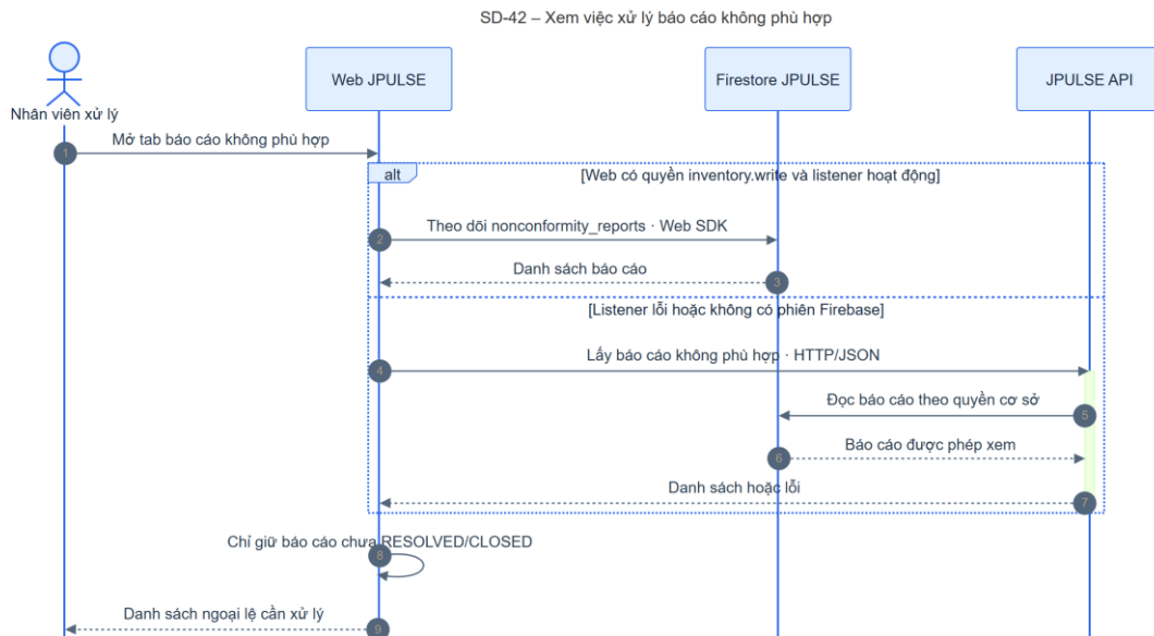
Hình 4-74: SD-42 xem việc xử lý báo cáo không phù hợp
