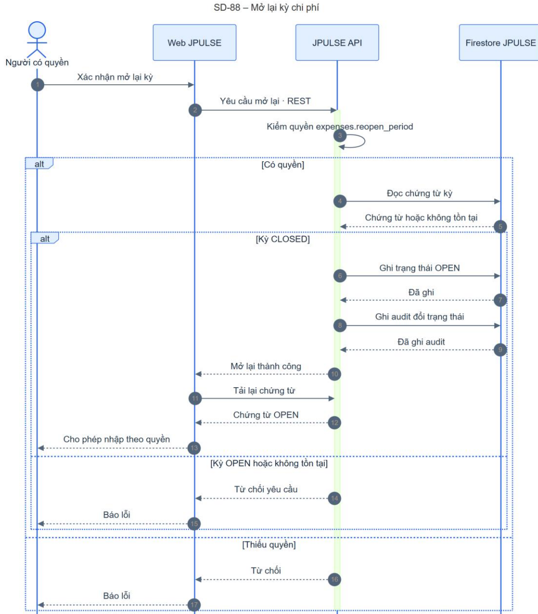
Hình 4-105: SD-88 mở lại kỳ
