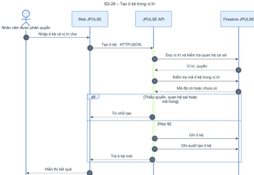
Hình 4-60: SD-28 tạo ô kê trong vị trí
