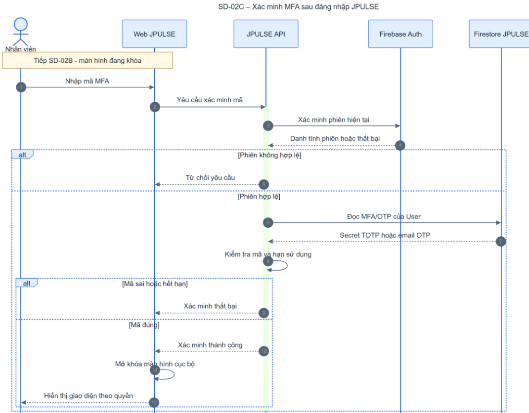
Hình 4-6: SD-02C xác minh MFA sau đăng nhập
