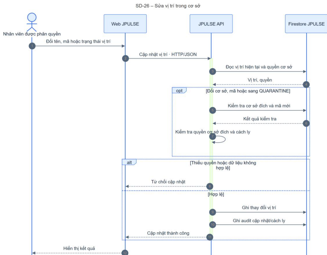
Hình 4-58: SD-26 sửa vị trí trong cơ sở
