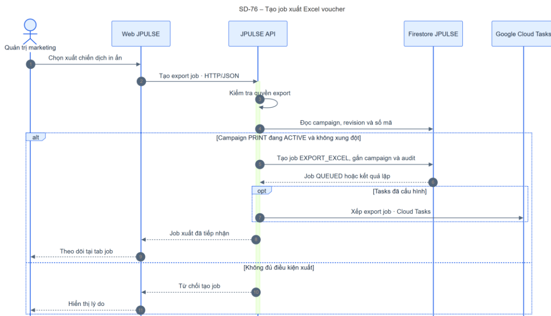
Hình 4-93: SD-76 tạo job xuất Excel voucher
