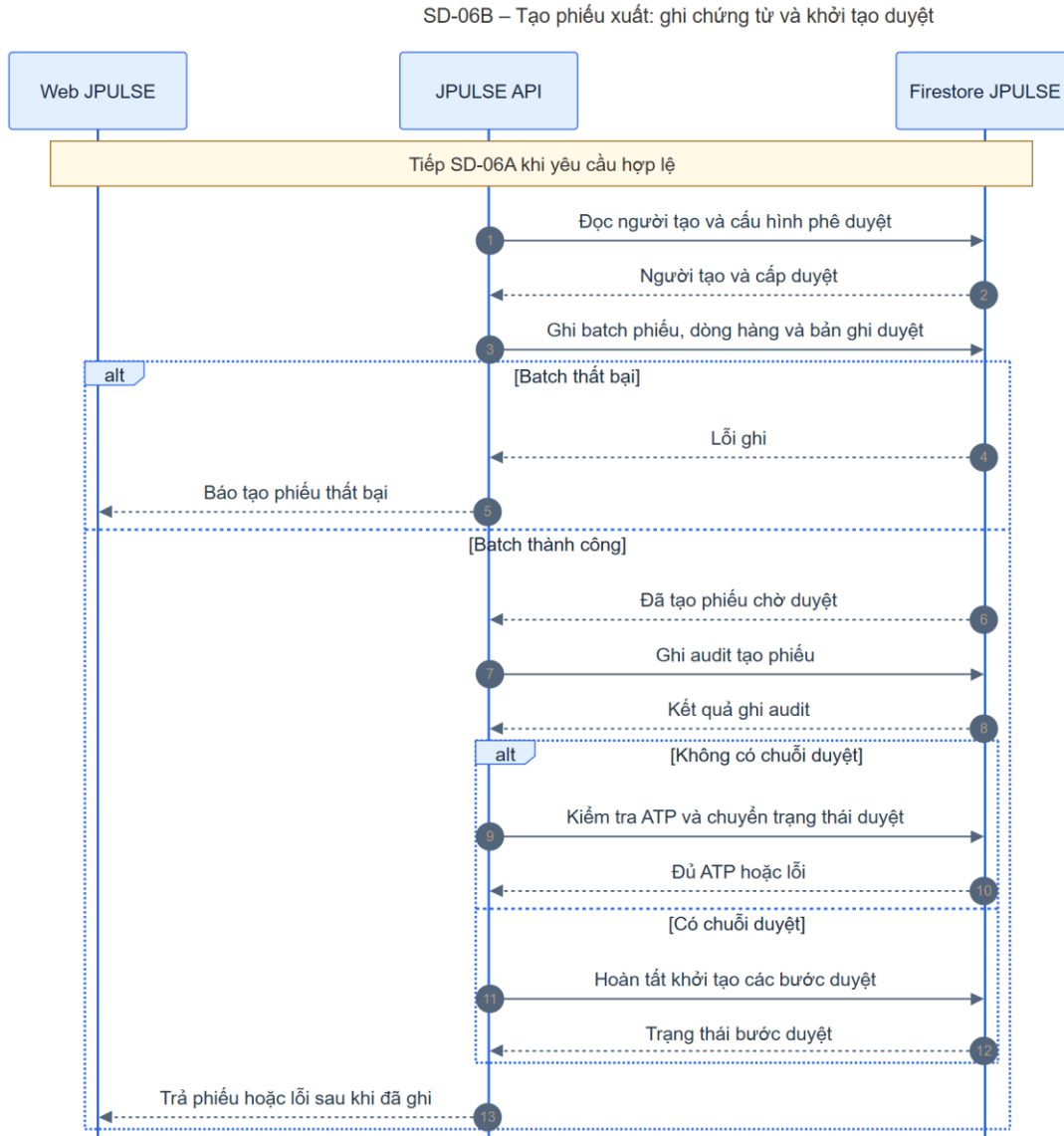
Hình 4-11: SD-06B ghi phiếu xuất và khởi tạo duyệt
