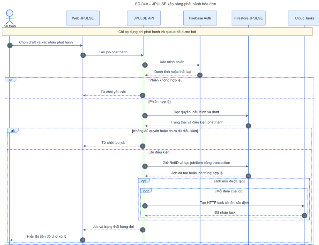
Hình 4-27: SD-04A tiếp nhận và xếp hàng phát hành hóa đơn
