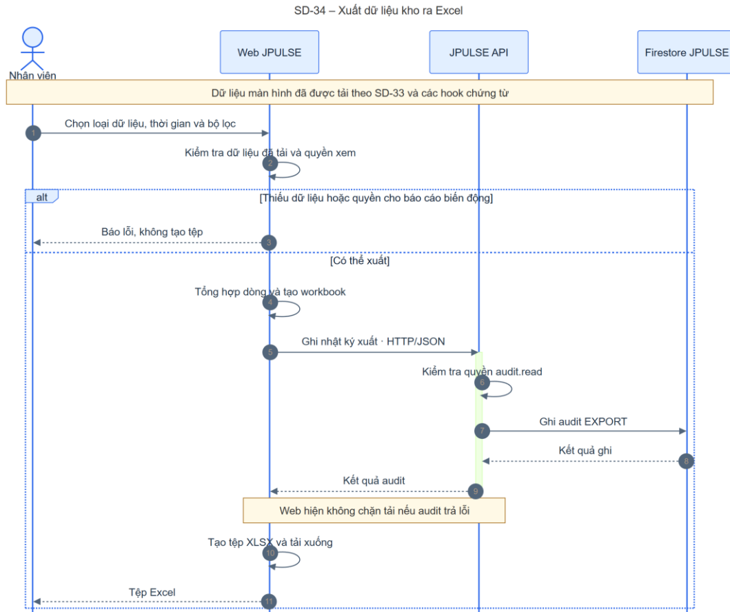
Hình 4-66: SD-34 xuất dữ liệu kho ra Excel
