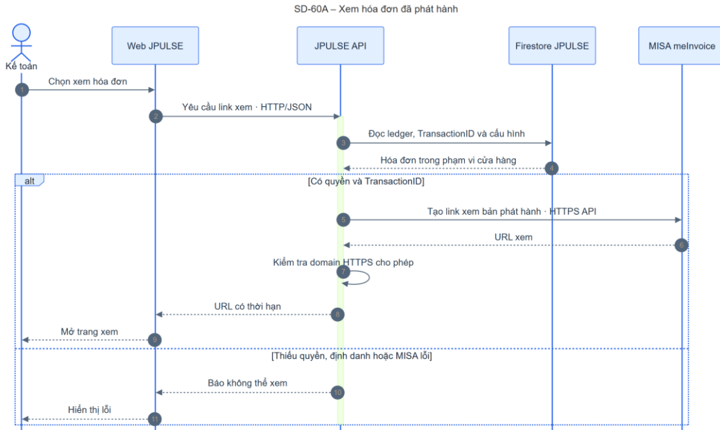
Hình 4-47: SD-60A xem hóa đơn đã phát hành
