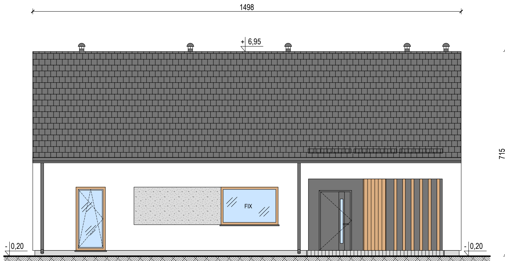
ELEWACJA WSCHODNIA, FRONTOWA
