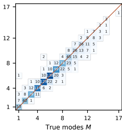
RoPE-TOA+Bias
